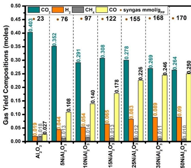
Fig. 4 Composition du gaz produit lors de la pyrolyse et du reformage à sec du polypropylène sur des catalyseurs au x\text{NiAl}_2\text{O}_3
