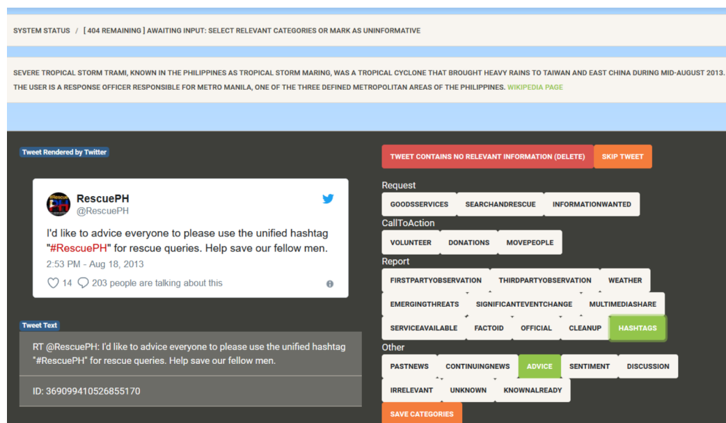
FIGURE 5.3 – Interface d'évaluation de TREC-IS (McCreadie et al. , 2019)
