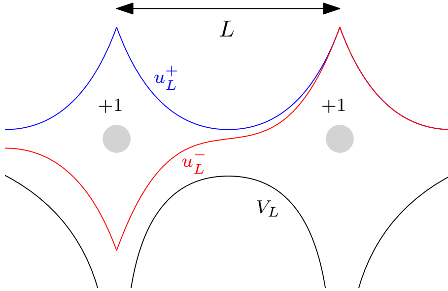
FIGURE 1.3 – Le double puits de potentiels. Les deux noyaux de charge +1 sont représentés par des disques colorés en gris et le potentiel V_L qu'ils génèrent est représenté par la courbe noire. La première fonction propre u_L^+ (resp. la seconde fonction propre u_L^- ) de h_L , représentée par la courbe bleue (resp. la courbe rouge), est approchée par une superposition paire (resp. impaire) de la première fonction propre de l'opérateur mono-atomique h .
