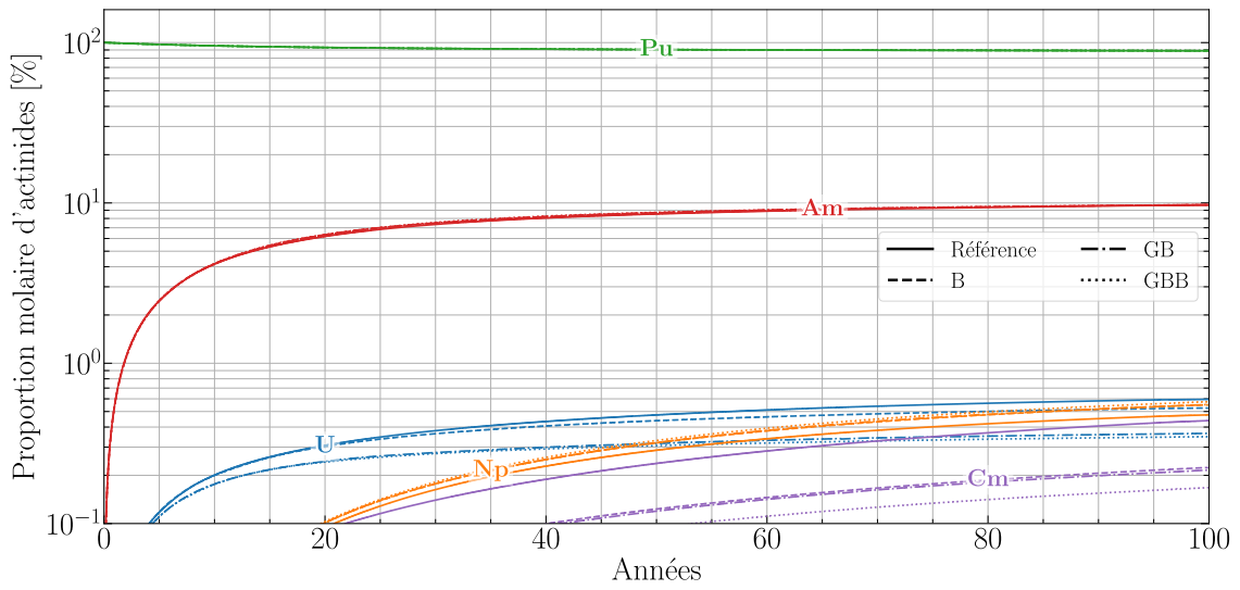
FIGURE 5.8 – Répartition molaire des actinides par éléments pour les configurations à 38.5% \text{Pu}_{\text{UOX}} avec comparaison au cas de référence
