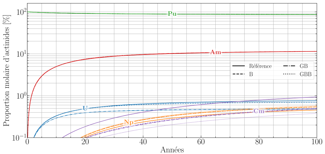
FIGURE 5.9 – Répartition molaire des actinides par éléments pour les configurations à 38.5% \text{Pu}_{\text{MIX}} avec comparaison au cas de référence
