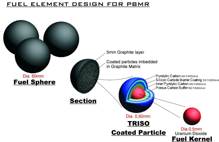
FIGURE 1.17 – Coupe d'un boulet de combustible (TRISO) d'un réacteur HTR (type PBMR)[47]
