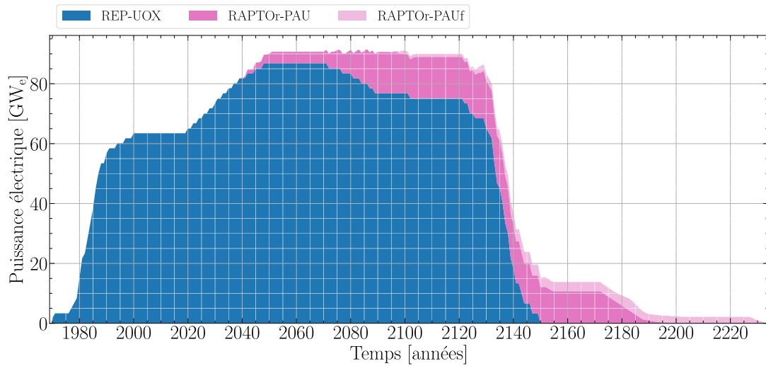
FIGURE 7.12 – Répartition de la puissance produite dans le parc lors du déploiement des RAPTOi-PAU et PAUf
