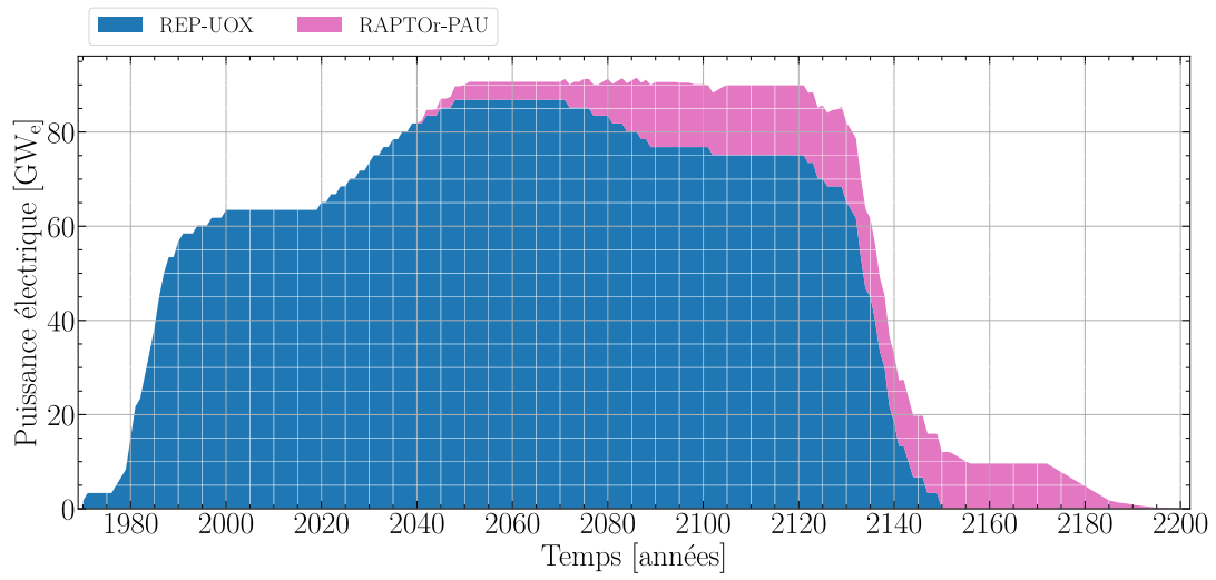
FIGURE 7.11 – Répartition de la puissance produite dans le parc lors du déploiement des RAPTOi-PAU
