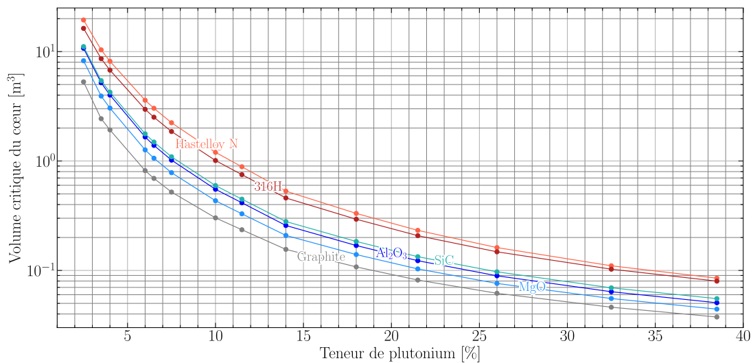
FIGURE 4.7 – Évolution du volume critique selon le matériau du réflecteur radial (aciers en rouge, céramiques en bleu et graphite en gris) pour un vecteur plutonium ex-UOX
