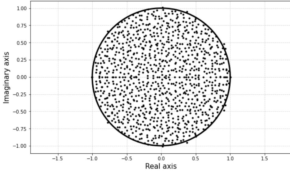
Figure 4: Spectre de la matrice aléatoire non-Hermitienne Y_n/\sqrt{n} dans le plan complexe ( n = 1000 , \sigma = 1 ). Le cercle de ligne continue représente la frontière de la loi circulaire.
