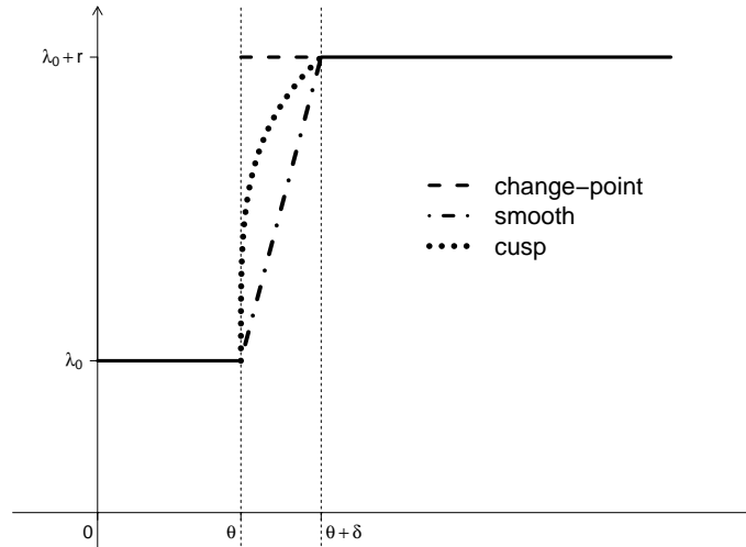
FIGURE 1 – Les cas de rupture, lisse et cusp (avec \varkappa = 1/4 )
