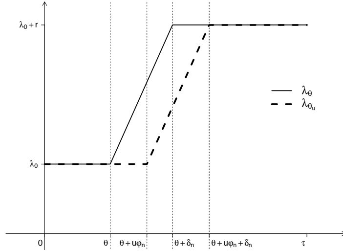
FIGURE 3 – \lambda_\theta et \lambda_{\theta_u} dans le cas u\varphi_n < \delta_n
