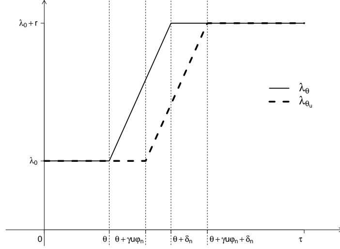
FIGURE 5 – \lambda_\theta et \lambda_{\theta_u} avec u, r > 0 et n \gg 1 (cas lent)
