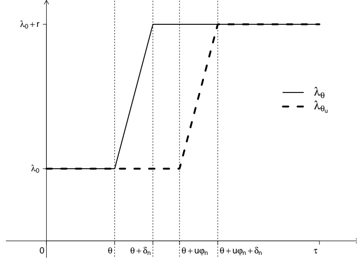
FIGURE 6 – \lambda_\theta et \lambda_{\theta_u} avec u, r > 0 et n \gg 1 (cas rapide)
