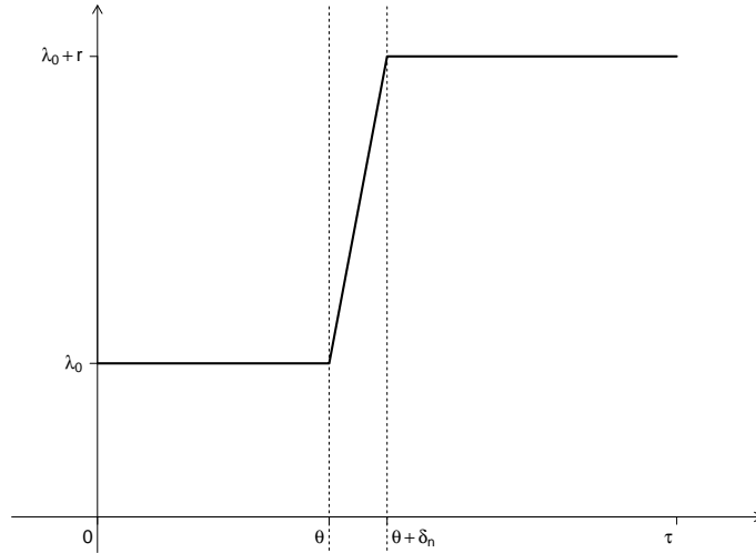
FIGURE 2 – fonction d'intensité \lambda_\theta^{(n)} , avec \psi \equiv \lambda_0
