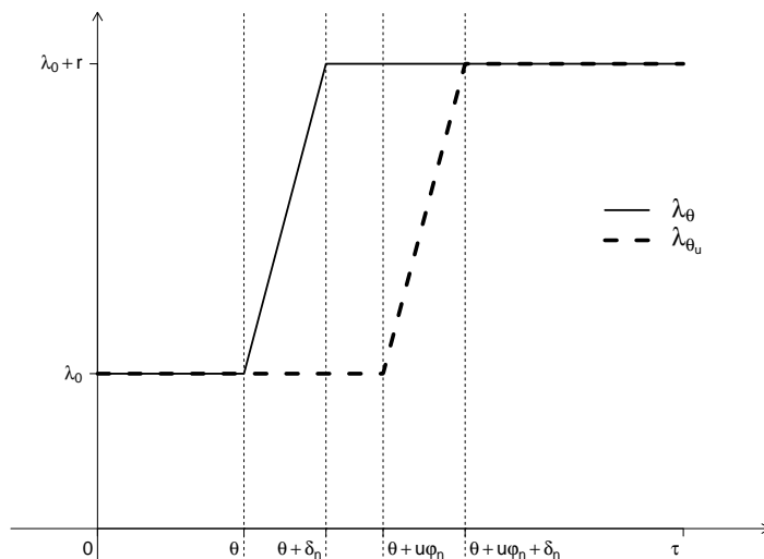
FIGURE 4 – \lambda_\theta et \lambda_{\theta_u} dans le cas \delta_n < u\varphi_n
