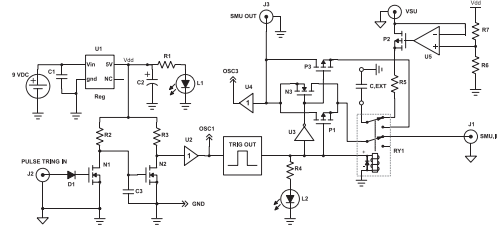
(d) Full schematic
