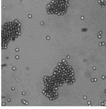
Figure 2: Formation de clusters denses de particule Janus à moitié recouverte de carbone évoluant dans un mélange quasi-critique d'eau et de lutidine [19].
