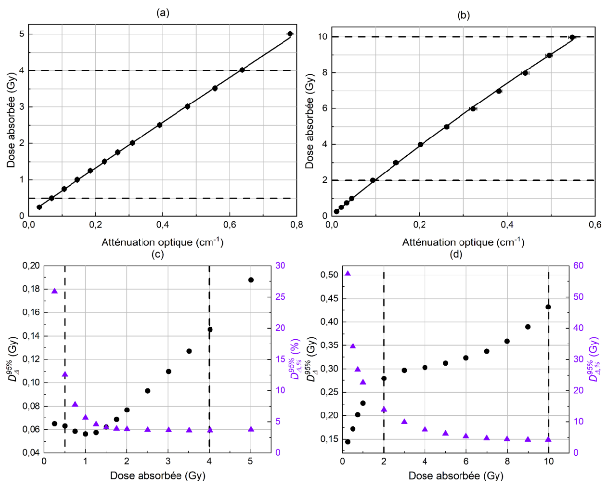
Figure 2.17 : Réponses en dose polynomiales du gel FXG (a) sur la gamme de dose [0,25 ; 5] Gy pour la lecture optique à 590 nm et (b) sur la gamme de dose [0,25 ; 10] Gy pour la lecture optique à 633 nm. Résolution en dose (cercles en noir) et résolution en dose relative (triangles en violet) à 590 nm (c) et 633 nm (d). Les lignes en pointillé dans les quatre graphes délimitent la gamme de dose absorbée pour laquelle la réponse en dose du gel FXG est linéaire.
