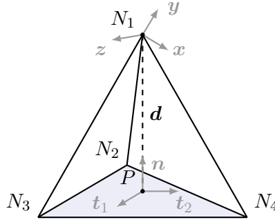
FIGURE 7.1 – Exemple d'un élément de contact 3D de typologie nœuds/faces connectant le nœud N_1 aux 3 autres nœuds N_2, N_3 et N_4 formant la surface en regard
