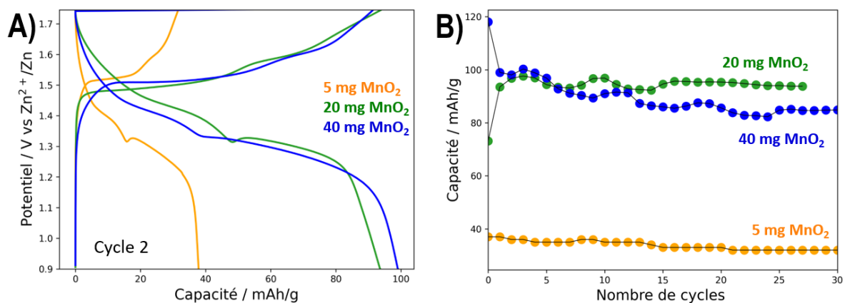
Figure V-10 : A) Profils de charge/décharge galvanostatiques à un courant de \pm 0,05 \text{ A/g}_{\text{MnO}_2} de cellules EMD-MnO 2 /Zn contenant 40, 20 ou 5 mg de MnO 2 (pourcentage massique de carbone C_{\text{sp}} maintenu à 20%) dans 100 µL 2M ZnSO 4 . B) Performance de cyclage des cellules montrées en A
