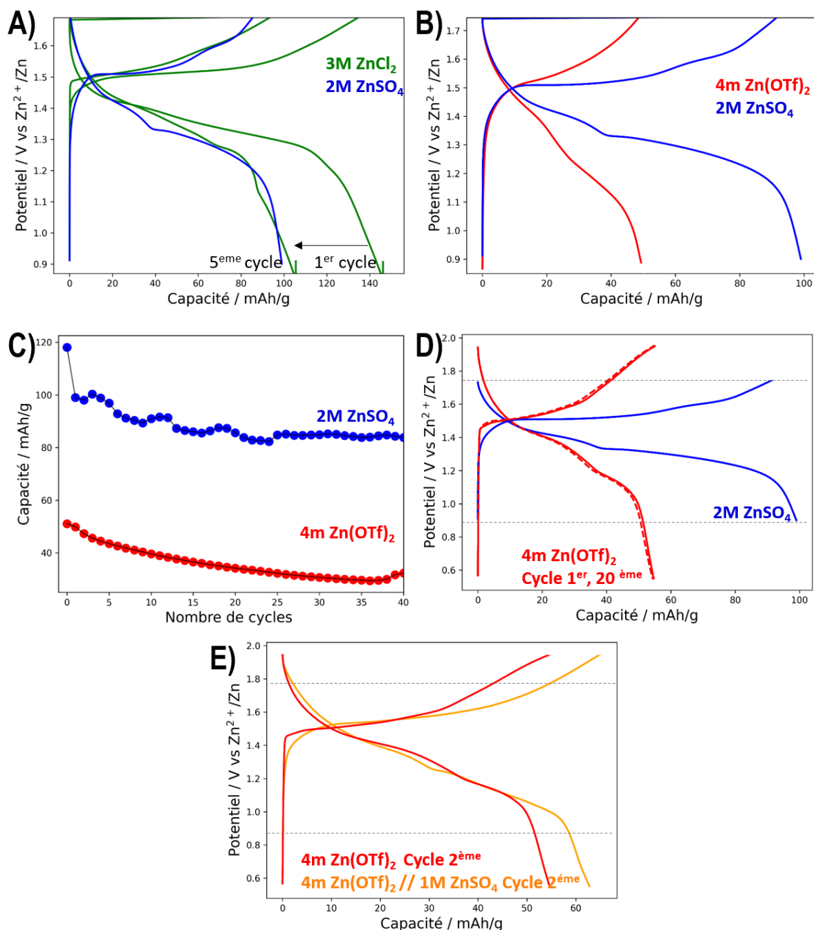
Figure V-11 : A) Profils de charge/décharge galvanostatiques à un courant de \pm 0,05 A/g MnO 2 de cellules EMD-MnO 2 /Zn contenant 20 mg de MnO 2 et 5 mg de C sp dans 100 μL de 2 M ZnSO 4 ou 3 M ZnCl 2 . B) Profils de charge/décharge galvanostatiques à un courant de \pm 0,05 A/g MnO 2 de cellules EMD-MnO 2 /Zn contenant 20 mg de MnO 2 et 5 mg de C sp dans 100 μL de 2 M ZnSO 4 ou 4 m Zn(OTf) 2 . C) Performance de cyclage des cellules montrées dans la Figure 11B. D) Profils de charge/décharge galvanostatiques de la cellule présentée dans la Figure
