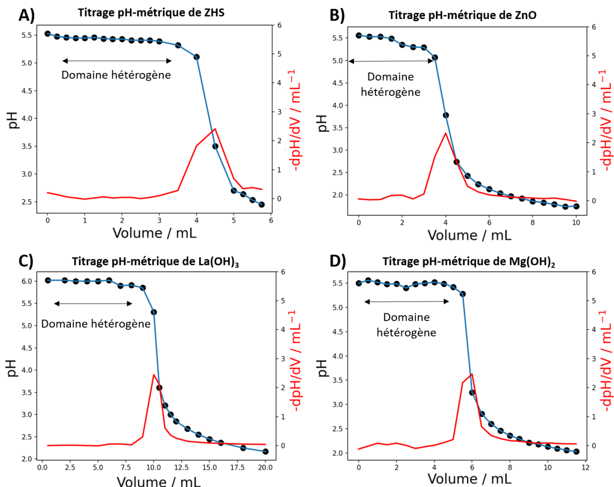
Figure V-3: A) Courbe du titrage pH-métrique d'une dispersion de 40 mg de Zn_4(OH)_6SO_4 \cdot 5H_2O dans 10 mL de 2 M ZnSO_4 . B) Courbe du titrage pH-métrique d'une dispersion de 20 mg de ZnO dans 10 mL de 2 M ZnSO_4 . C) Courbe du titrage pH-métrique d'une dispersion de 80 mg de La(OH)_3 dans 25 mL de 2 M ZnSO_4 . D) Courbe du titrage pH-métrique d'une dispersion de 20 mg de Mg(OH)_2 dans 10 mL de 2 M ZnSO_4
