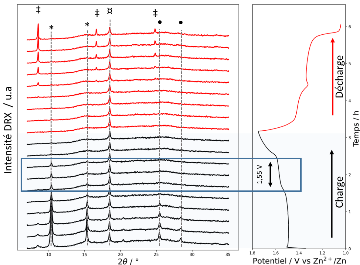
Figure III-4 : Profil de tension (charge et de décharge) à 10 \mu\text{A} et son suivi DRX in situ d'une cellule ZHS- \text{C}_{\text{sp}} /Zn dans un électrolyte 2 \text{ M ZnSO}_4 + 0,2 \text{ M MnSO}_4 . Attributions : (●) \text{ZnSO}_4 \cdot 3\text{Zn(OH)}_2 \cdot \text{H}_2\text{O} , (PDF 00-039-0690), (*) \text{ZnSO}_4 \cdot 3\text{Zn(OH)}_2 \cdot 4\text{H}_2\text{O} , (PDF 00-044-0673), (‡) \text{ZnSO}_4 \cdot 3\text{Zn(OH)}_2 \cdot 5\text{H}_2\text{O} , (PDF 00-039-0688), (⌘) Poly(fluorure de vinylidène), PDF 00-057-1927). Le ZHS a été synthétisé selon le protocole Moezzi et al. 164
