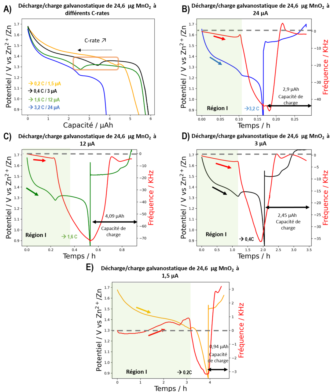
Figure IV-8 : A) Profils de décharge galvanostatique à -1,5 \mu\text{A} (courbe orange), -3 \mu\text{A} (courbe noire), -12 \mu\text{A} (courbe verte) et -24 \mu\text{A} (courbe bleu) correspondant à 0,2 C, 0,4 C, 1,6 C et 3,2 C respectivement dans un électrolyte de 4 mL de 2 M \text{ZnSO}_4 + 0,2 \text{ M MnSO}_4 enregistré sur un électrode QCM en or recouvert de \text{C}_{\text{sp}}\text{-PVDF} sur lequel a été déposé 24,6 \mu\text{g} de \text{MnO}_2 . Le C-rate a été calculés en suivant l'équation : C = I/Q_c où I correspond au courant appliqué (en \mu\text{A} ) et Q_c à la capacité (en \mu\text{Ah} ) utilisée pour électrodéposer 24,6 \mu\text{g} de \text{MnO}_2 . B) Décharge/charge galvanostatique (ligne bleue) et variation de fréquence (courbe rouge) d'une cellule de 24,6 \mu\text{g MnO}_2 à \pm 24 \mu\text{A} / 3,2 \text{ C} . C) Décharge/charge galvanostatique (ligne verte) et variation de fréquence (courbe rouge) d'une cellule de 24,6 \mu\text{g MnO}_2 à \pm 12 \mu\text{A} / 1,6 \text{ C} . D) Décharge/charge galvanostatique (ligne noire) et variation de fréquence (courbe rouge) d'une cellule de 24,6 \mu\text{g MnO}_2 à \pm 3 \mu\text{A} / 0,4 \text{ C} . E) Décharge/charge galvanostatique (ligne orange) et variation de fréquence (courbe rouge) d'une cellule de 24,6 \mu\text{g MnO}_2 à \pm 1,5 \mu\text{A} / 0,2 \text{ C}
