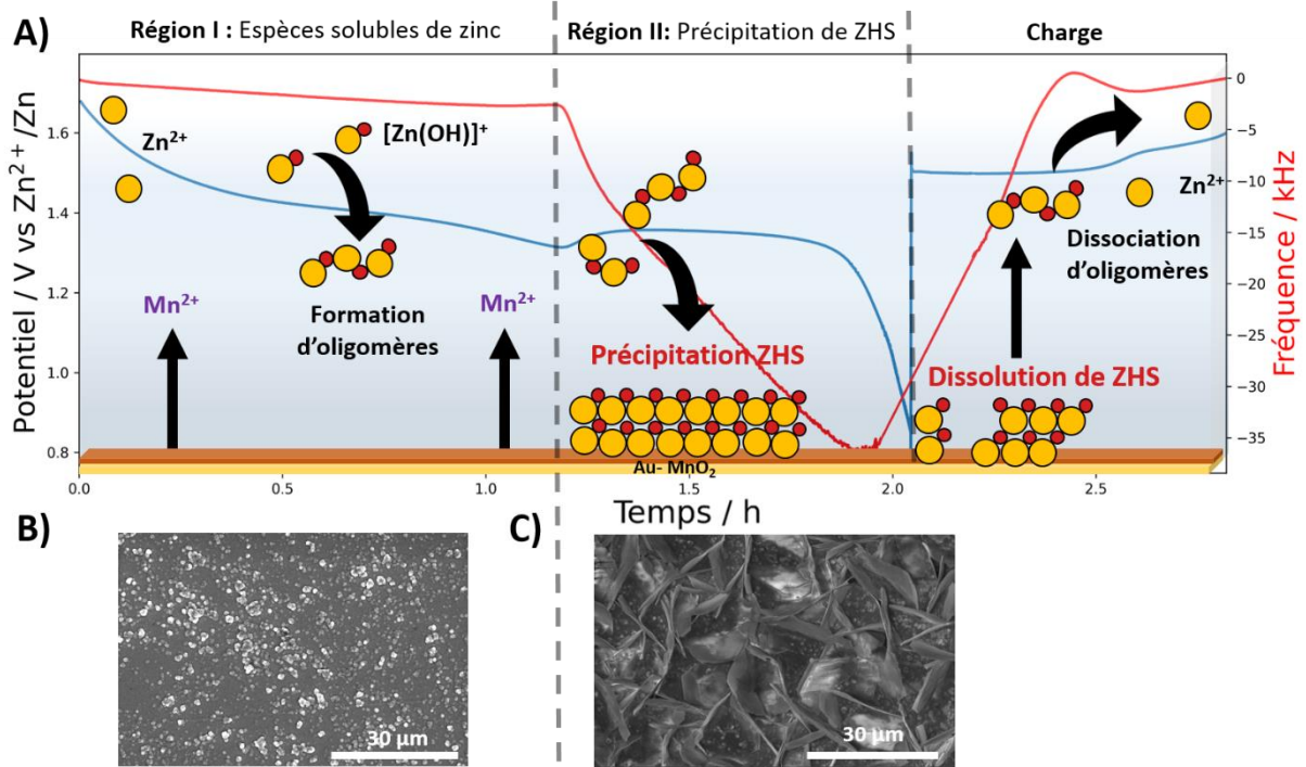
Figure IV-6 : A) Profil de décharge/charge galvanostatique à \pm 3 \mu\text{A} enregistré sur un électrode QCM en or recouvert de carbone sur lequel 24,6 \mu\text{g} de \text{MnO}_2 a été électrodéposé (ligne bleue) et variation de fréquence correspondante (ligne rouge) dans de 2 \text{ M ZnSO}_4 + 0,2 \text{ M MnSO}_4 (avec un schéma du processus chimique). B-C) Images MEB des électrodes à différents états de décharge (avant et après le pic de nucléation) dans des conditions identiques à A
