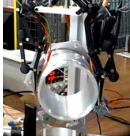
FIGURE 7.24 – Scénario 2 : Résultats expérimentaux de la préhension prismatique avec une référence de force=15 N.
