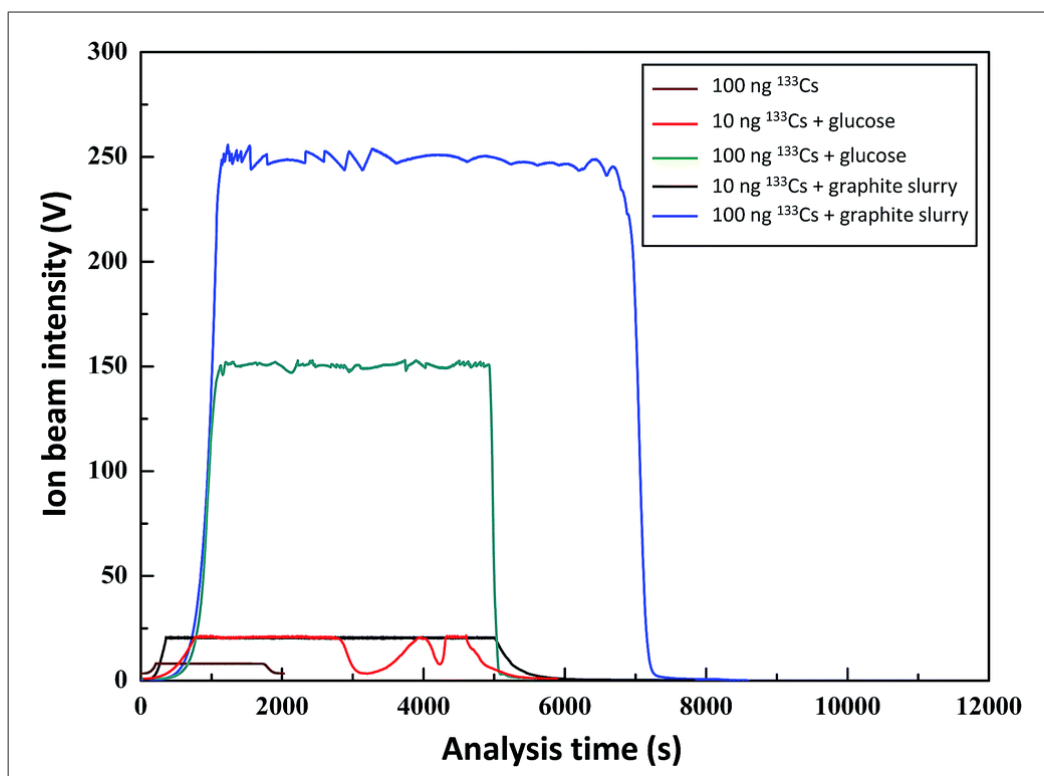
Figure I.IV-13 : Comparaison de l'intensité et de la stabilité du faisceau d'ion en fonction de la teneur en ^{133}\text{Cs} et des activateurs ajoutés. (Source : Bu et al. 2019)
