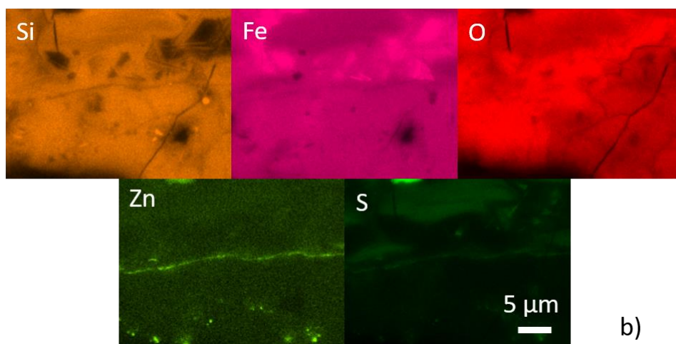
Figure 4-26 : Micrographie MEB rétrodiffusée dans le liseré séparant les PCs internes des PCs externes (a), et cartographies EDS associées (b) (distance = 0,390 mm).
