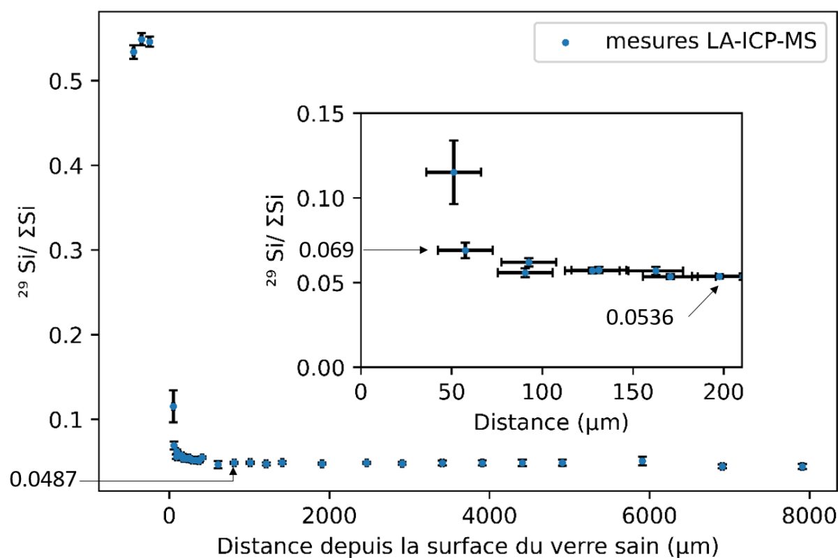
Figure 4-61 : Profil du ^{29}\text{Si} dans l'argilite à partir de la surface du verre sain, déterminée par AL-ICP-MS (distance = 6,1 mm). L'encadré est le graphique zoomé entre 0 et 200 µm de distance de la surface du verre sain. Spot d'analyse de 30 µm.
