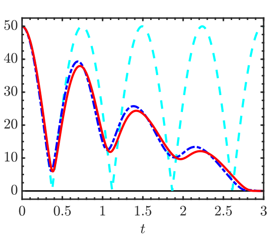
Figure 2: c_g = 1 – (—) \|y^*(\cdot, t)\|_{L^2(\Omega)} ; (---) \|y_0(\cdot, t)\|_{L^2(\Omega)} ; (—) \|y(\cdot, t; 0)\|_{L^2(\Omega)} .
