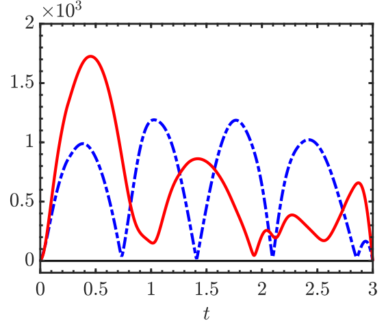
Figure 5: c_g = 5 – (—) \|f^*(\cdot, t)\|_{L^2_x(\omega)} ; (---) \|f_0(\cdot, t)\|_{L^2_x(\omega)} .
