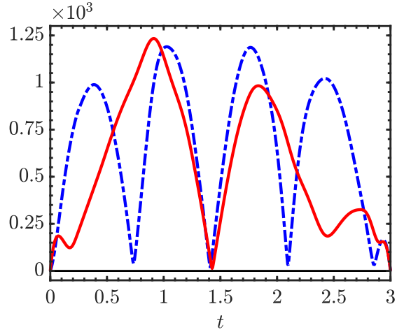
Figure 7: c_g = 10 – (—) \|f^*(\cdot, t)\|_{L^2_x(\omega)} ; (---) \|f_0(\cdot, t)\|_{L^2_x(\omega)} .
