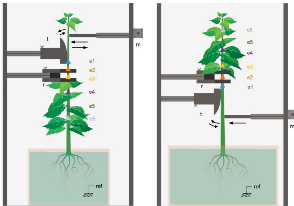
Figure 24 : Dispositifs expérimentaux pour mesurer la réponse électrique dans la tige après une flexion apicale (A) ou basale (B) transitoire. Le peuplier est placé dans une cage de Faraday, fixé en deux points de la tige par des anneaux de serrage (r). Le système racinaire baigne dans une solution nutritive. La tige est fléchie à une vitesse de 2.5 \text{ cm}\cdot\text{s}^{-1} avec un bras motorisé (m) qui pousse la tige le long d'un gabarit en plastique de courbure constante (t). Les électrodes sont placées dans la partie immobile de la tige. L'électrode e1 est insérée 2 cm en dessous du contact tige-gabarit. Les distances sont alors : e1-e2 = 2 cm, e2-e3 = 3 cm, e3-e4 = 5 cm, e4-e5 = 5 cm and e5-e6 = 5 cm. La différence de potentiel est mesurée le long de 20 cm de tige droite, en dessous (A) ou au-dessus (B) de la région courbée.
