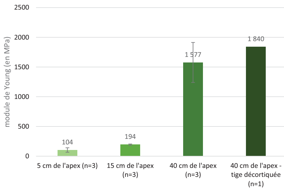
Figure 57 : Modules de Young mesurés pour différentes sections de tige de peupliers ( Populus tremula x alba ). Les peupliers sont cultivés en hydroponie et âgés de 5 mois. Le module de Young a été mesuré à 5 cm de l'apex, 15 cm de l'apex et 40 cm de l'apex (zone sollicitée lors de la flexion apicale standard) décortiqué ou non. La décortication retire les tissus de l'épiderme jusqu'à l'assise cambiale, ne laissant que le xylème et la moelle.
