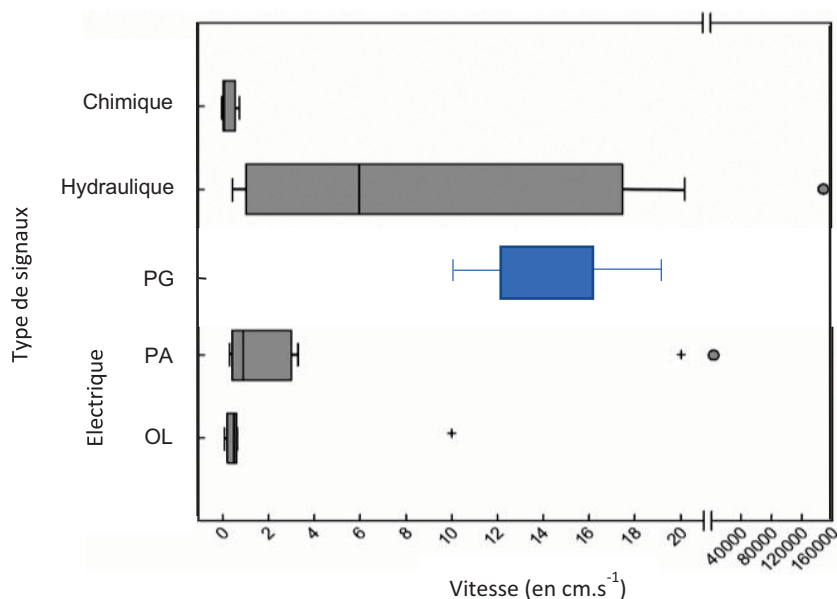
Figure 45 : Gammes de vitesse de propagation (et erreurs standards) des différents types de signaux chez les plantes, signaux chimiques, hydrauliques, le potentiel 'graduel' (PG) et électriques (potentiels d'action et onde lente). La vitesse du PG correspond à la vitesse de propagation
