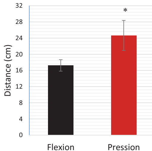
Figure 44 : Distance maximale théorique de propagation de l'onde de dépolarisation dans la tige de peuplier suite à la mise sous pression du système racinaire. '*' désigne une différence significative par rapport à la flexion (IC à 95%, Cf. Mat&Met Chapitre 1). (Pression, N=10 ; Flexion, N=40).
