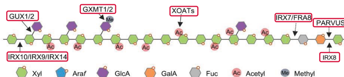
Figure 51 : Représentation de la biosynthèse des xylanes (hémicellulose) chez une dicotylédone. D'après Zhang et al. , (2021). Les gènes codant pour les enzymes encadrées en rouge sont identifiés et régulés négativement en A1 suite à la flexion de la tige de peuplier. IRX9, IRX10, IRX14 sont des xylosyltransférases et forment un complexe xylane synthase. Les GUX1-2 sont des glucuronyltransférases. Les GXMT sont des glucuronoxylane méthyltransférases. Les XOATs sont des acétyltransférases. FRA8, PARCUS et IRX8 sont impliquées dans la synthèse de la séquence terminale des xylanes.
