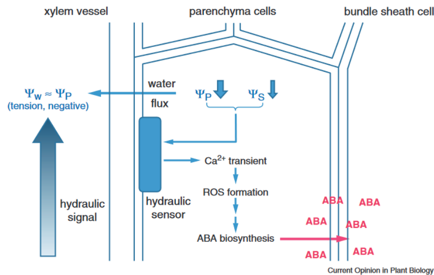
Figure 9 : Conversion d'un stress hydrique des racines en signal hydraulique perçu dans les parties aériennes de la plante via le xylème. D'après Christmann et al. , 2013.
