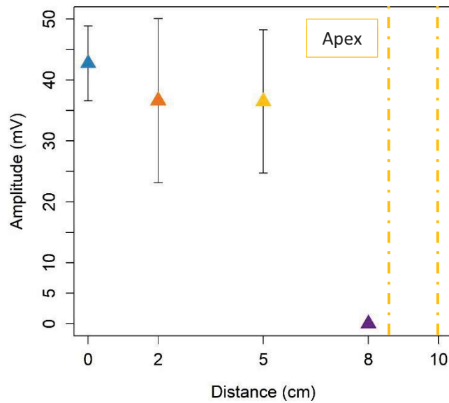
Figure 56 : Evolution du PG induit par une flexion de la tige de peuplier localisée à 10 cm de l'apex. La zone délimitée par les pointillés jaunes correspond à l'apex, échantillonné 30 minutes après la flexion de la tige pour l'analyse transcriptomique.
