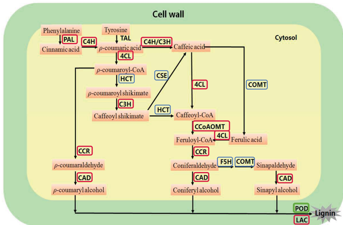
Figure 52 : La voie de biosynthèse de la lignine chez le peuplier et sa régulation en réponse à la flexion (en A1). D'après Zhang et al. , (2018). Les enzymes dont les gènes sont régulés négativement en réponse à la flexion sont encadrées en rouge. En vert sont encadrées les peroxydases (POD) pour la surexpression de l'une d'elle en réponse à la flexion. En bleu sont encadrées les enzymes dont les gènes ne sont pas régulés par la flexion. PAL, phenylalanine ammonia-lyase; TAL, tyrosine ammonia-lyase; C4H, cinnamate 4-hydroxylase; 4CL, 4-coumarate: CoA ligase; CCR, cinnamoyl-CoA reductase; HCT, hydroxycinnamoyl-CoA shikimate/Quinatehydroxycinnamoyltransferase; C3H, p-coumarate 3-hydroxylase; CCoAOMT, caffeoyl-CoA O-methyltransferase; F5H, ferulate 5-hydroxylase; CSE, caffeoyl shikimate esterase; COMT, caffeic acid O-methyltransferase; CAD, cinnamyl alcohol dehydrogenase; LAC, laccase.
