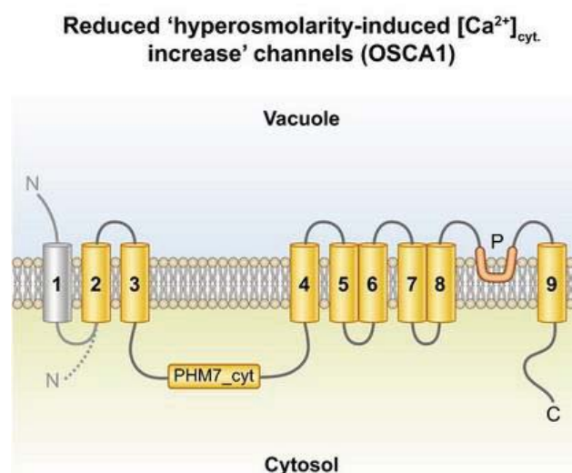
Figure 23 : Représentation de la topologie membranaire du canal OSCA1 (Reduced'hyperosmolarity-induces [Ca^{2+}]_{cyt} increase' channel 1). D'après Demidchik et al. , (2018).
