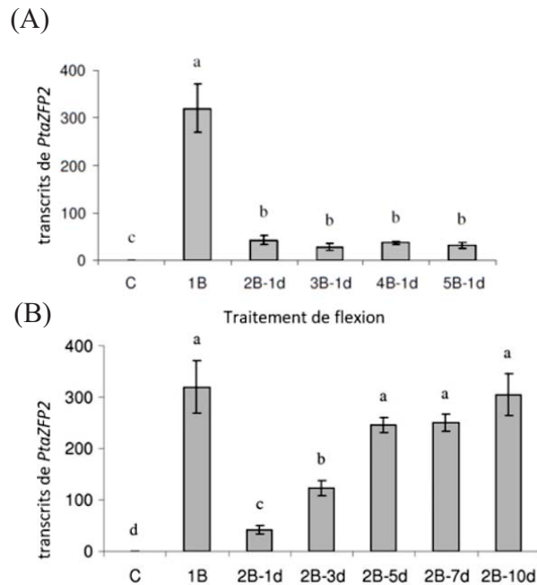
Figure 3 : Phénomène d'accommodation : effet des flexions répétées. (A) Accumulation des transcrits de PtaZFP2 en réponse à une ou plusieurs flexions successives de la tige séparées de 24h (1d). (B) Effet du délai entre deux flexions successives sur l'accumulation des transcrits de PtaZFP2 . C : plantes contrôles non fléchies, B : traitements de 1, 2, 3, 4, 5 flexions, d : délais de 1, 3, 5, 7 et 10 jours entre les deux flexions. D'après Martin et al. (2010).
