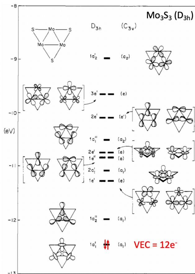
Figure 1.49 : Diagramme d'orbitales moléculaires du motif à cluster isolé \text{Mo}_3\text{S}_3 ( D_{3h} , VEC = 12) (adapté de [4]).
