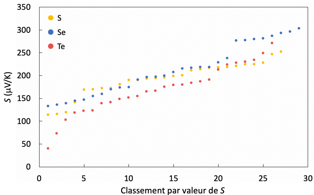
Figure 3.5 : Coefficients de Seebeck classés dans leur ordre croissant à T = 800 K et n_{\text{moy}} des 82 formules hypothétiques, triés selon chaque type de ligand (S en jaune, Se en bleu, Te en rouge).
