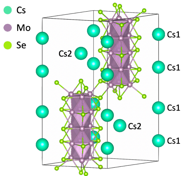
Figure 1.24: Structure cristalline du composé Cs 3 Mo 15 Se 17 ( P6 3 /m ) [34].
