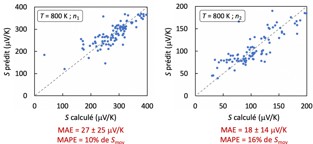
Figure 3.12 : Comparaison des coefficients de Seebeck calculés par DFT et prédits par Random Forest pour les quatre modèles prédictifs. La MAE, son écart-type et la MAPE sont indiqués.
