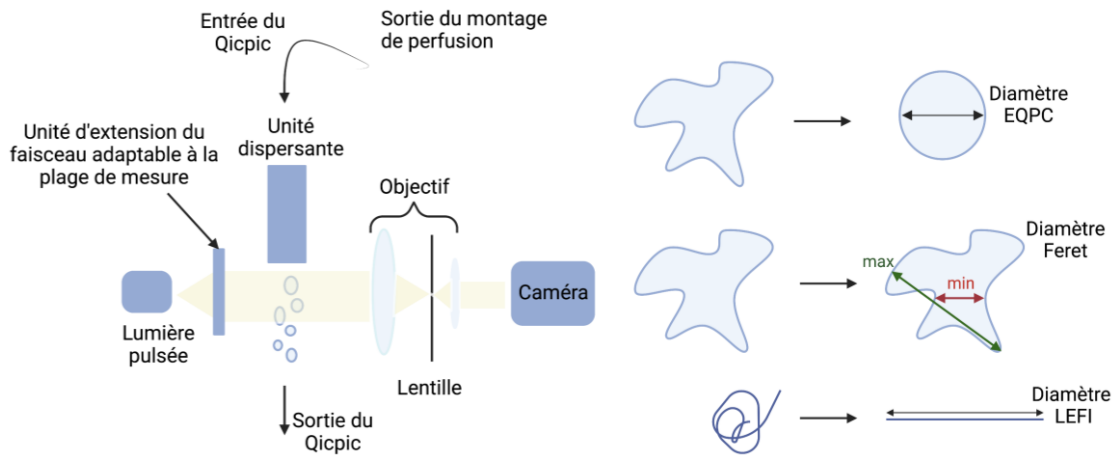
Figure 8. Schéma représentant le principe de fonctionnement du Qicpic® et les diamètres particuliers calculés par l'algorithme du logiciel Windox® relié au Qicpic, inspiré de (267)
