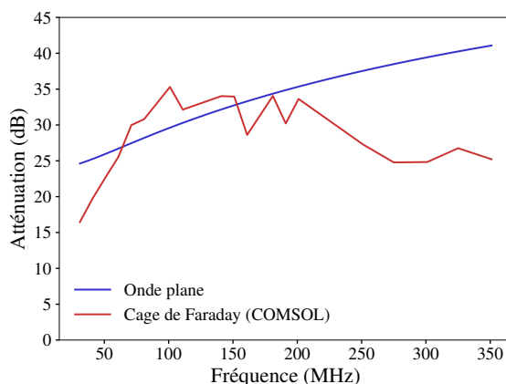
FIGURE 3.8 – Comparaison des atténuations obtenues avec la formule en onde plane et en cage de Faraday avec COMSOL sur un voile homogène
