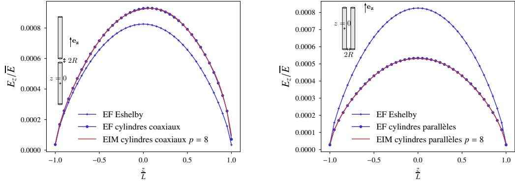
(a) Deux cylindres coaxiaux, d'élongement L/R = 50 , soumis à un champ électrique extérieur \bar{\mathbf{E}} = \bar{E} \mathbf{e}_z , pour un contraste \sigma_1/\sigma_0 = 10^6
