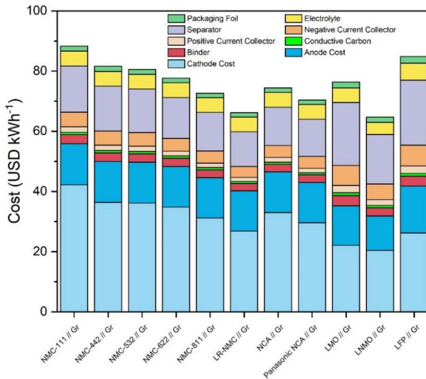
Figure 1-14 : Comparaison des coûts des matériaux les plus utilisés dans les cellules Li-ion [128].
