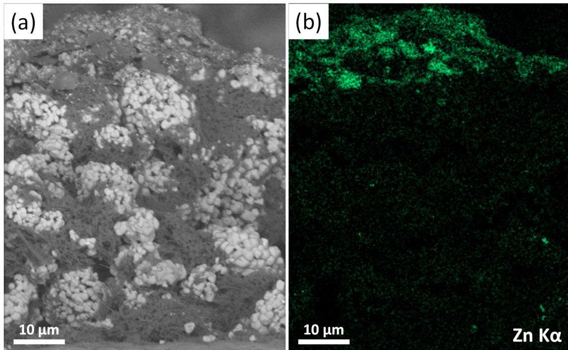
Figure 3-22 : Image MEB d'une coupe de l'électrode revêtue (a) et cartographie EDX du zinc associée (b).
