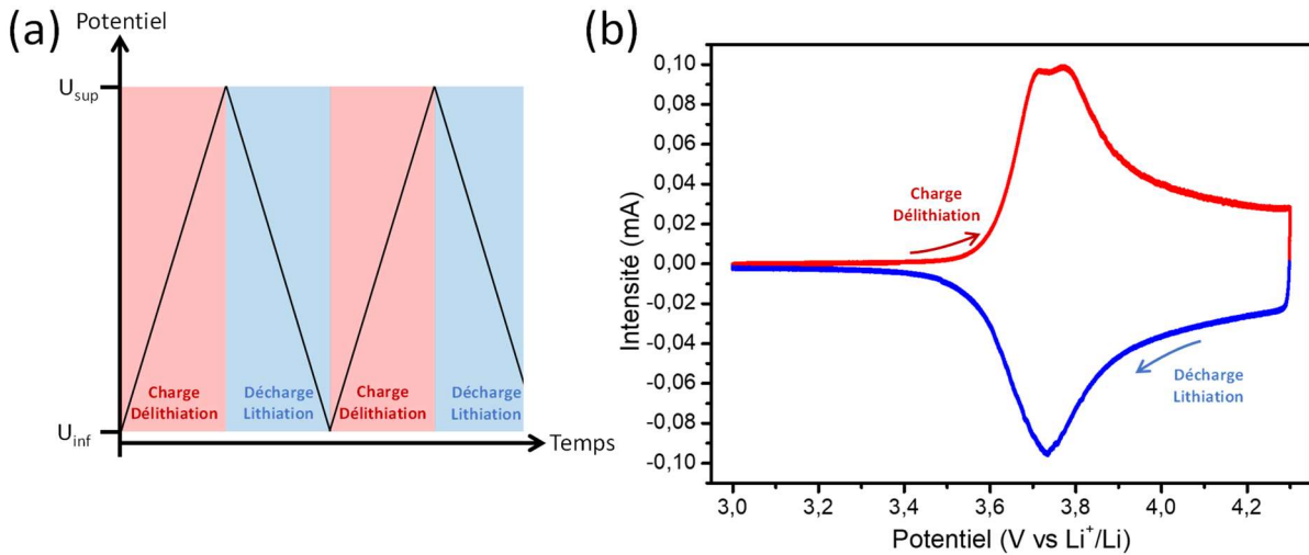
Figure 2-27 : (a) programme du potentiel appliqué en voltammétrie cyclique ; (b) Courbe de cyclage obtenue en voltammétrie cyclique en traçant l'intensité mesurée en fonction du potentiel.
