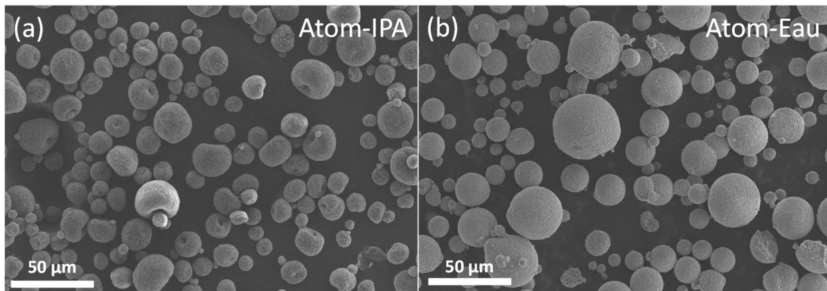
Figure 3-7 : Images MEB des particules secondaires obtenues après séchage dans l'isopropanol (a) et dans l'eau (b).
