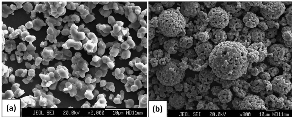
Figure 1-25 : Images MEB des poudres de NMC333 (a) par la méthode de réaction à l'état solide classique à 1 000°C, (b) par méthode de séchage par atomisation à 1000°C [208].
