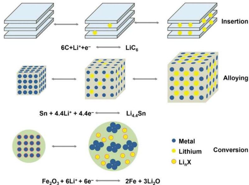
Figure 1-2 : Changements structuraux pendant la (dé)charge des matériaux d'insertion, d'alliage et de conversion [18]
