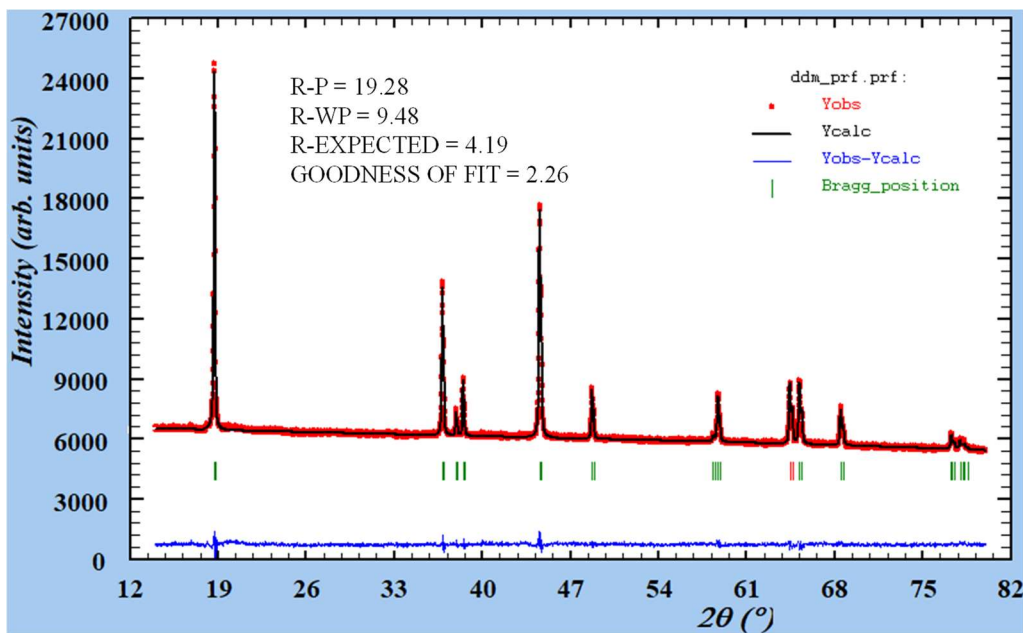
Figure 3-6 : Affinement du diffractogramme du NMC333 obtenu avec un broyage ultrafin.
