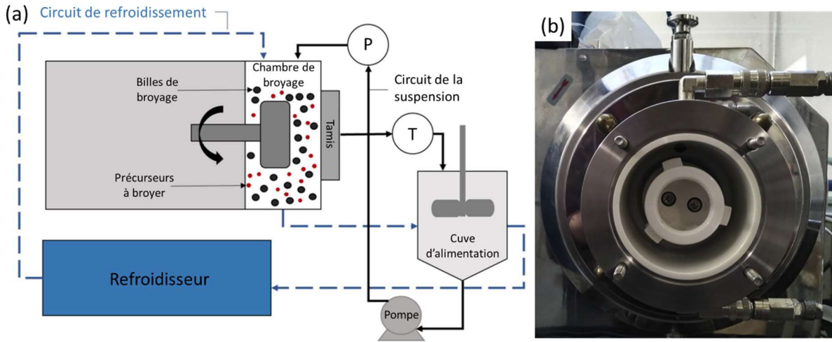
Figure 2-4 : (a) Schéma de fonctionnement de l'attriteur [250], P et T représentent le manomètre et le thermomètre respectivement ; (b) Photo de l'intérieur de la chambre de broyage en céramique [251].
