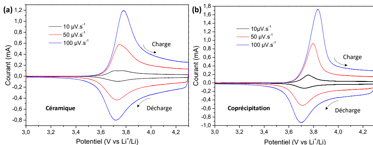
Figure 3-30 : Voltammétries cycliques à plusieurs vitesses de balayage entre 3 V et 4,3 V du matériau NMC333 synthétisé par voie céramique (a) et par coprécipitation (b).
