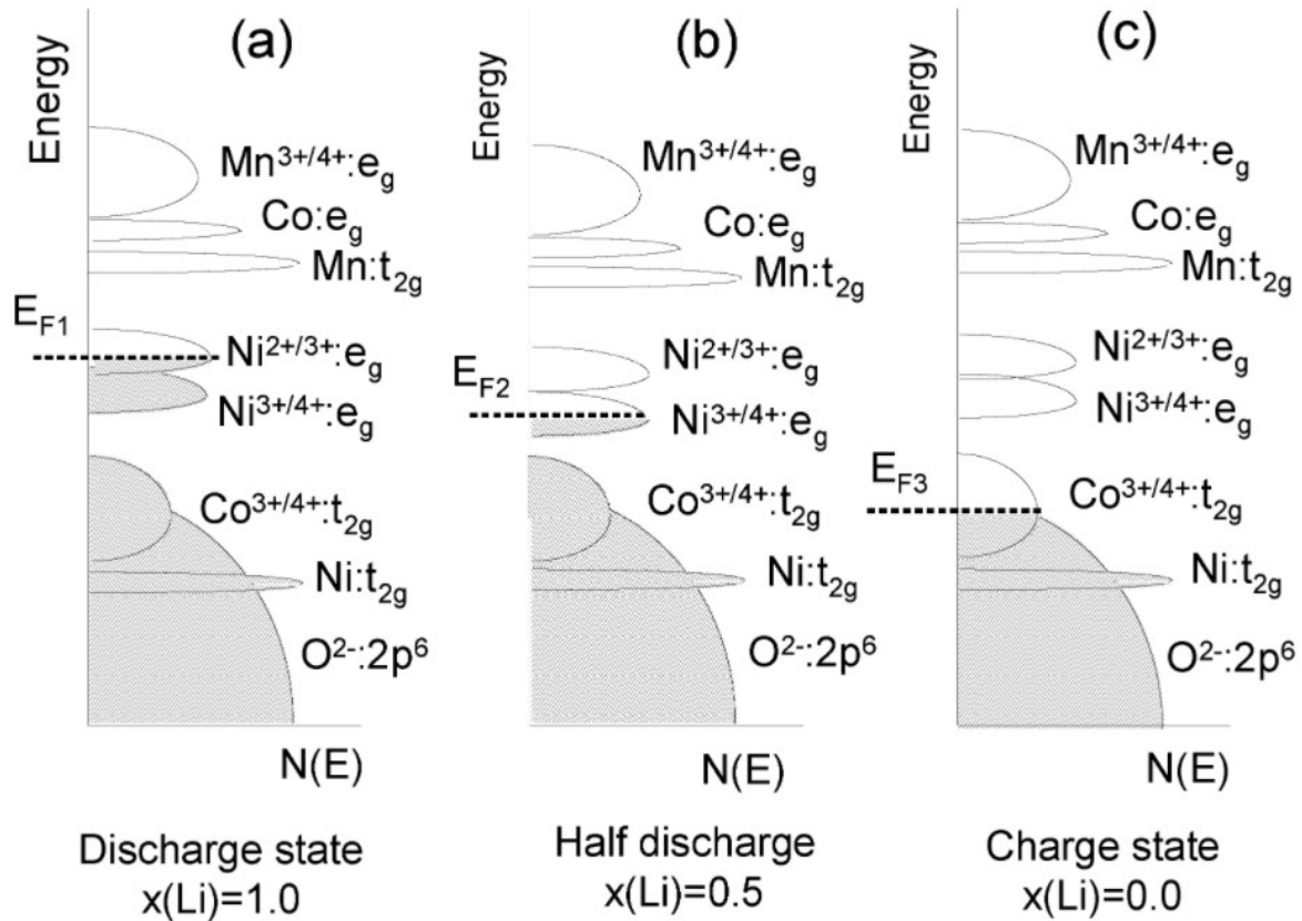
Figure 1-18 : Diagramme d'énergie en fonction de la densité d'état montrant les niveaux de Fermi relatifs des couples redox du composé \text{LiNi}_x\text{Co}_y\text{Mn}_{1-x-y}\text{O}_2 à trois états de charge du matériau : (a) état lithié/déchargé, (b) état intermédiaire et (c) état délithié/chargé [156]
