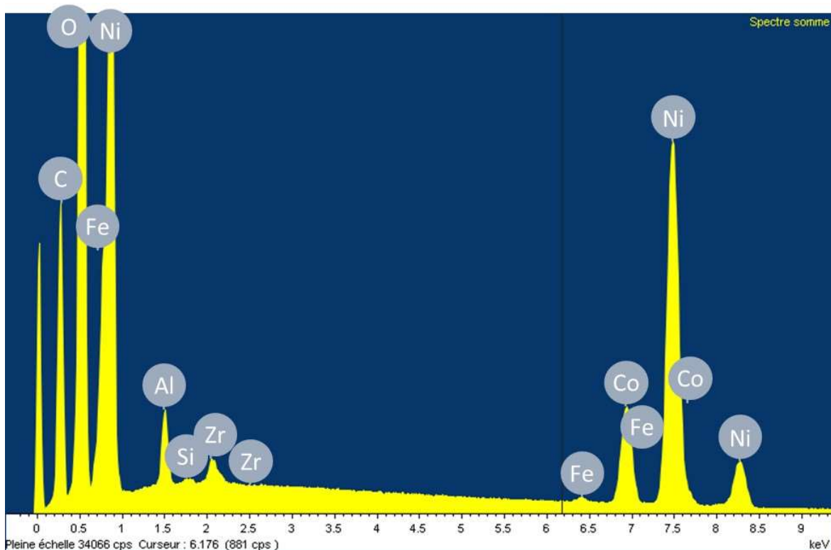
Figure 2-21 : Exemple d'une analyse par EDX obtenue sur une zone riche en nickel d'un mélange de précurseurs de NMC avant broyage.
