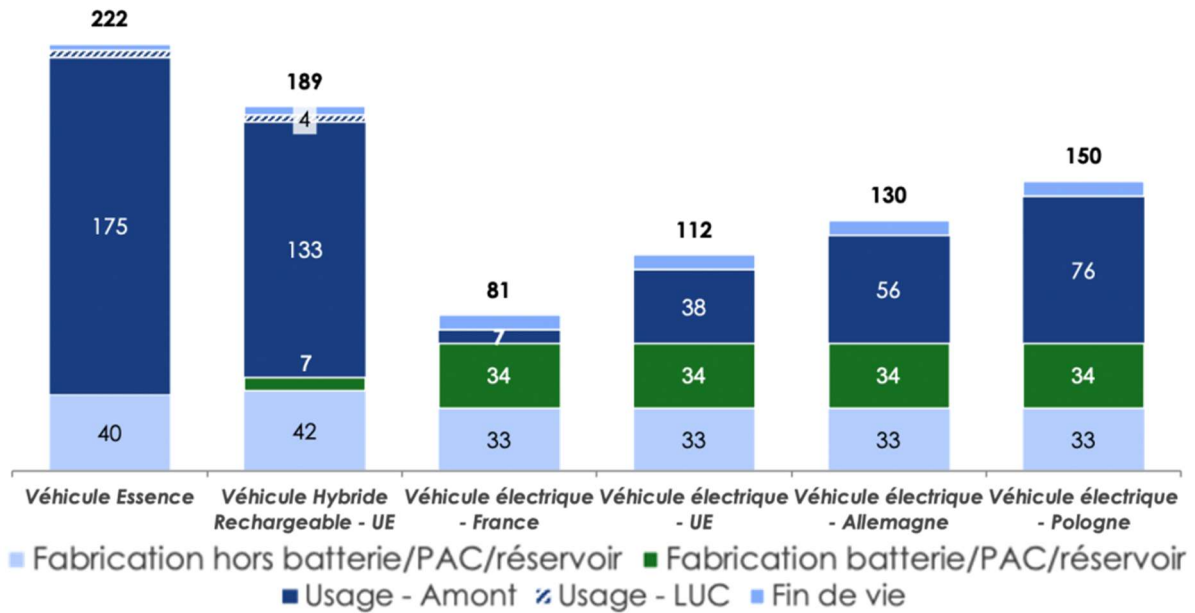
Figure 2 : Empreinte carbone moyenne (en gCO_2e/km ) sur la durée de vie d'un véhicule compact vendu en 2020 dans l'Union Européenne [6].
