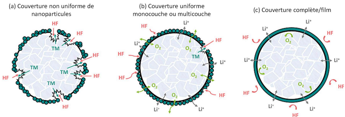
Figure 1-27 : Représentation schématique des morphologies de revêtement, de leur résistance potentielle à l'attaque de HF et des chemins de diffusion de Li^+ et O_2 possibles. [218].
