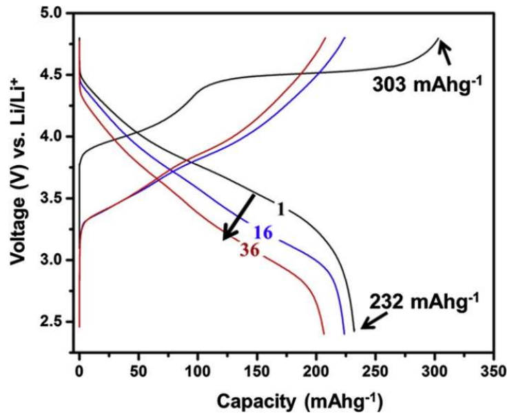
Figure 1-22 : Profils de charge/décharge d'une NMC enrichie en lithium [178].
