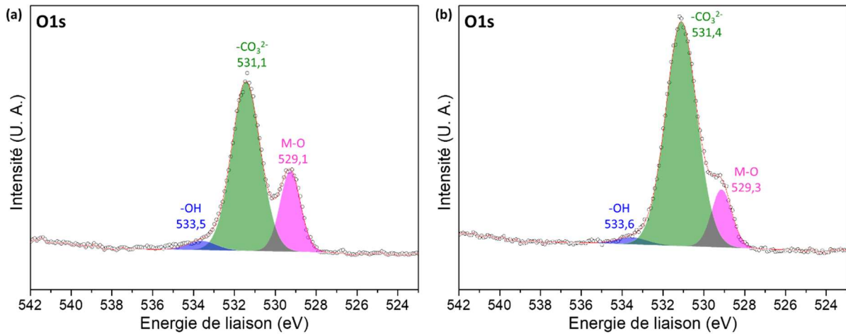
Figure 4-6 : Signal décomposé de la couche 1s de l'oxygène des spectres XPS (a) du matériau NMC622 de référence (coprécipitation) et (b) du matériau NMC622 synthétisée (voie solide).
