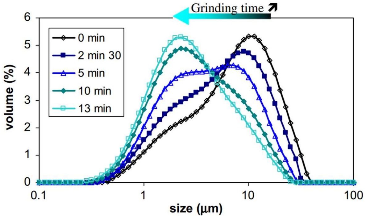
Figure 2-2 : Evolution bimodale de la distribution en taille des particules solides au cours du broyage [249].
