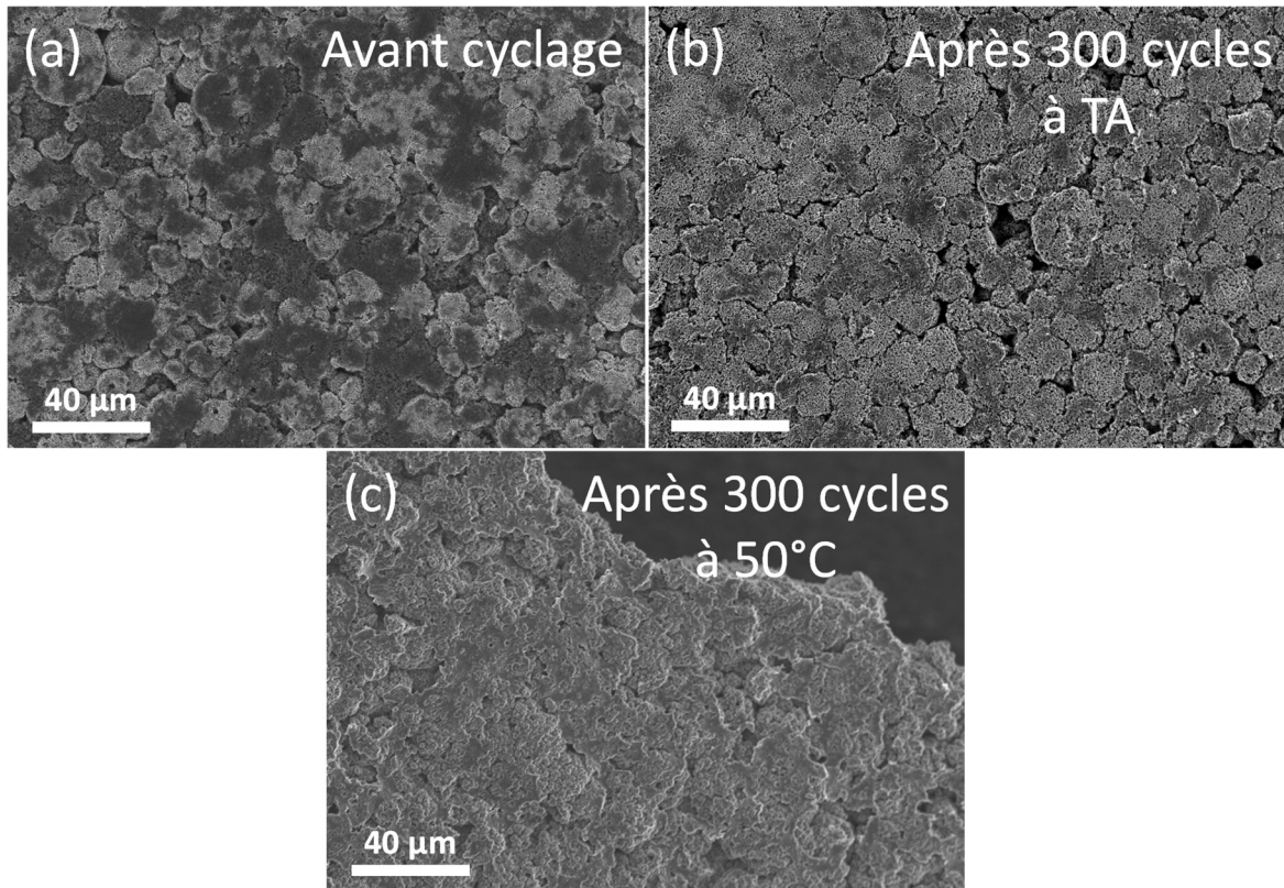
Figure 3-27 : Images MEB d'une électrode (a) avant cyclage, (b) après cyclage à température ambiante et (c) après cyclage à 50°C.
