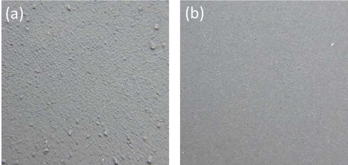
Figure 3-19 : Photos des électrodes enduites avec le matériau non-tamisé (a) et le matériau tamisé (b).
