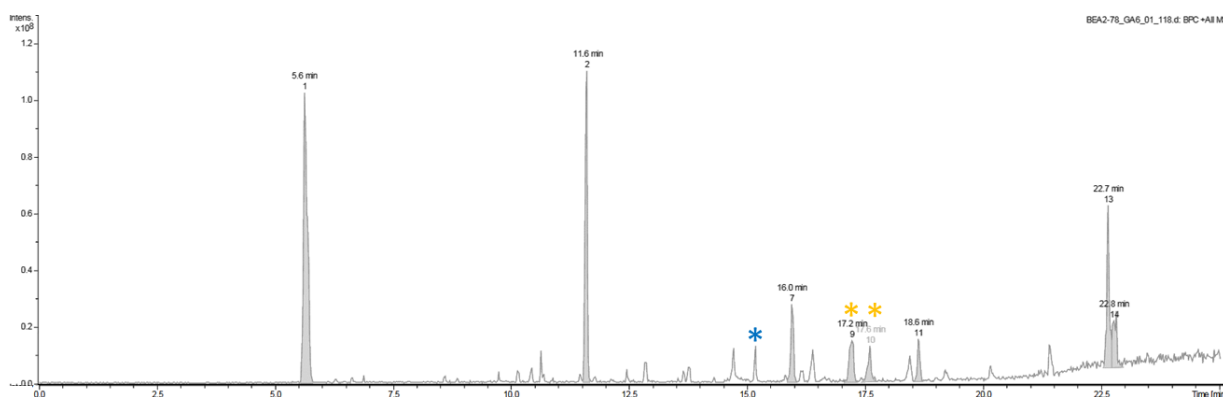
Figure 61 : chromatogramme de l'analyse LC-MS en mode ESI+ du mélange de produits obtenus à l'issue de l'application du plan de synthèse de la voie « Sonogashira sur un mélange de plusieurs éthers de propargyle (en bleu, produit formé avec la 4-propargyloxyanisole 7 ; en jaune, produits formés avec l'aurone propargylée 8 )
