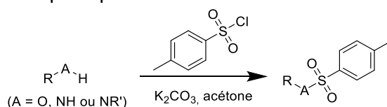
Schéma 20 : principe de formation de CEE par sulfonylation avec du chlorure de p -toluènesulfonylo [71]
