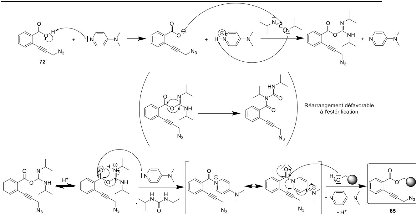
Schéma 114 : mécanisme du greffage sur résine de Wang d'acide 2-(3-azidoprop-1-yn-1-yl)benzoïque 72 par estérification de Steglich de 65
