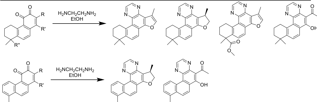
Schéma 13 : formation d'un CEE par synthèse de quinoxalinetanshinones à partir de tanshinones d'un extrait de Salvia miltiorrhiza Bunge [62]
