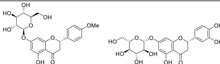
Figure 88 : produits de la coupure inter-osidique de la poncirine et de la O -déméthylation de l'hespéridine
