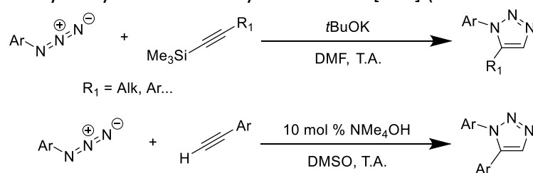
Schéma 66 : possibilités de synthèse de 1,2,3-triazoles 1,5-disubstitués avec emploi d'une base [259,260]
