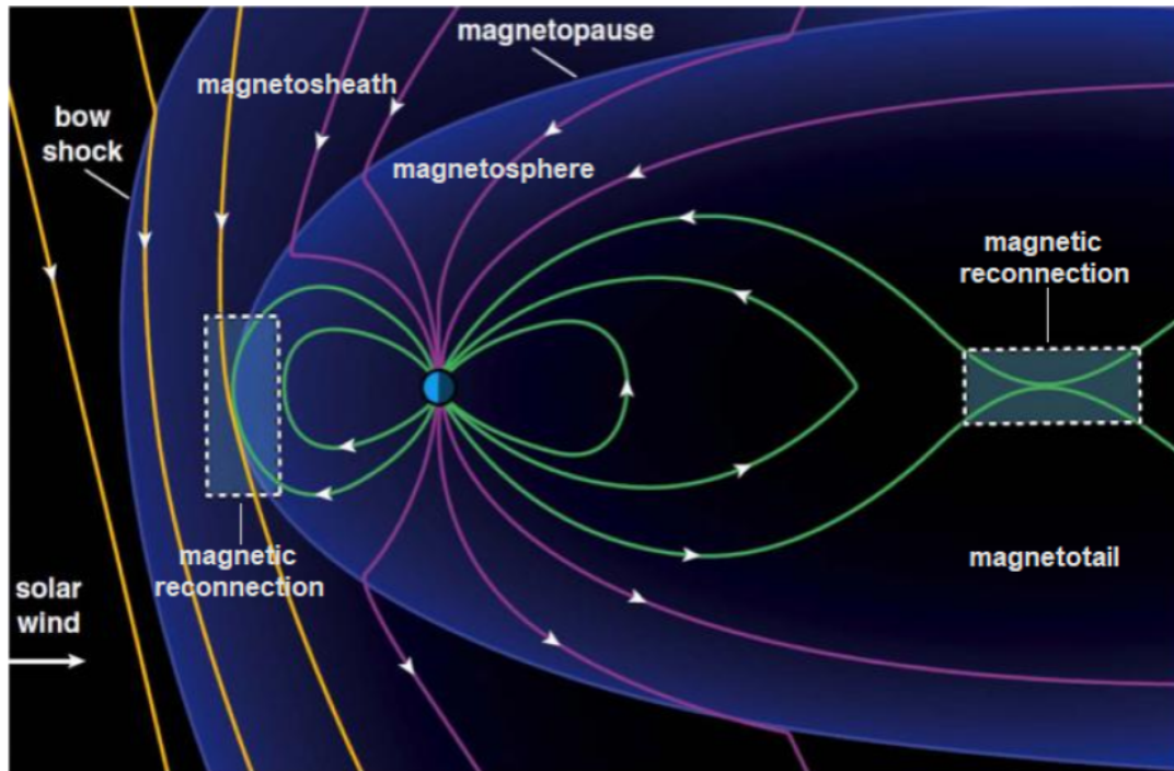
Figure 1.1: Figure montrant l'environnement plasma de la Terre.
