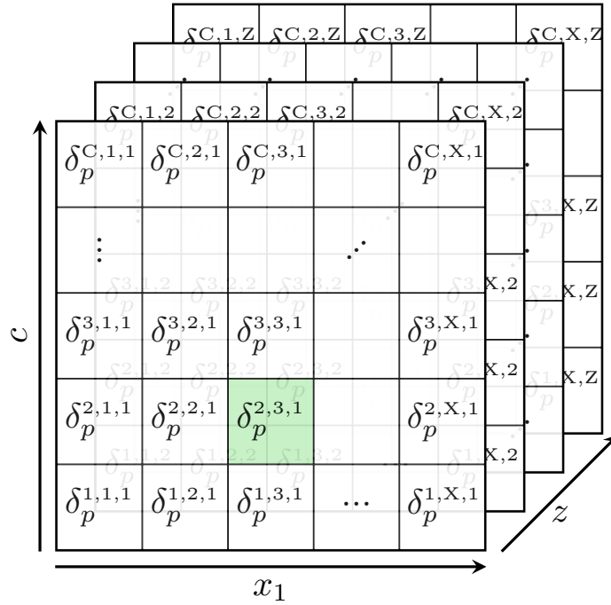
FIGURE VII.5 – Schéma de fonctionnement du découpage de l'échantillon BiasCor en 3 dimensions x_1 , c , z de la méthode BBC5D. Pour une supernova dont les valeurs de c , x_1 , z sont dans les intervalles 2, 3, 1, respectivement, les valeurs \delta_{m_B} , \delta_{x_1} et \delta_c seront celles issues de la cellule coloriee en vert.
