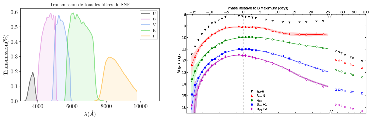
(b) Courbe de lumière en bandes UBVRI de la SN Ia confirmée SN2011fe avec ajustement par SALT2 (ligne pleine et bande pour son erreur). Figure de PEREIRA et al. (2013).
