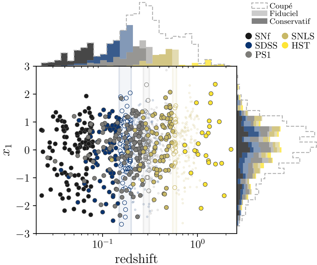
FIGURE V.9 – En bas : étirement des courbes de lumière ajustées avec SALT2.4 en fonction du redshift en échelle logarithmique pour chaque sondage de cette analyse (cf. légende). Les points pleins, creux et transparents correspondent aux échantillons conservatif, fiduciel et total, respectivement. En haut : histogrammes en redshift superposés, en sombre, clair et pointillé pour les échantillons conservatif, fiduciel et total, respectivement (cf. légende). À droite : histogrammes en étirement superposés. Notre hypothèse de travail se base sur le dépeuplement des étirements < -1 avec le redshift, que nous pouvons apercevoir dans les histogrammes de droite : relativement aux données x_1 > -1 , cette partie se peuple moins.
