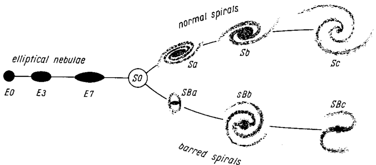
FIGURE III.1 – Classification morphologique des galaxies d'après HUBBLE (1936). De gauche à droite : galaxies elliptiques (E0-7), lenticulaires (S0) et spirales, barrées en bas (SBa-c) et non-barrées en haut (Sa-c).
