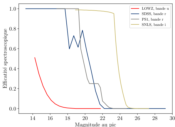
FIGURE V.4 – Comparaison des efficacités spectroscopiques des différents sondages. Figure produite avec les données de la collaboration Dark Energy Survey (DES, ABBOTT et al. 2019 ) pour LOWZ, de Pantheon ( SCOLNIC et al. 2018 ) pour PS1, et de Pantheon+ ( POPOVIC et al. 2021a ) pour SDSS et SNLS.
