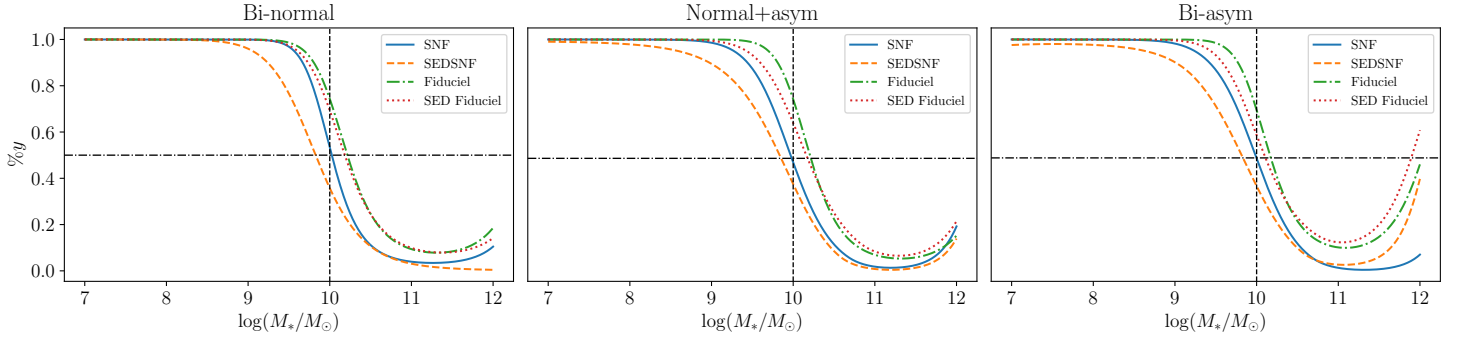
FIGURE VIII.4 – Comparaison de la prédiction de l'évolution de la fraction de jeunes SNe Ia ( \%y ) en fonction de la masse de la galaxie hôte ( M_* ) pour chaque modèle et selon chaque échantillon utilisé pour l'ajustement. Alors que le sens de variation devrait être constant, pratiquement tous les modèles finissent par remonter après M_* \approx 10^{11} M_\odot , sauf le modèle Bi-normal ajusté sur SEDSNf. Nous excluons les modèles Normal+asym et Bi-asym par ce critère.
