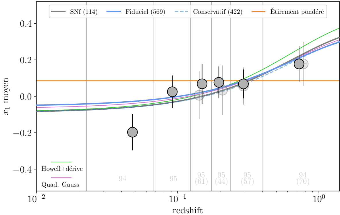
FIGURE VI.2 – Évolution de l’étirement moyen ( x_1 ) des SNe Ia issu d’un ajustement SALT2.4 en fonction du redshift pour notre modèle de base. Les marqueurs montrent la moyenne pondérée de l’étirement mesurée dans des intervalles de redshift de tailles d’échantillon égales, indiquées en gris clair en bas de chaque intervalle. Les marqueurs opaques et transparents sont utilisés lorsque les échantillons fiduciel ou conservatif sont considérés, respectivement. La ligne horizontale orange représente l’étirement pondéré des données. Les meilleurs ajustements de notre modèle de dérive de base sont présentés en bleu, bleu pointillé et gris lorsqu’ils sont ajustés sur l’échantillon fiduciel, conservatif ou l’ensemble de données SNfactory uniquement, respectivement ; ils sont tous compatibles entre eux et avec les données. La bande bleu clair illustre l’amplitude de l’erreur (covariance comprise) du modèle le mieux ajusté lorsque nous considérons l’ensemble de données fiduciel. Les lignes verte et violette représentent les meilleurs ajustements d’autres modèles dérivants, voir Sections VI.1.2, VI.2.2.
