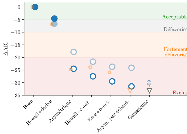
FIGURE VI.6 – \Delta\text{AIC} entre le modèle de base et les autres modèles, avec cette fois-ci en petits marqueurs oranges les résultats de l’étude pour un échantillon « super-conservatif » constitué de 244 SNe Ia. Le modèle Howell+dérive n’est pas fortement défavorisé par cette coupe, alors que les modèles non-dérivants y sont plus sensibles, tous voyant leur valeur d’AIC baisser significativement.
