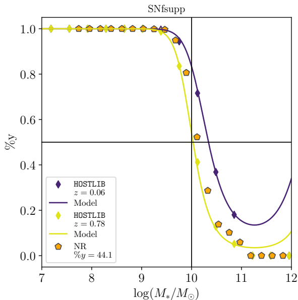
FIGURE VIII.6 – En violet (jaune) : fraction de jeunes étoiles en fonction de la masse pour le modèle de masse SNfsupp au redshift moyen de la HOSTLIB utilisée à hauts (bas) redshifts. En orange : même fraction mais pour l’échantillon simulé NR. Nous observons bien ici la suppression du modèle pour M_* > 10^{11} M_\odot .
