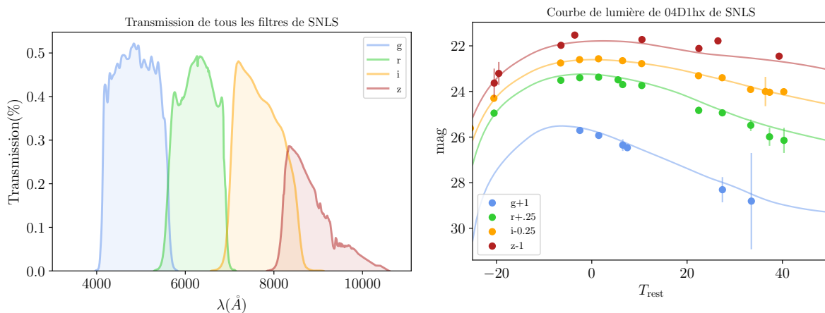
(b) Courbe de lumière en bandes griz de la SN Ia confirmée 04D1hx, à z = 0,56 . Figure produite avec les données du sondage et de l'analyse Pantheon (SCOLNIC et al. 2018).
