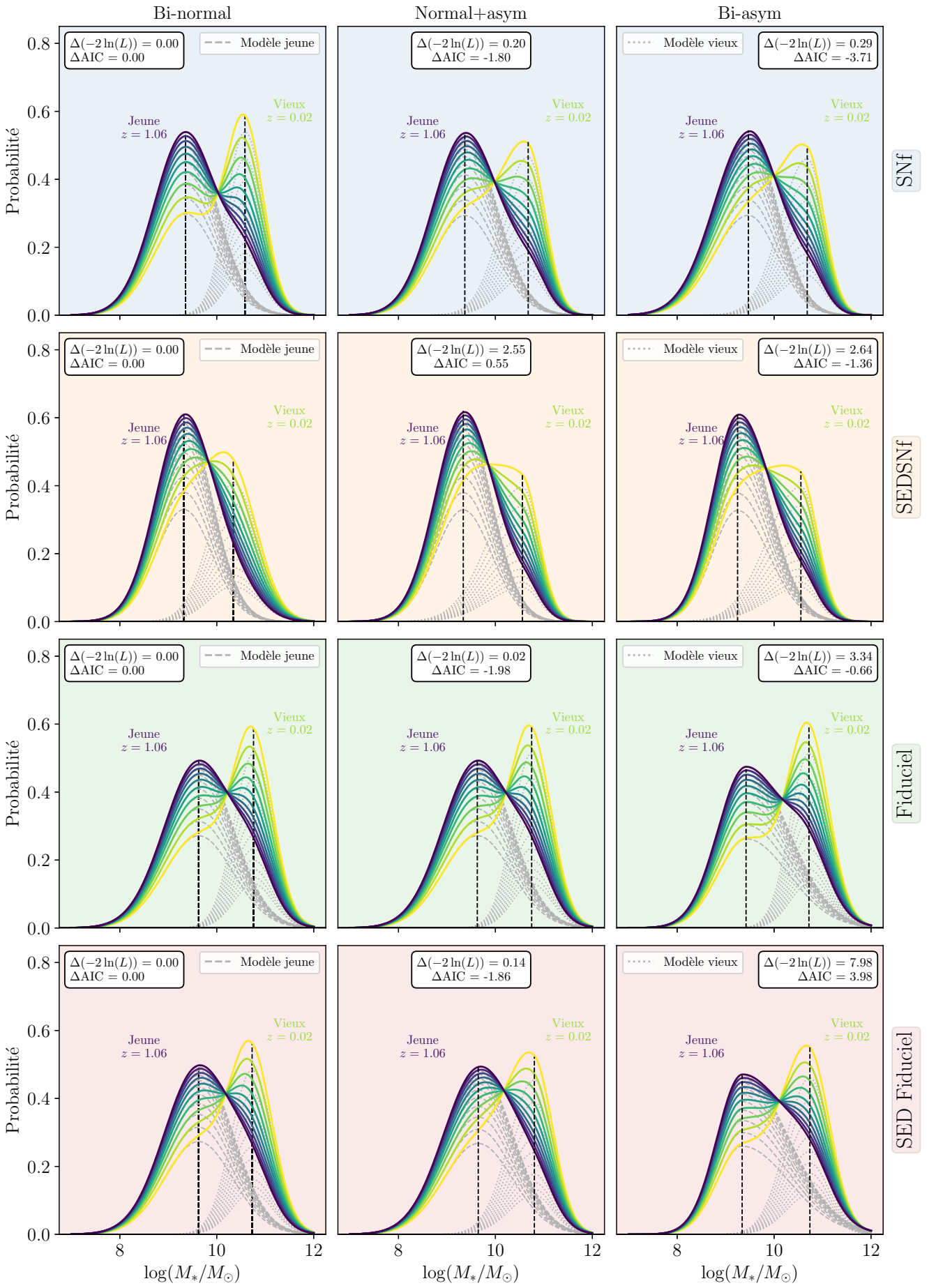
FIGURE VIII.3 – Modèles implémentés et testés dans l'étude de l'évolution de la masse avec le redshift. Les modèles Bi-normal, Normal+asym et Bi-asym sont tracés dans la colonne de gauche, du milieu et de droite, respectivement. Les échantillons sur lesquels ils sont ajustés correspondent aux lignes et à la couleur de fond du graphique : SNf (bleu), SEDSNf (orange), fiduciel (vert), fiduciel avec SEDSNf (rouge), correspondant aux mêmes couleurs que dans la Figure VIII.2. Les quantités \Delta(-2\ln(L)) et \Delta AIC par rapport au modèle Bi-normal de chaque ligne sont indiquées pour chaque modèle figure. Nous avons tracé dix réalisations des modèles selon la valeur du redshift moyen considéré, de la valeur la plus basse de notre échantillon ( z = 0,02 ) à la valeur maximale des données totales (sans coupe en redshift) de SNLS ( z = 1,06 ). Ces modèles sont représentés en couleur allant du jaune (bas redshift, plus vieux environnement) au violet (haut redshift, environnement jeune) et les distributions des populations jeune et vieille constituant le modèle total sont en gris pointillé et fin pointillé, respectivement. Nous y retrouvons l'information que tous les modèles sont compatibles en tant que bonnes représentations des données par rapport au modèle de base.
