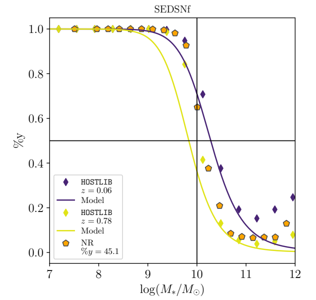
(c) Fraction pour SEDSNf.
