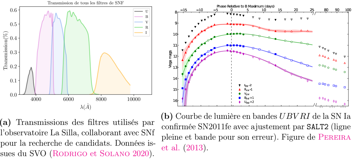
FIGURE IV.1 – Caractéristiques du sondage SNF.
