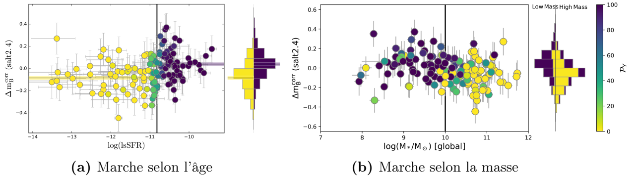
FIGURE III.6 – Marches de magnitudes selon l'âge (à gauche) ou la masse (à droite). Figures de RIGAULT et al. (2020). Pour chacune des figures, nous avons en encadré les différences entre les magnitudes corrigées des SNe Ia et le modèle cosmologique de référence en fonction du paramètre concerné ; et à côté les histogrammes pondérés par l'âge ou la masse. Les lignes horizontales représentent les moyennes des deux populations (et leurs erreurs). Les couleurs correspondent à la probabilité qu'une SN Ia soit jeune, voir barre de couleur. Nous observons que les SNe Ia vieilles sont plus lumineuses de -0,16 mag que les jeunes, alors que les SNe dans des environnements massifs ne le sont que de -0,12 mag.
