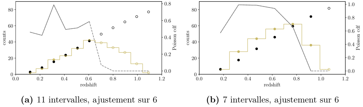
FIGURE V.1 – Exemple d’ajustement statistique pour deux tirages aléatoires d’histogrammes de SNLS.
