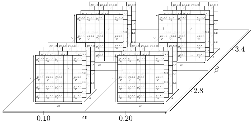
FIGURE VII.6 – Schéma de fonctionnement de la correction de biais à 5 dimensions de la méthode BCC5D : les paramètres \alpha et \beta sont générés sur une grille de taille 2 \times 2 , et à chacune des valeurs de cette grille sont associées les matrices de découpe de l'échantillon BiasCor en 3 dimensions : x_1 , c et z . Les valeurs finales à ajouter au module de distance de la SN simulée résulte de l'interpolation en 5D du meilleur ajustement.
