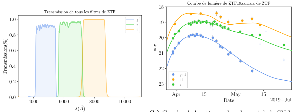
(b) Courbe de lumière en bandes gri de la SN Ia confirmée ZTF19aantarc, à z = 0,099 . Figure produite avec les données (à paraître) de la seconde publication du sondage via le module ztfidr 16 .
