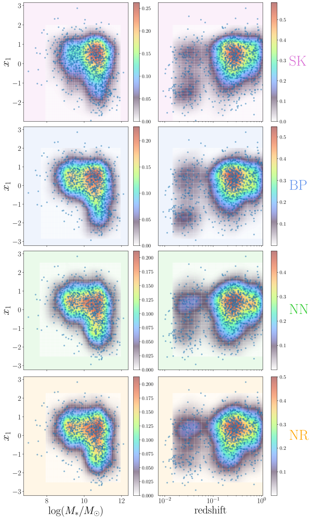
FIGURE VIII.10 – Accord données réelles (en points bleus transparents) et simulées (en couleur) en 2D pour tous les modèles. À gauche : étirement en ordonnée et masse en abscisse. À droite : étirement en ordonnée et redshift en abscisse. De haut en bas : modèles SK, BP, NN et NR, respectivement, voir légende. Les couleurs correspondent à celles de la Figure VIII.7.
