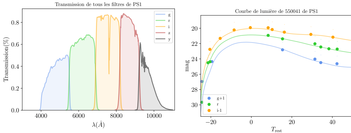
(a) Transmissions des filtres grizy de la caméra utilisée par PS1. Données tirées du SVO (RODRIGO et SOLANO 2020). (b) Courbe de lumière en bandes gri de la SN Ia confirmée 550041, à z = 0,26 .
