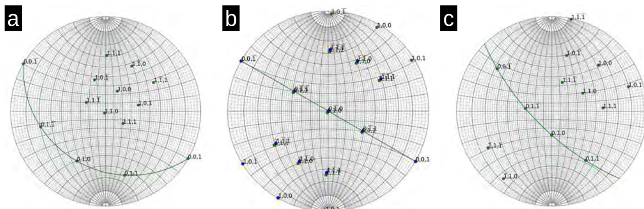
Figure 40 : Figures de pôle associées à l'orientation de la phase \varepsilon\text{-Fe}_2\text{O}_3 dans les dendrites de LHP-01 (a), LHP-02 (b) et BG-01 (c)
