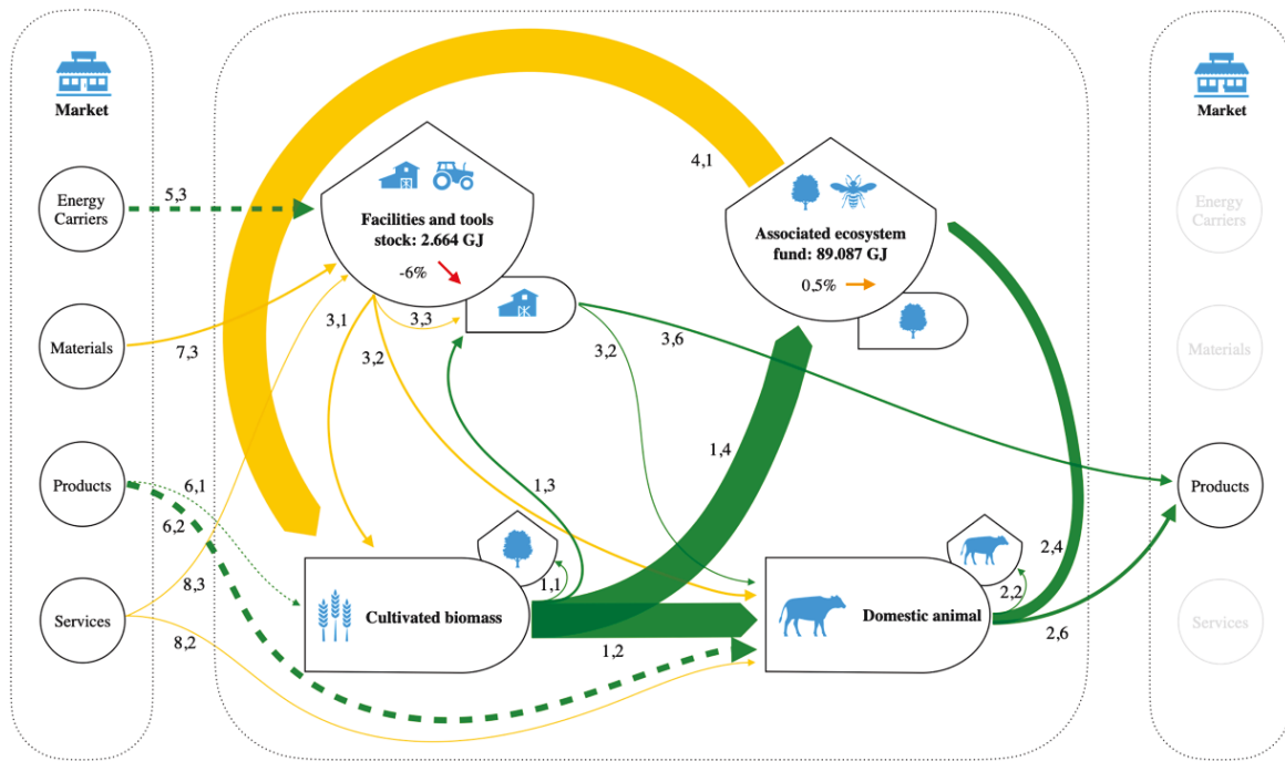
Figure 3: Diagramme des flux d'énergie du cas d'étude. L'épaisseur des flèches est proportionnelle à la valeur.
