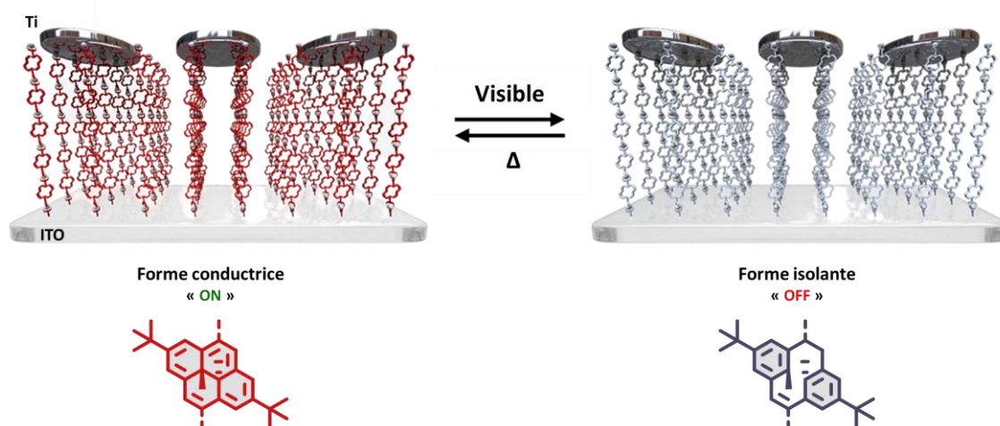
Figure 51 : Fils moléculaires commutables à base de DHP entre des électrodes d'ITO et de Titane. Reproduit avec la permission de Nanoscale. 10 Copyright 2018.
