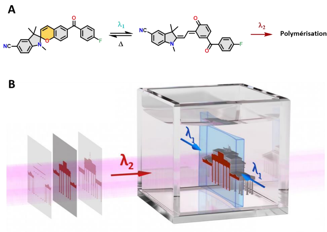
Figure 20 : A) Processus d'isomérisation et de polymérisation du dérivé spiropyrane synthétisé par l'équipe de Hecht. B) Illustration du nouveau procédé d'impression volumétrique proposé par Hecht : la Xolographie. Reproduit avec la permission de Nature. 102 Copyright 2020.
