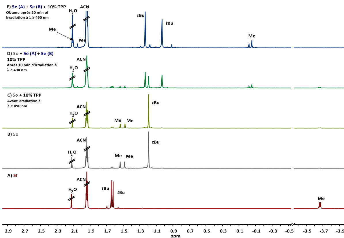
Figure 88 : Etude de la réaction entre 5o et ^1\text{O}_2 suivie par spectroscopie RMN ^1\text{H} . A) Solution initiale de 5f sous atmosphère inerte dans l'acétonitrile. B) Solution de 5o dans l'acétonitrile obtenue après irradiation sous atmosphère inerte de 5f à \lambda = 660 \text{ nm} . C) Solution B avec 10 mol% de tétraphénylporphyrine (TPP) sous atmosphère aérobie. D) Solution de C après 10 minutes d'irradiation à \lambda \geq 490 \text{ nm} . E) Solution de C après 20 minutes d'irradiation à \lambda \geq 490 \text{ nm} : les deux endoperoxydes 5e (A) et 5e (B) sont clairement identifiés. [C] \sim 2 \text{ mM} .
