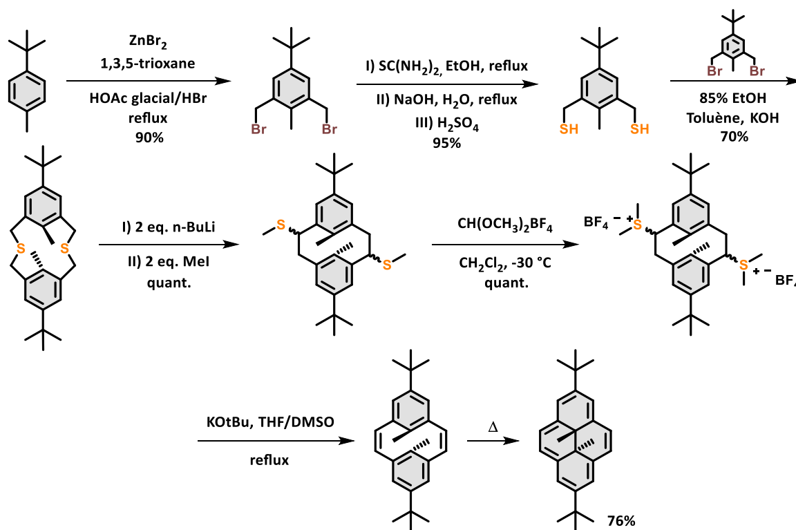
Figure 38 : Synthèse du composé 2,7-di- tert -butyl- trans -10b,10c-diméthyl-10b,10c-dihydropyrène (di- t Bu-DHP) 154,155,157 proposée par l'équipe de Mitchell.
