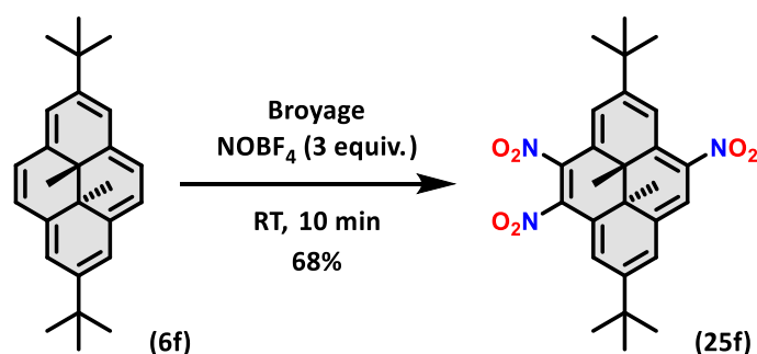
Figure 140 : Nouvelle voie de préparation de 25f par mécano-chimie.
