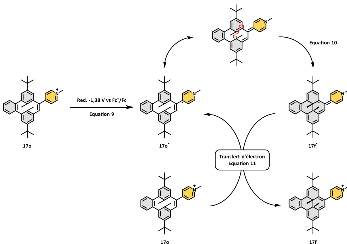
Figure 112 : Mécanisme de cyclisation auto-catalytique de 17o en 17f lors de la réduction à -1.38 V vs \text{Fc}^+/\text{Fc} .
