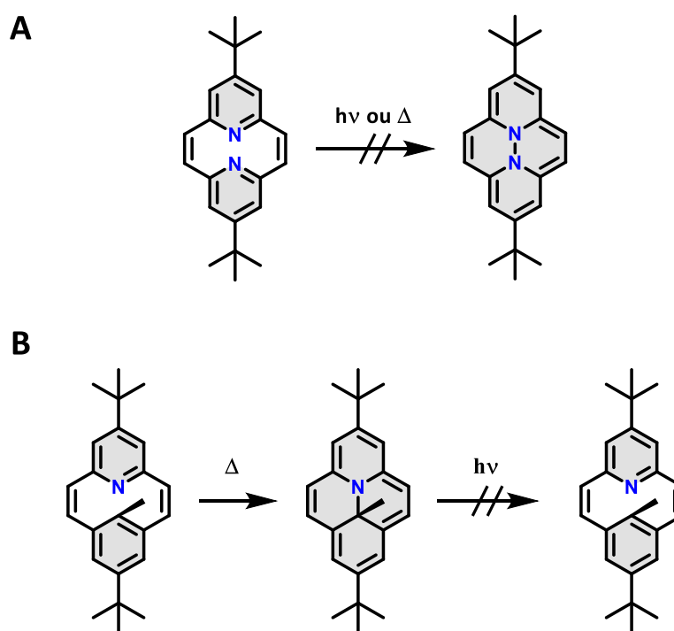
Figure 41 : A) [2,2](2,6)Pyridinophane-1,9-diène synthétisé par Boekelheide et Lawson 185 où aucune tautomérisation de valence n'a été observée. B) Dérivé [2.2]métacyclophanediène synthétisé par Chifuku et al. en 2007 186 montrant une fermeture thermique non réversible.
