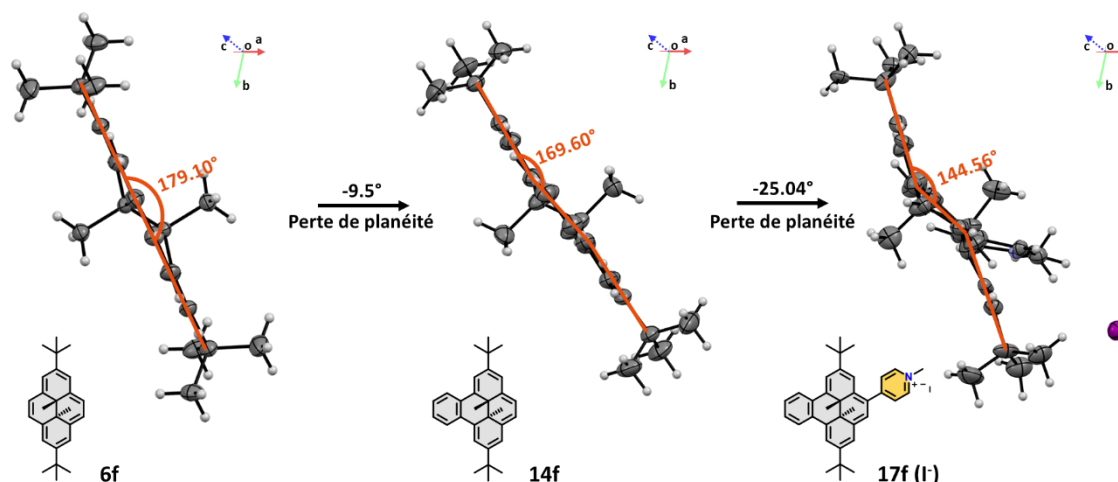
Figure 122 : Structures moléculaires des composés 6f , 14f et 17f déterminées par diffraction des rayons X et représentation de la perte de planéité entre ces différents dérivés. Ellipsoïdes représentés au seuil de probabilité de 50%.
