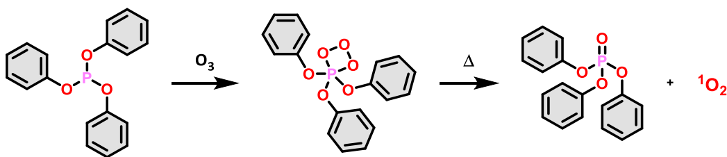
Figure 58 : Traitement du triphénylphosphite avec de l’ozone puis traitement thermique pour libérer une molécule de dioxygène singlet.
