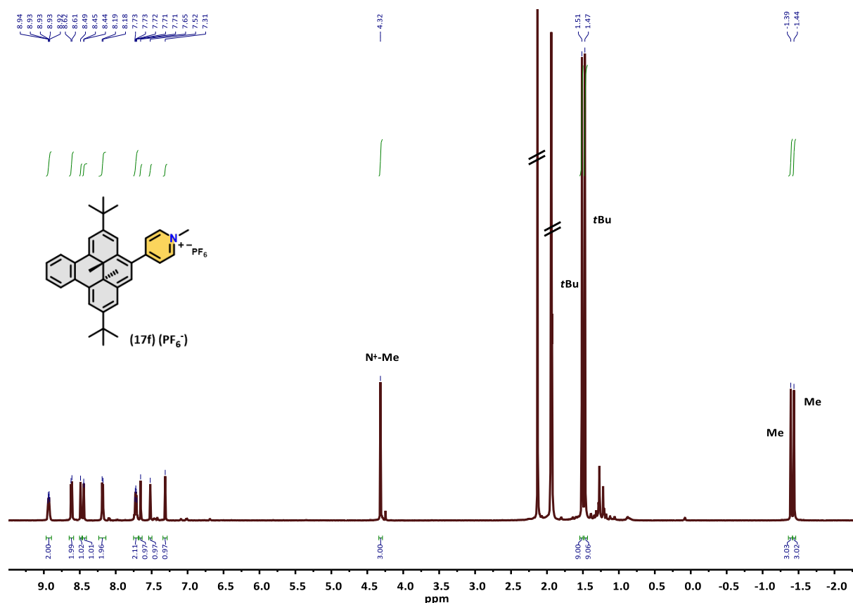
Figure 98 : Spectre RMN ^1\text{H} du composé 17f ( \text{PF}_6^- ) dans l'acétonitrile deutéré ( [\text{C}] = 2 \text{ mg/mL} ).
