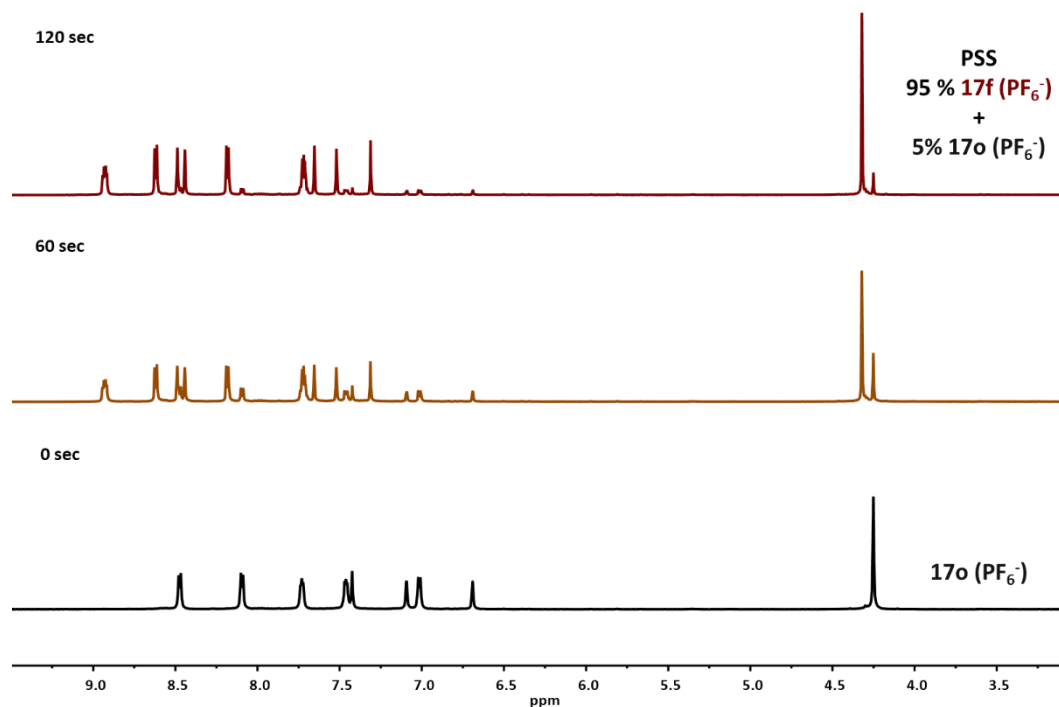
Figure 102 : Evolution des spectres RMN ^1\text{H} lors de l'irradiation de 17o ( \text{PF}_6^- ) dans l'acétonitrile deutéré à \lambda_{\text{exc}} = 470 nm. Au cours de l'irradiation les signaux du composé 17o ( \text{PF}_6^- ) sont progressivement remplacés par ceux de la forme fermée 17f ( \text{PF}_6^- ).
