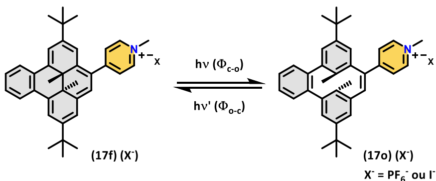
Figure 104 : Processus d'isomérisation d'ouverture et de fermeture du couple photochrome 17f/17o .
