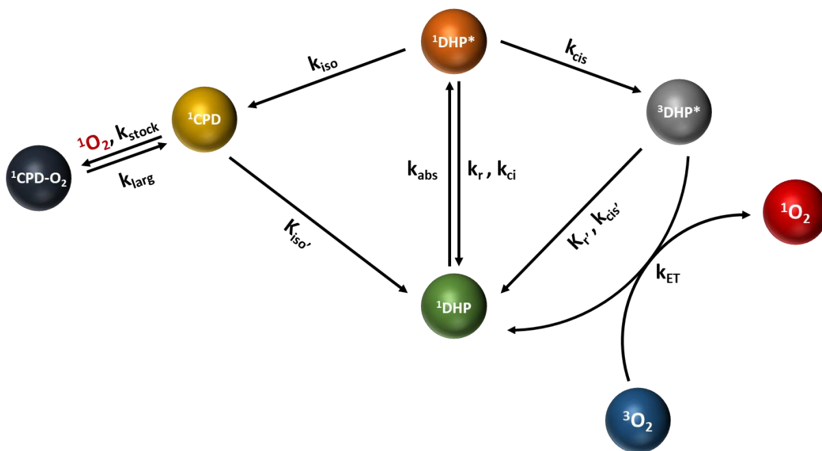
Figure 152 : Représentation schématique des processus photophysiques et photochimiques observables dans le système DHP.
