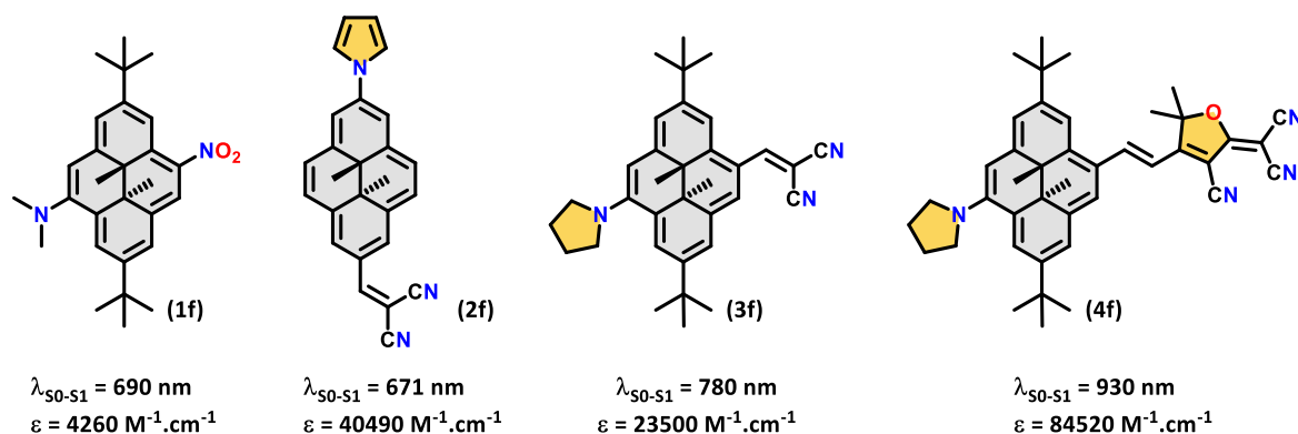
Figure 64 : Structures de composés de types donneur-accepteur de DHP préparés par l'équipe de Hecht. 242-244
