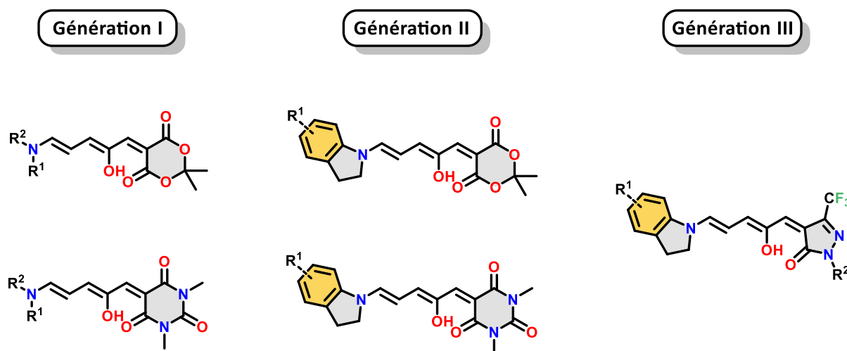
Figure 26 : Structure chimique générale des DASA's de génération I, II et III.
