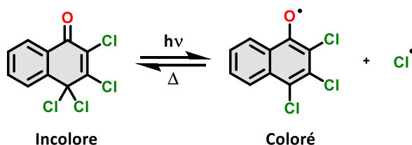
Figure 2 : « Phototropisme » à l'état cristallin du la 2,3,4,4-tétrachloronaphthalen-1(4H)-one ( \beta -TCDHN) proposé par Marckwald 20 en 1899.
