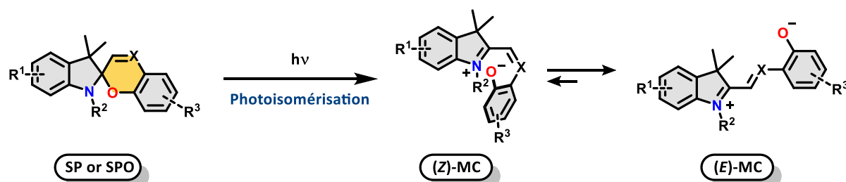
Figure 19 : Processus de la photoisomérisation chez les spiropyranes et les spirooxazines.
