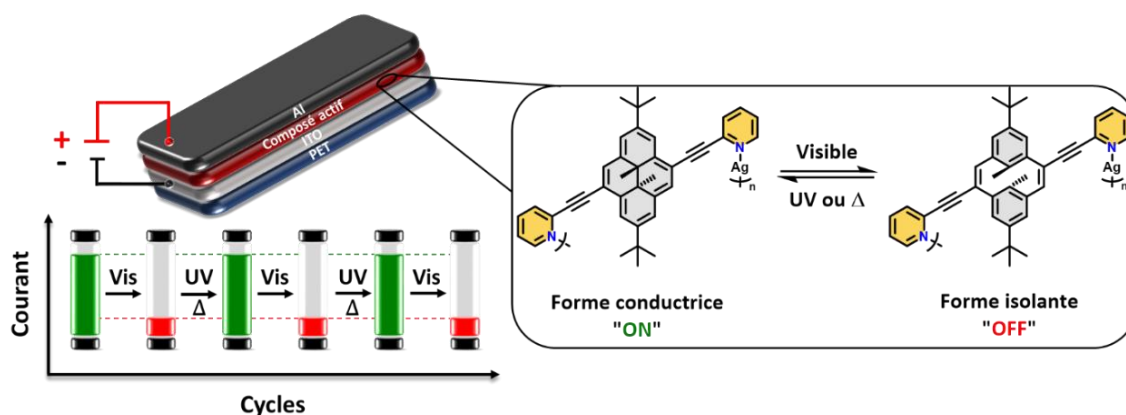
Figure 52 : Dispositif proposé par Bandyopadhyay et collaborateurs permettant de moduler la conductivité des formes ouvertes et fermées d'un polymère de coordination photochrome. Reproduit avec la permission de ACS Applied Materials & Interfaces. 202 Copyright 2020.
