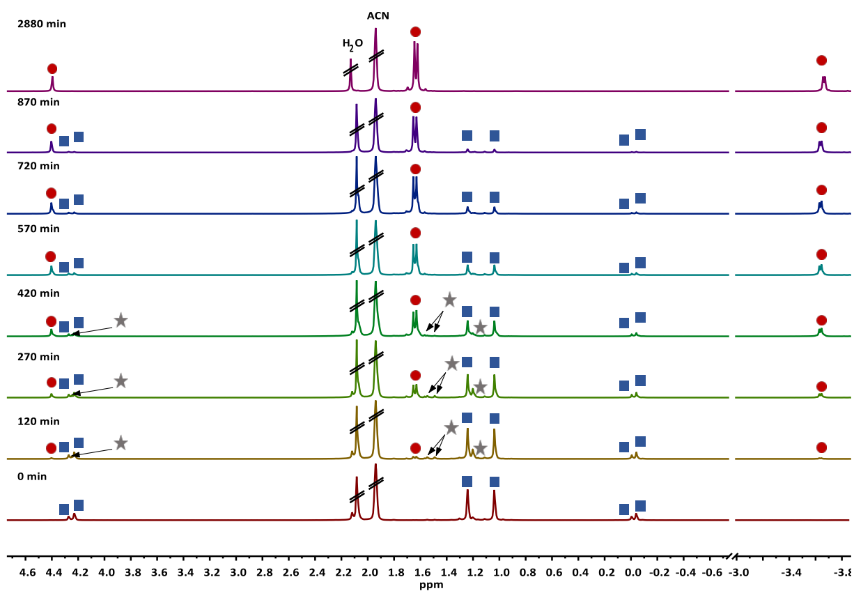
Figure 89 : Evolution des spectres RMN {}^1\text{H} lors du chauffage d'une solution fraîchement préparée des endopéroxydes 5e (2 mM) dans l'acétonitrile à T = 37\text{ }^\circ\text{C} . Les différents composés sont identifiés par les symboles suivants : 5f (●), 5o (★) and 5e (■).
