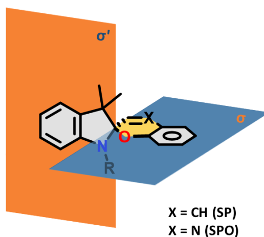
Figure 17 : Représentation des plans \sigma et \sigma' contenant les hétérocycles indoline et chromène pour un spiropyran (SP) ou une spirooxazine (SPO).
