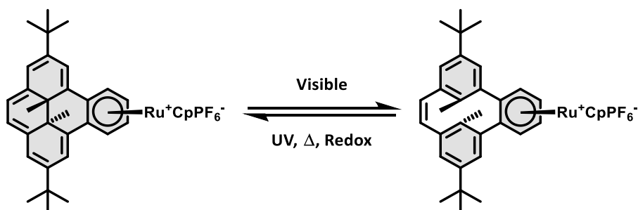
Figure 46 : Métallocène intégrant l'unité DHP présentant un retour électrochimique. 191
