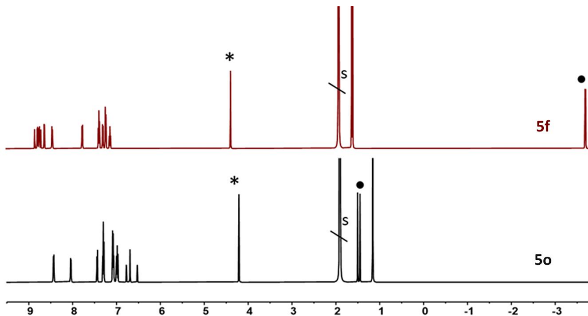
Figure 74 : Spectres RMN ^1\text{H} des composés 5f et 5o obtenus dans l'acétonitrile deutéré. Les symboles • et * indiquent respectivement les signaux relatifs aux méthyles internes et au groupement méthylpyridinium ( \text{N}^+\text{-CH}_3 ). s : solvant.
