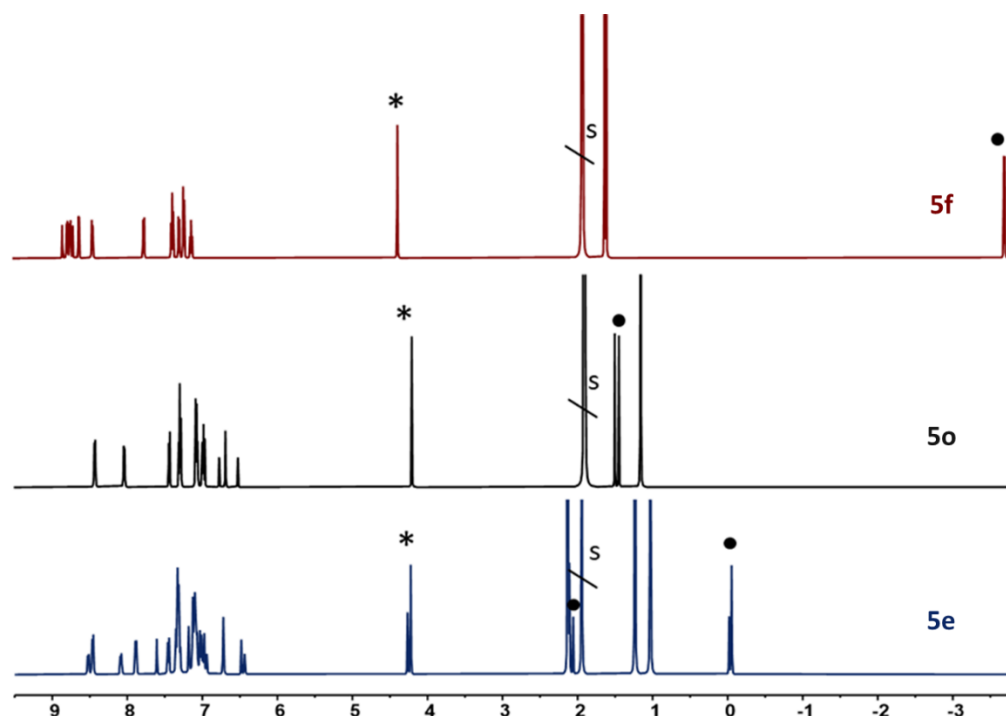
Figure 82 : Spectres RMN ^1\text{H} des composés 5f , 5o et 5e mesurés dans l'acétonitrile deutéré. Les symboles • et * indiquent respectivement les signaux relatifs aux méthyles internes et au groupement méthylpyridinium ( \text{N}^+\text{-CH}_3 ). s : solvant. 5e correspond à la forme endoperoxyde.
