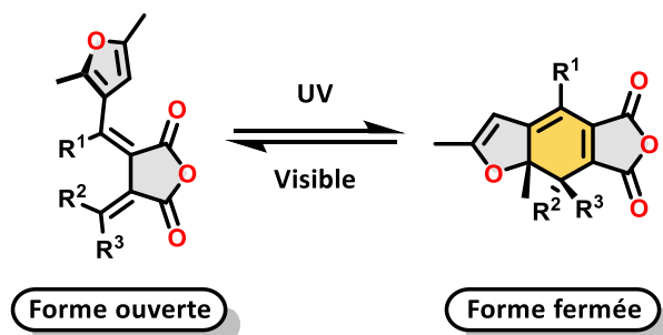
Figure 22 : Processus d'isomérisation entre la forme ouverte et fermée de fulgides.
