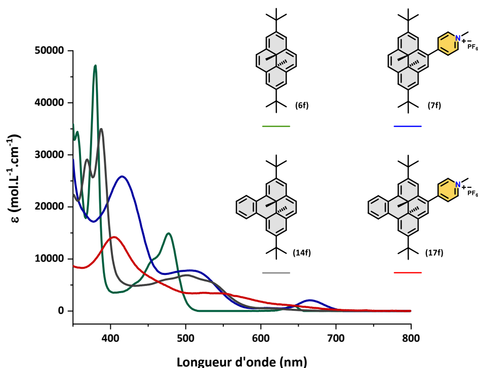
Figure 99 : Spectres UV-Vis des composés 7f et 17f ( \text{PF}_6^- ) (dans l'acétonitrile) et de 6f et 14f (dans le cyclohexane).
