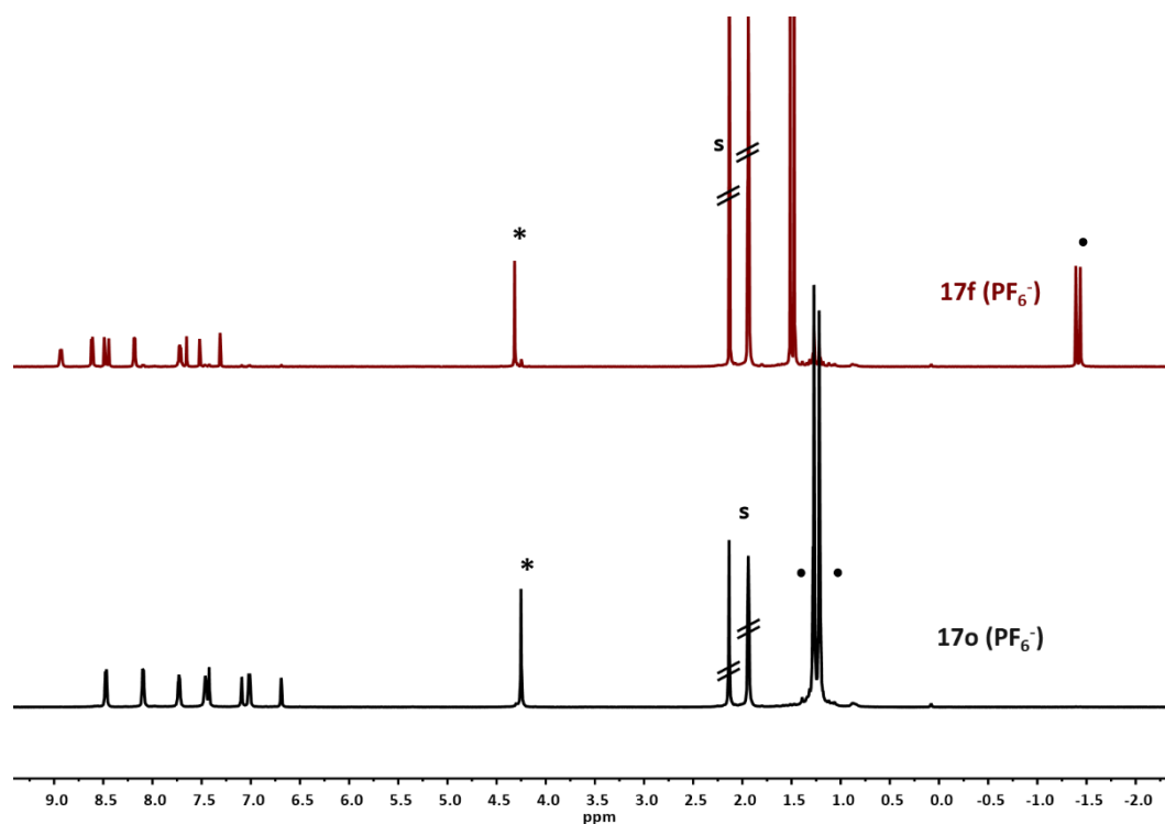
Figure 101 : Spectres RMN ^1\text{H} des composés 17f (haut) et 17o ( \text{PF}_6^- ) (bas) obtenus dans l'acétonitrile deutéré. Les symboles • et * indiquent respectivement les signaux relatifs aux groupements méthyles internes et méthylpyridinium ( \text{N}^+\text{-CH}_3 ), s : solvant.
