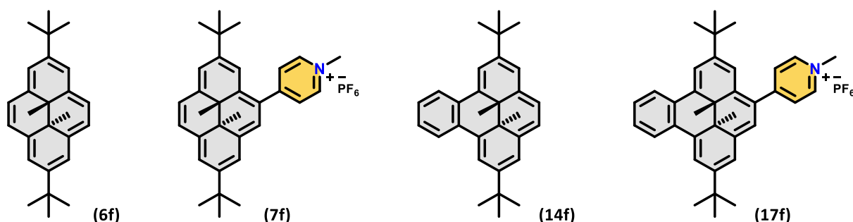
Figure 94 : Structures du composé benzo[e]pyridinium ciblé ( 17f ) et des molécules de référence étudiées ( 6f , 7f et 14f ) à titre de comparaison.
