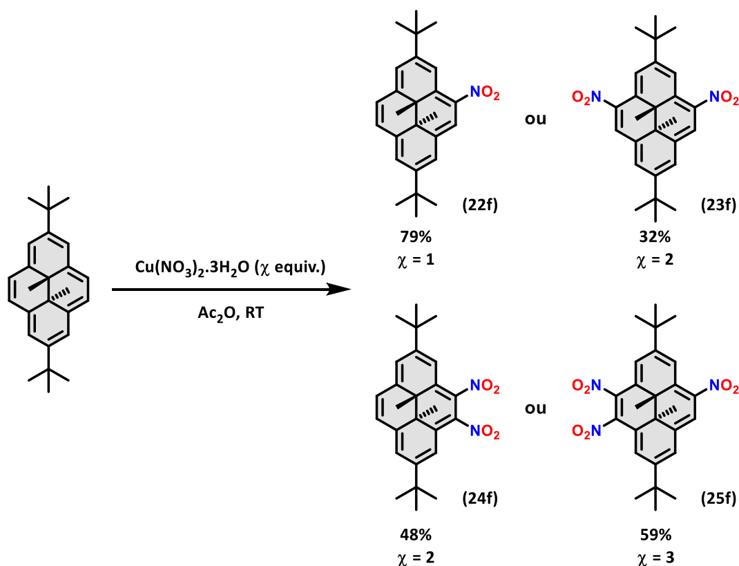
Figure 137 : Voie de synthèse proposée par l'équipe de Tashiro pour la préparation des composés 22f , 23f , 24f et 25f . 251
