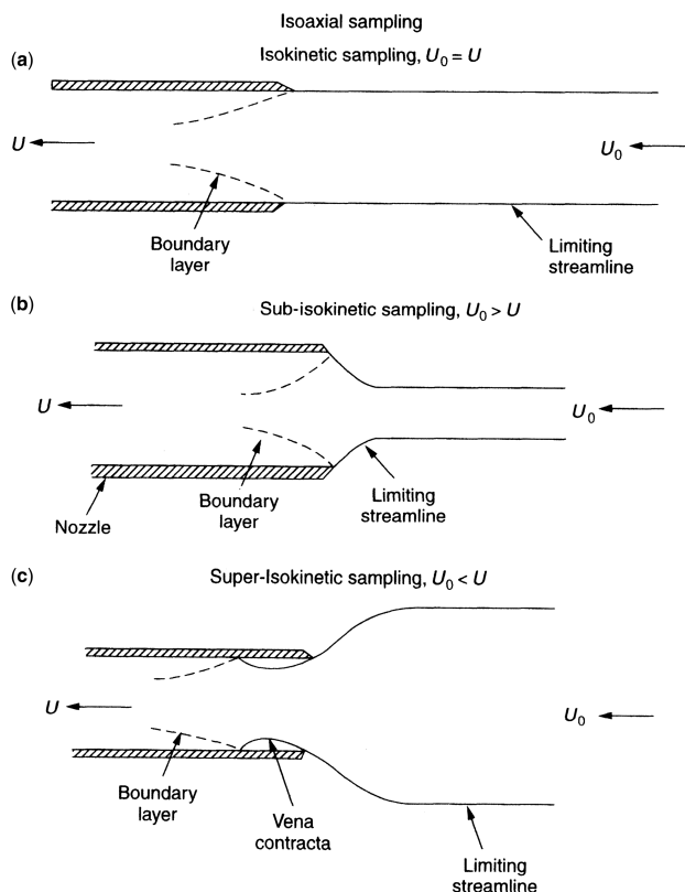
FIGURE 2.3 – Diagramme schématique d'un prélèvement isocinétique (a), super-isocinétique (b) et sub-isocinétique [18]
