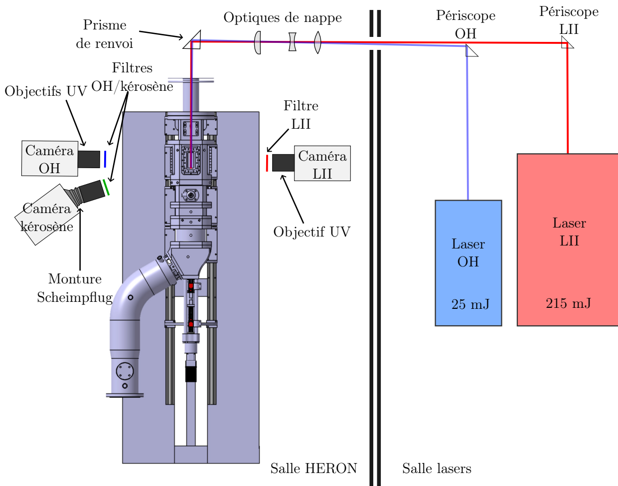
FIGURE 7.8 – Schéma du montage pour la mesure couplée de PLIF-OH/PLIF-kérosène/LII
