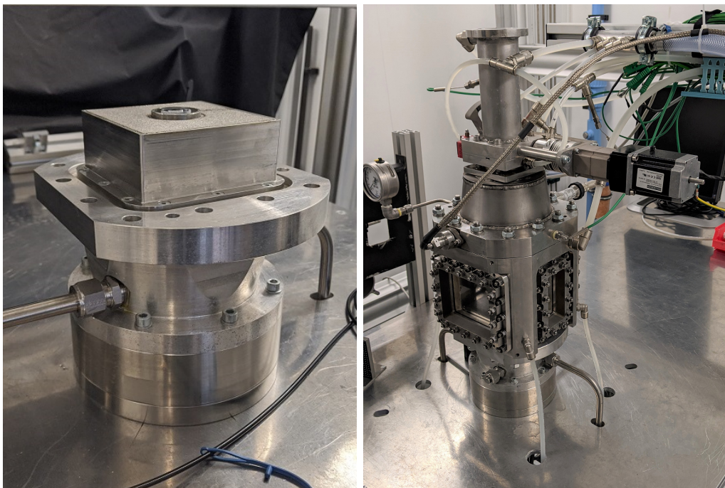
FIGURE 3.5 – Déclinaisons du brûleur SIRIUS. À gauche : en version atmosphérique. À droite, doté de son module à pression élevée
