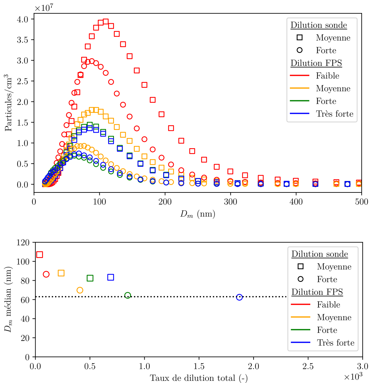
FIGURE 7.4 – Validation de la procédure de prélèvement à une pression chambre de 6 bar. En haut : distributions brutes obtenues. En bas : évolution du diamètre médian mesuré en fonction du taux de dilution global appliqué lors du prélèvement
