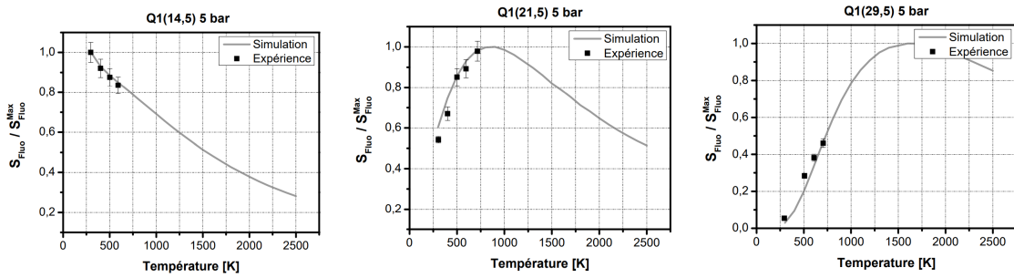
FIGURE 2.10 – Évolution de la fluorescence du NO en température pour les transitions Q_1(14,5) , Q_1(21,5) et Q_1(29,5) à une pression de 5 bar [65]
