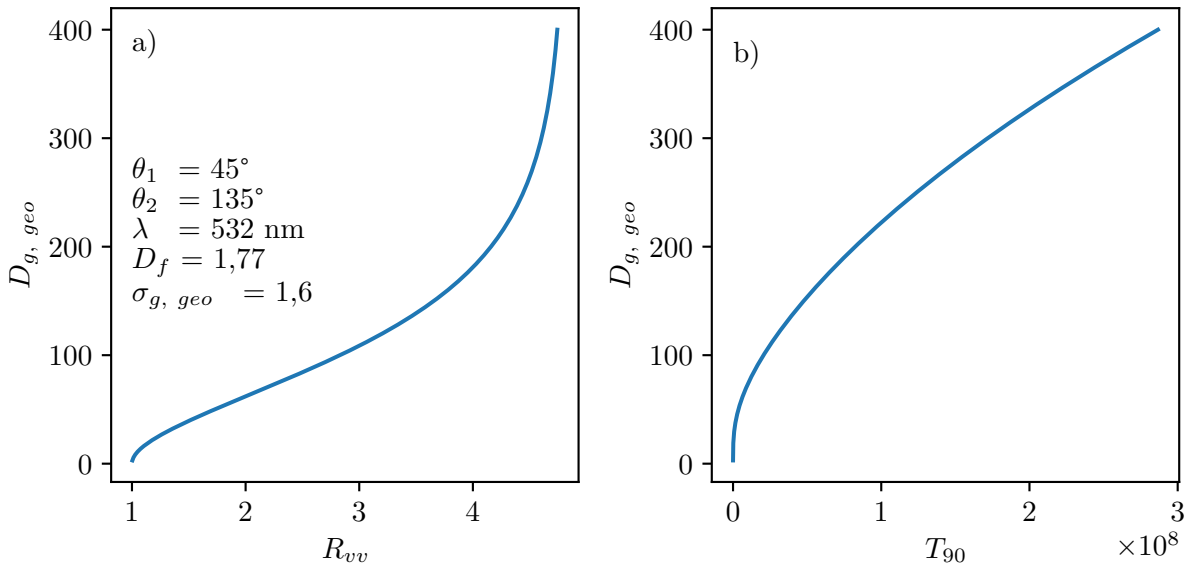
FIGURE 5.8 – Détermination du diamètre moyen géométrique a) et du paramètre de taille b) par méthode numérique, en supposant un modèle de diffusion RDG-FA et une population de type log-normale
