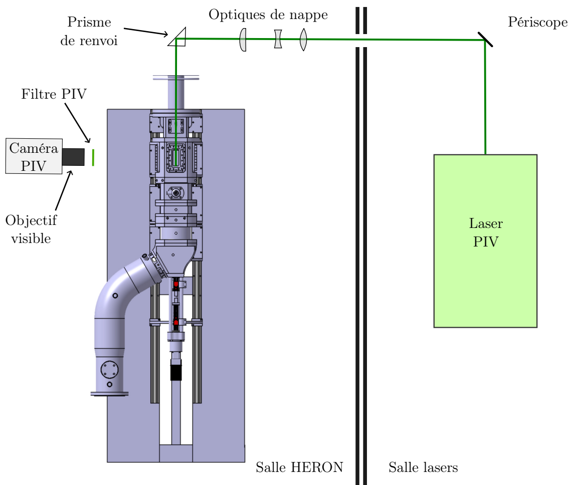
FIGURE 7.10 – Schéma du montage pour la mesure de PIV haute cadence
