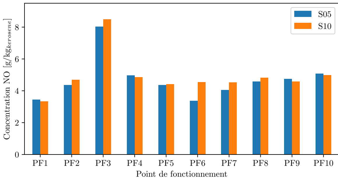
FIGURE 7.17 – Émissions de monoxyde d'azote NO en sortie de chambre - résultats globaux
