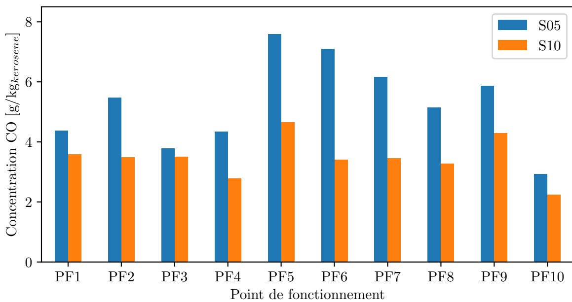
FIGURE 7.18 – Émissions de monoxyde de carbone CO en sortie de chambre - résultats globaux
