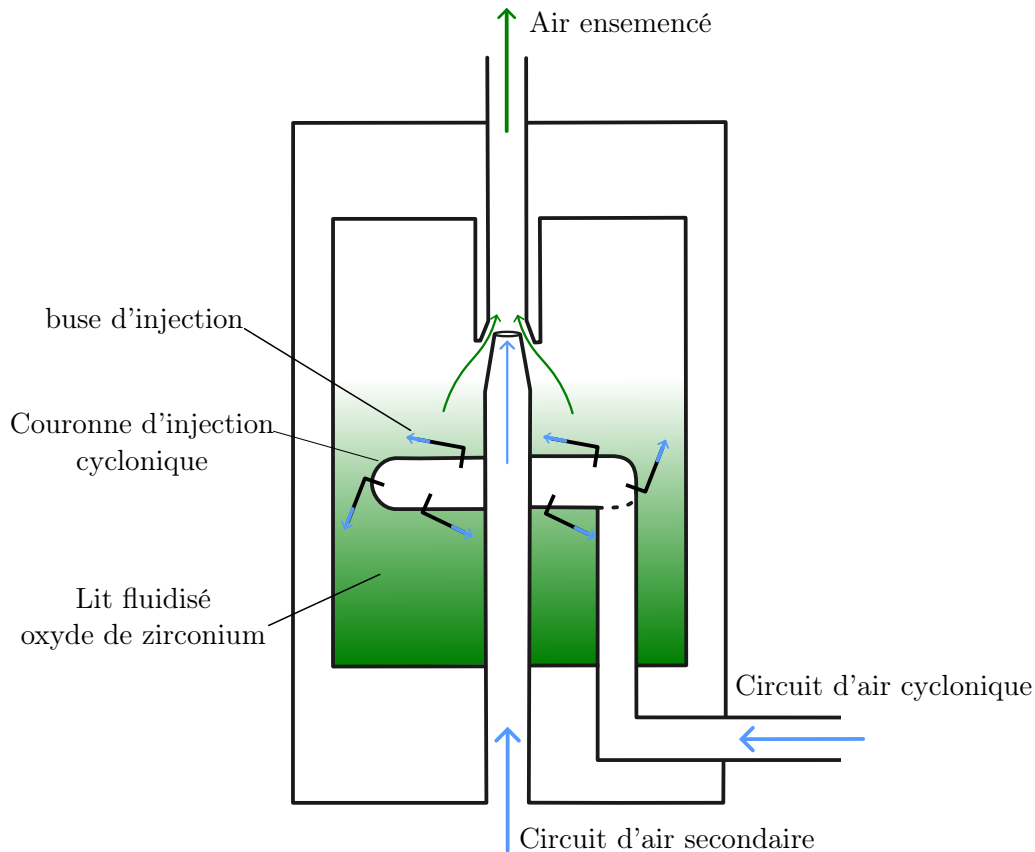
FIGURE 7.9 – Schéma simplifié du dispositif d'ensemencement utilisé sur le banc de combustion HERON
