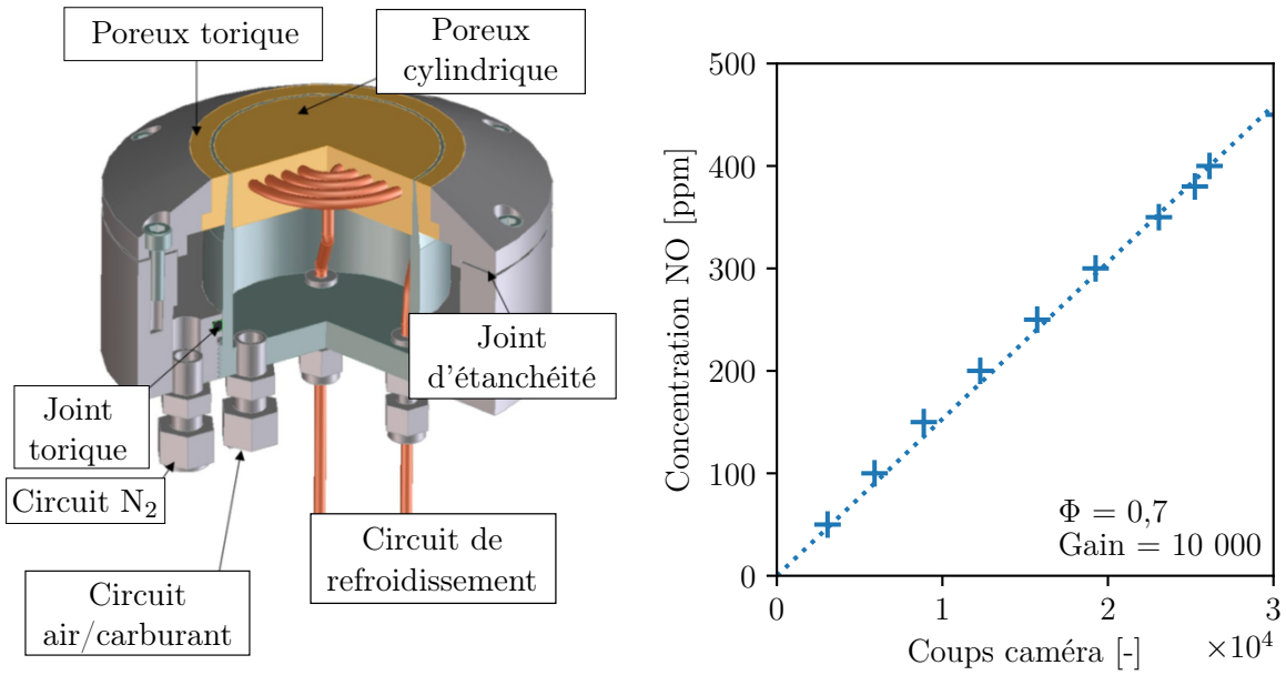
FIGURE 7.15 – Étalonage du signal de PLIF-NO. À gauche : représentation du brûleur laminaire de référence McKenna. À droite : résultats obtenus pour un gain caméra de 10 000
