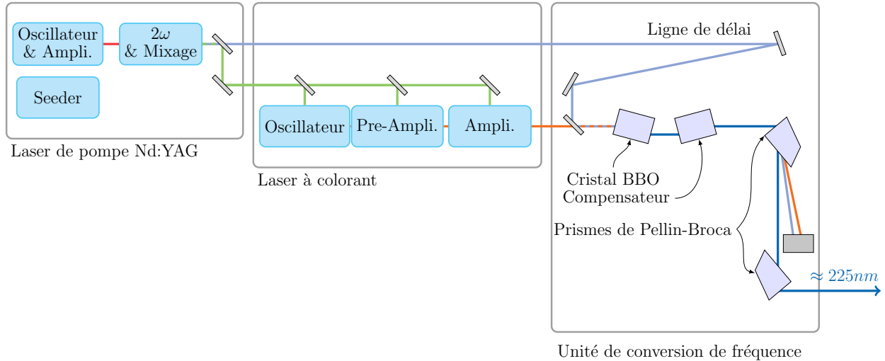
FIGURE 7.7 – Schéma du laser NO
