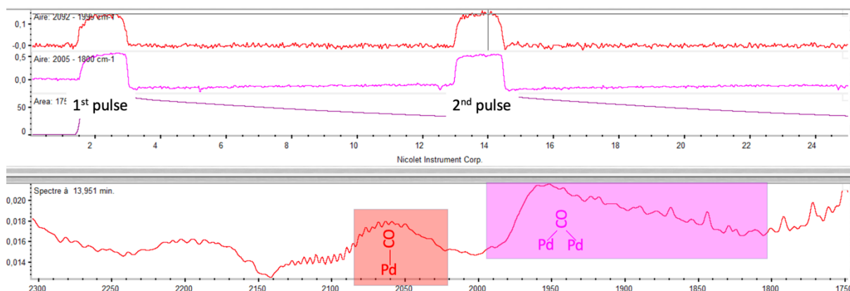
FIGURE 25 PARTIE INFÉRIEURE : SPECTRE IR CARACTERISTIQUE DE CZ(0-100) Pd EN MILIEU DE PLATEAU (PSEUDO-CRENEAU) A 250°C. PARTIE SUPERIEURE : CHIMIGRAMMES (PROFIL DE CONCENTRATION MOYEN) CARACTERISTIQUES DE CO ADSORBE SUR Pd.
