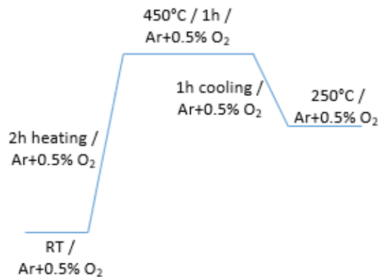
FIGURE 10 ETAPE D'ACTIVATION DU CATALYSEUR EN CONDITION 'OPERANDO'
