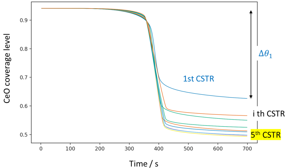
FIGURE 11 : EVOLUTION DU TAUX DE COUVERTURE DE CeO AU SEIN DE CHACUN DES CSTR CONSTITUANT LE REACTEUR DURANT UN PULSE DE CO SUR UN ECHANTILLON DE CZ 50-50 Pd A 250°C. DONNEES CALCULEES PAR LE MODELE CINETIQUE.
