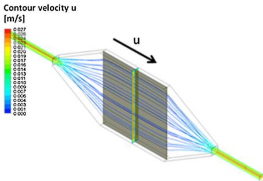
FIGURE 2 MODELISATION DES FLUX DE GAZ PASSANT AU TRAVERS DU PORTE ECHANTILLON CARRE, ADAPTE DE [1]
