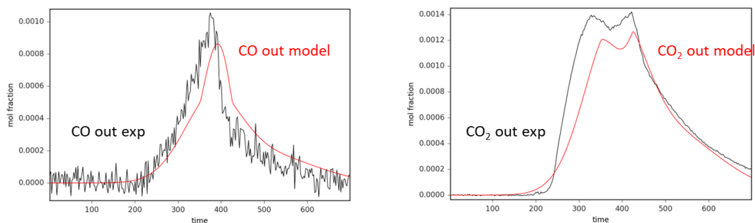
FIGURE 12 OPTIMISATION DES PROFILS DE CONCENTRATION SUR UN ECHANTILLON DE CZ 50-50 Pd A 250°C EN UTILISANT LES EQUATIONS DE REACTION 2, 4, 7, 8 ET 9. PROFILS DE CONCENTRATION EN ENTREE DU REACTEUR POUR LA MODELISATION CINETIQUE OBTENUS A PARTIR D'UN BLANC ENREGISTRE A TEMPERATURE AMBIANTE.
