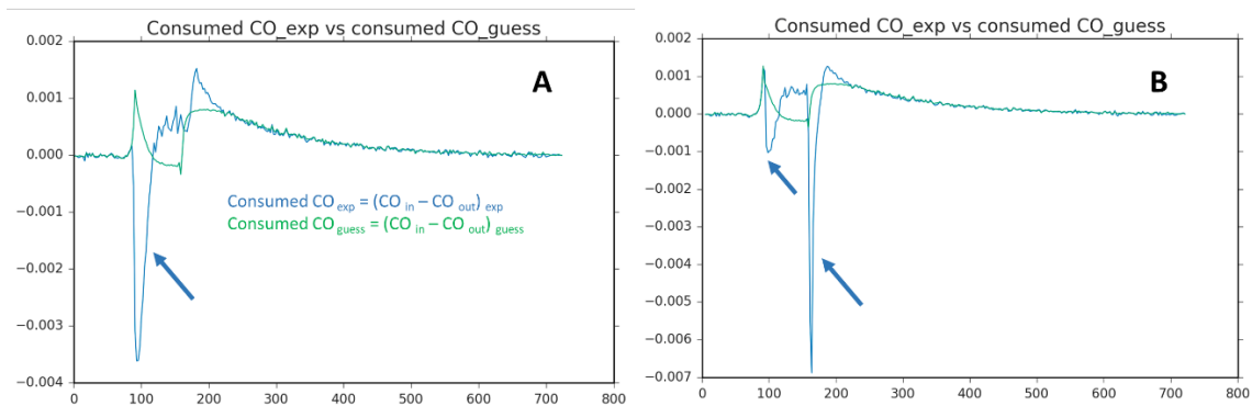
FIGURE 18 COMPARAISON DE LA CONSOMMATION DE CO, A) SANS DECALAGE TEMPOREL ET B) AVEC UN RECALAGE TEMPOREL DU BLANC DE +5 SECONDES. CO IN = PROFIL OBTENU POUR UN BLANC EFFECTUE A TEMPERATURE AMBIANTE. CO OUT = PROFIL OBTENU POUR UN TEST EN PRESENCE DE CZ(0-100) RH EFFECTUE A 300°C.
