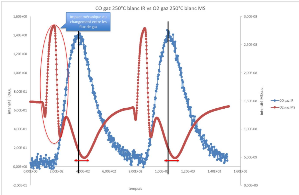
FIGURE 4 COMPARATIF DES SIGNAUX OBTENUS ENTRE LE CO ET L'OXYGENE DURANT UN BLANC
