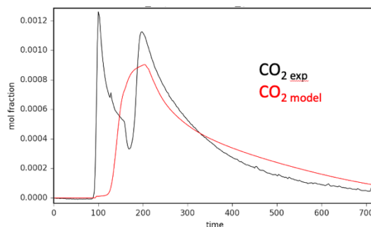
FIGURE 22 MODELISATION DE LA PRODUCTION DE CO 2 A 250°C SUR CZ(0-100) RH EN CONSIDERANT L'ADSORPTION REVERSIBLE DE CARBONATES SUR UN SEUL TYPE DE SITES SUPERFICIELS Zr 2 O 3 . OPTIMISATION REALISEE EXCLUSIVEMENT SUR L'ACCORD ENTRE LES DONNEES EXPERIMENTALES ET MODELISEES POUR LE CO 2 GAZEUX.
