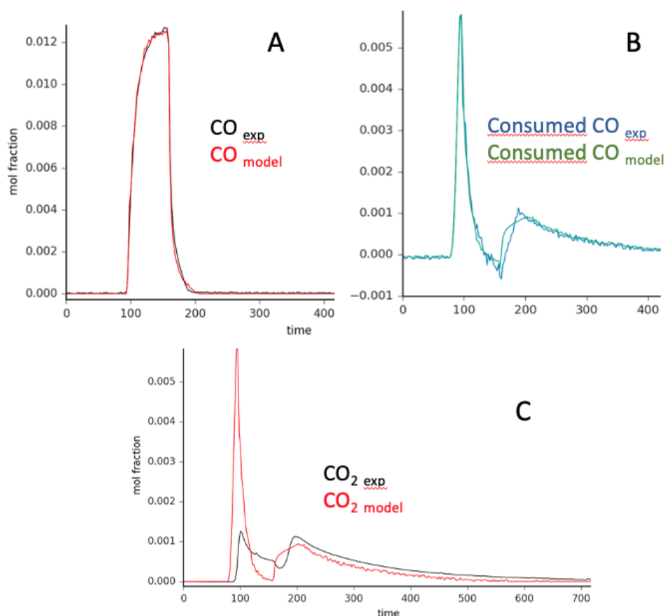
FIGURE 21 MODELISATION A PARTIR DU MECANISME REACTIONNEL PRESENTE AU TABLEAU 4, A) DU PULSE DE CO GAZ, B) DU CO CONSOMME ET C) DE LA PRODUCTION DE CO 2 A 250°C POUR CZ(0-100) RH
