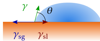
FIGURE 1.12 – L'équilibre mécanique sur la ligne triple permet d'obtenir la valeur de l'angle de contact \theta à partir des tensions de surface entre le liquide et le gaz \gamma , le solide et le liquide \gamma_{sl} et enfin le solide et le gaz \gamma_{sg} .
