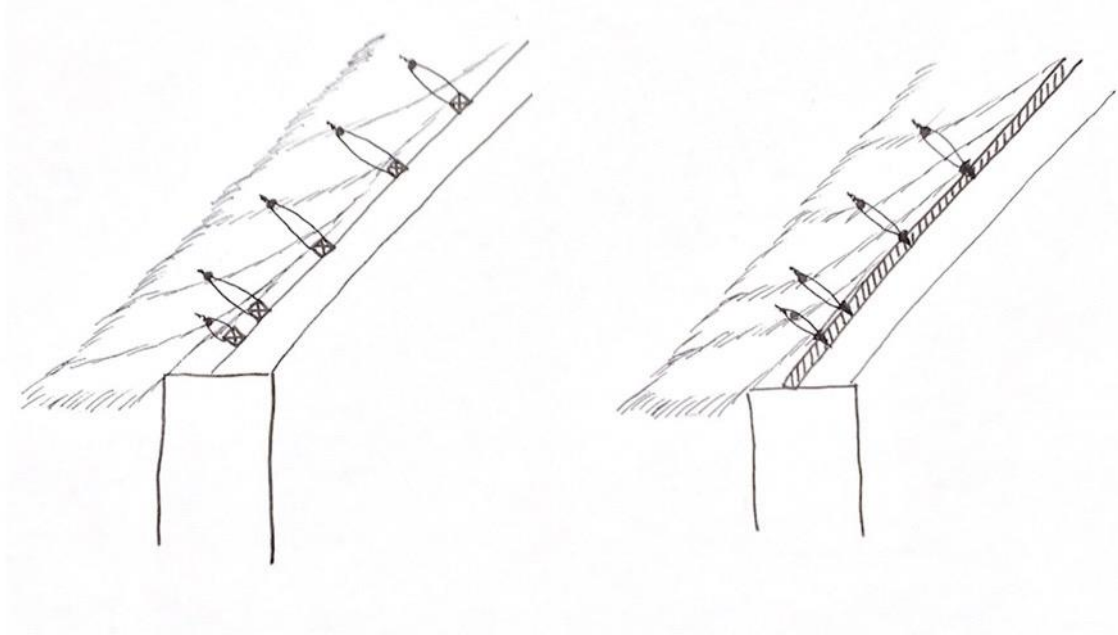
Figure 6 : Croquis de la technique traditionnelle sur liteaux et de la technique vissé sur OSB, crédit Carole Lemans
