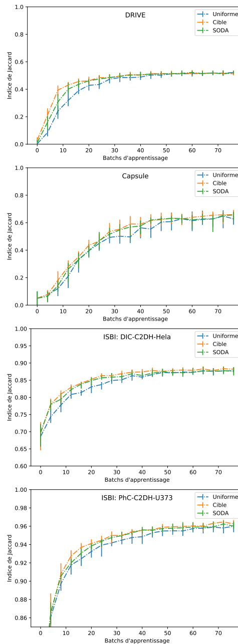
FIGURE 4.1 – Indices de Jaccard moyens (sur 10 exécutions) pour les 4 jeux de données et les trois stratégies d'allocation au cours de l'apprentissage, divisé en batchs de taille 80.
