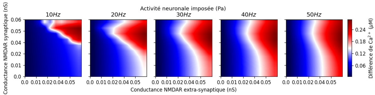
FIGURE 3.4 – Différence moyenne de concentration en calcium post-synaptique (gliotransmission - pas de gliotransmission) sur l'ensemble de la simulation, en fonction des conductances NMDAR synaptique (ordonnées) et extra-synaptique (abscisses), pour les 5 fréquences d'activité neuronale testées.
