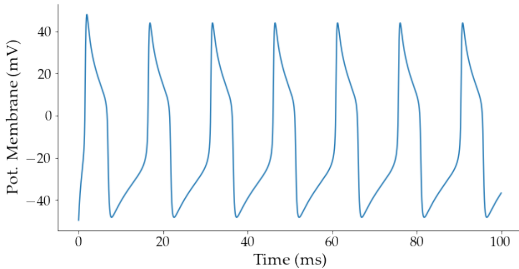
FIGURE 2.8 – Modélisation du neurone selon MORRIS et LECAR (1981). Les paramètres utilisés sont : C = 1 \mu F.cm^{-2} , g_L = 2 mS.cm^{-2} , g_{Ca} = 4 mS.cm^{-2} , g_K = 8 mS.cm^{-2} , V_L = -50 mV , V_{Ca} = 100 mV , V_K = -70 mV , \lambda_{n_{max}} = 0.1 ms^{-1} , V_1 = -1 mV , V_2 = 15 mV , V_3 = 10 mV , V_4 = 14.5 mV , I = 50 \mu A.cm^{-2} .
