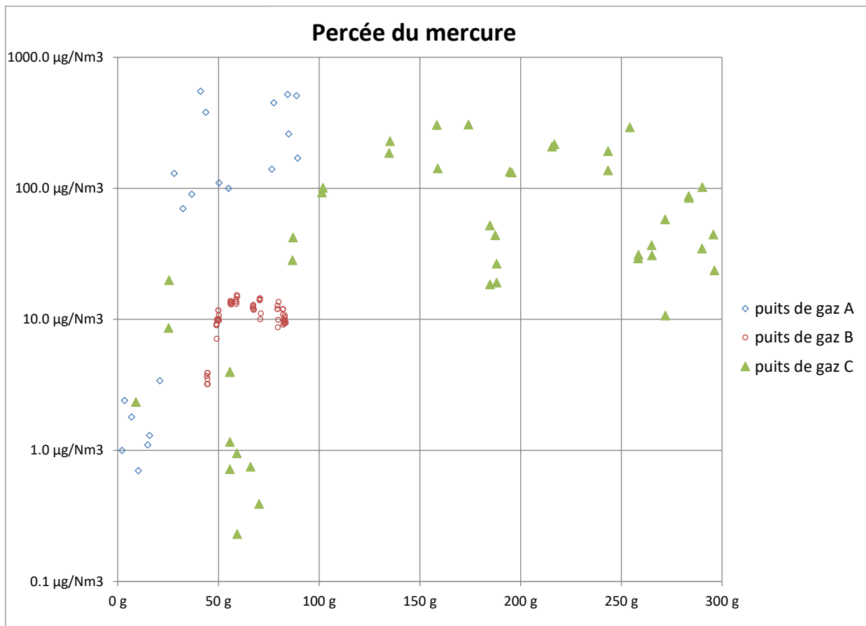
Figure 15. Temps de "percée du mercure" obtenu en fonction de la quantité totale produite estimée lors de trois tests de puits
