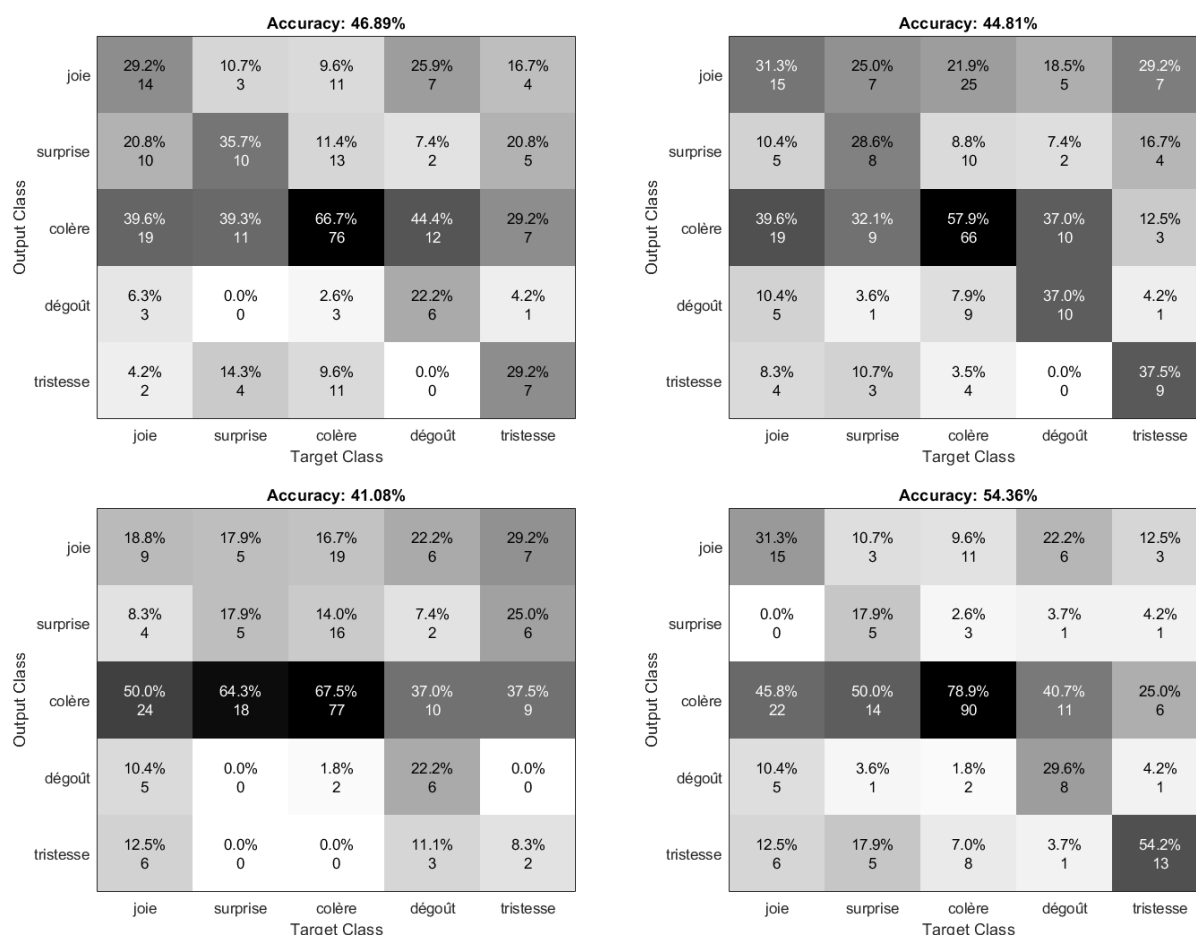
FIGURE 5.4 – Matrices de confusion obtenues sur le système complet à partir de quatre méthodes d'estimation de l'apex : (en haut, à droite) le \chi^2 du LBP, (en haut, à gauche) le \chi^2 HOOF, (en bas, à droite) la somme du flot optique et (en bas, à gauche) la durée moyenne d'une ME (DMME).
