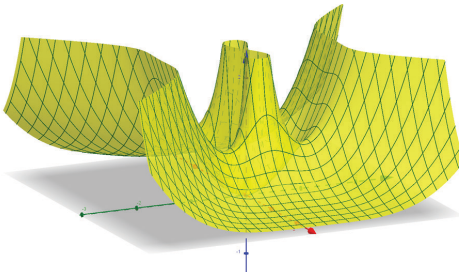
Graphes de g_1/g_2 . On voit une « explosion » au centre, qui montre que la division n'est plus « au moins aussi forte ».
