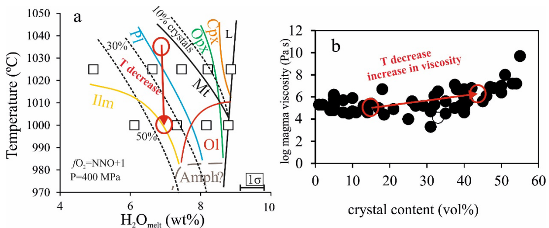
Figure 7-18: Diagramme de phase d'une andésite à 4 kbar. L'augmentation de la teneur en cristaux lorsque la température diminue de 35 °C (modifié d'après Andújar et al. 2017). b) Evolution de la viscosité en fonction de la teneur en cristaux dans les magmas (modifié d'après Andújar and Scaillet 2012).
