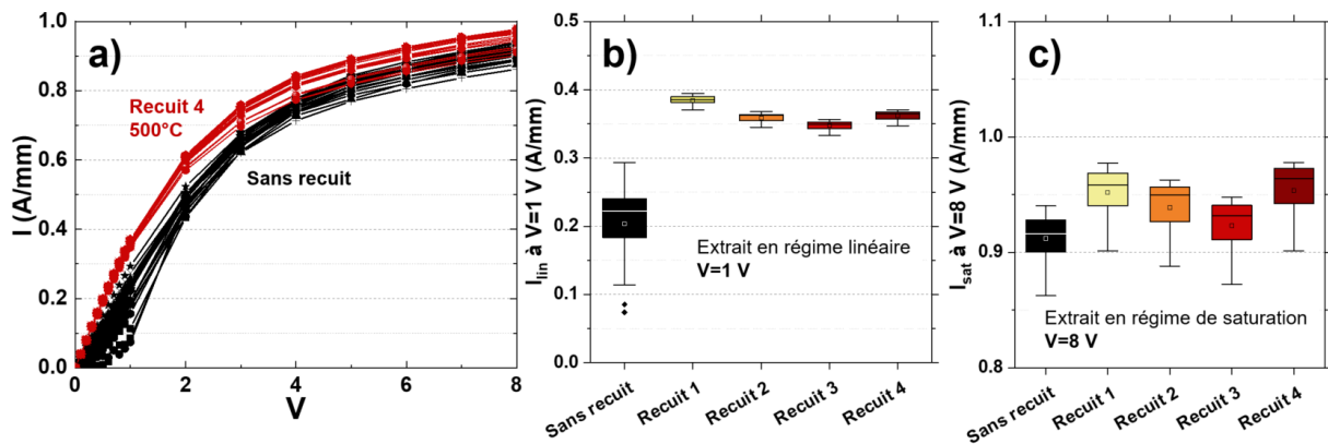
Figure 89 : a) Caractéristique I-V sur un motif TLM espacé de 1,5 \mu\text{m} en fin de fabrication et pour le recuit n°4. b) Courant extrait en régime linéaire (à V=1 V) sur le TLM espacé de 1,5 \mu\text{m} pour tous les recuits. c) Courant extrait en régime de saturation (à V=8 V) sur le TLM espacé de 1,5 \mu\text{m} pour tous les recuits.
