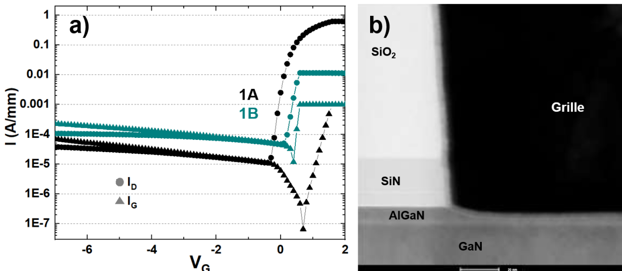
Figure 27 : a) Caractéristiques de transfert des wafers 1A et 1B. b) Image STEM en coupe du pied de grille du wafer 1A.
