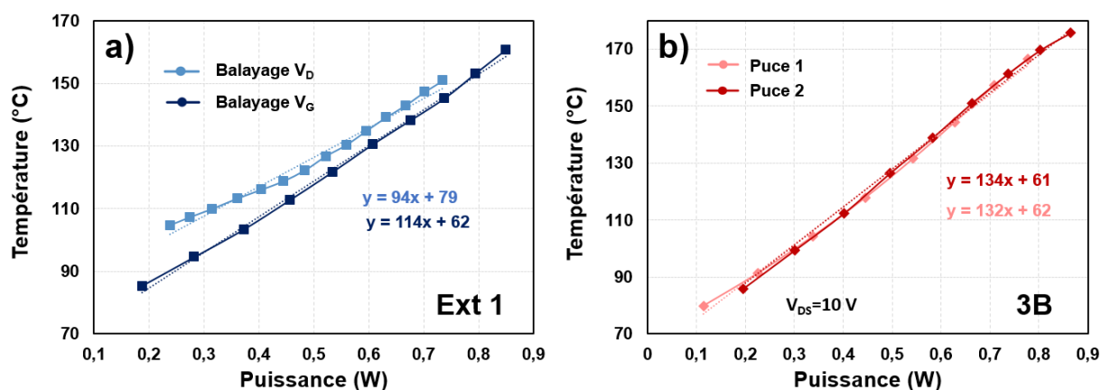
Figure 96 : a) Caractéristique de la température maximale mesurée en fonction de la puissance dissipée en balayant la tension de drain ou de grille sur la plaque Ext 1 ( W_G=2 \times 50 \mu m ). b) Courbe température maximale mesurée en fonction de la puissance dissipée sur 2 puces de la plaque 3B ( W_G=2 \times 50 \mu m ).
