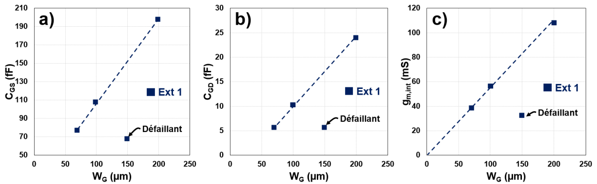
Figure 76 : a) Capacité grille-source, b) capacité grille-drain et c) transconductance intrinsèque en fonction de plusieurs développements de grille.
