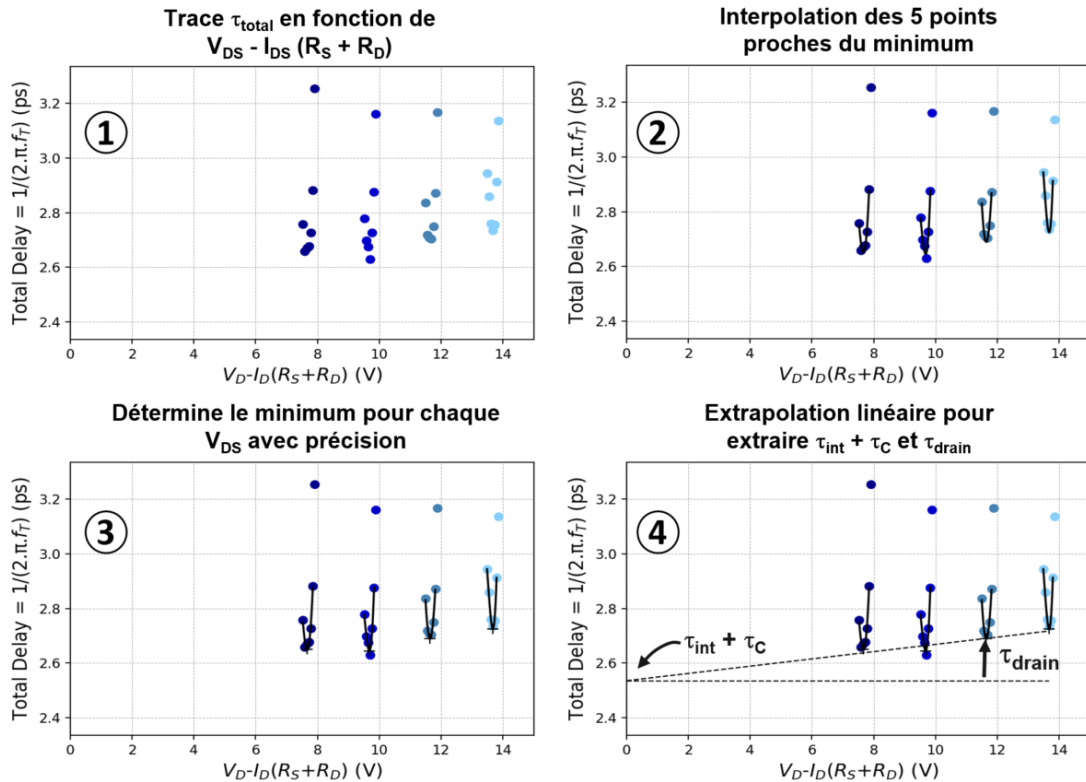
Figure 81 : Méthodologie de la détermination graphique de \tau_{int} + \tau_C et de \tau_{drain} .
