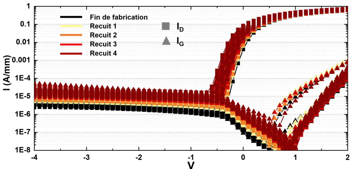
Figure 93 : Caractéristique de transfert I_D-V_G à V_{DS}=10 V d'un transistor ( W_G=2 \times 35 \mu m ; L_G=150 nm, L_{GS}=0,3 \mu m ; L_{GD}=1 \mu m) sur 21 sites mesurés entre chacun des recuits cumulés soit 105 courbes.
