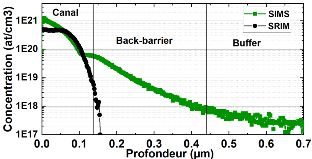
Figure 58 : Profil ToF-SIMS du silicium en fonction de la profondeur dans l'empilement épitaxial (N. Gautier).
