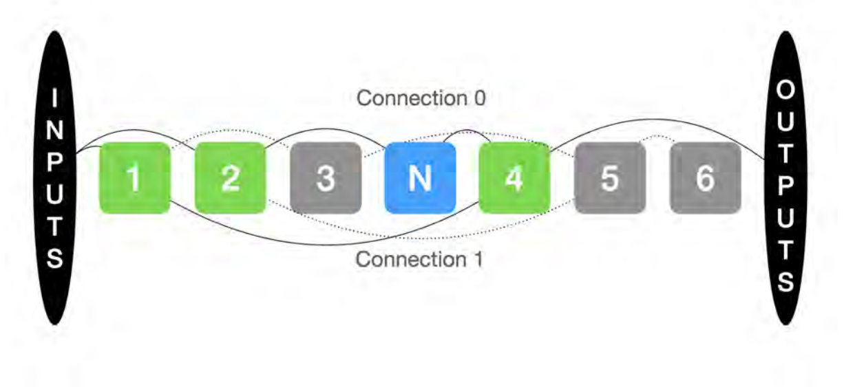
Figure 4.2: Un graphe avec un nœud N inséré à l'index 4
