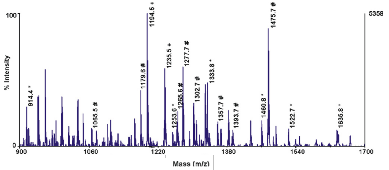
FIGURE 2.4 – Exemple de spectre MS1 obtenu expérimentalement. Spectre issu de [THIEDE et al. 2005]. Le spectre MS1 a été obtenu à partir d’un extrait cytosolique d’ Helicobacter pylori . L’analyse par empreinte peptidique (PMF) permet de détecter la présence de contaminants (#), de peptides issus de la protéine régulatrice HP0703 (*) et de peptides issus de la protéine HP0163 (+).
