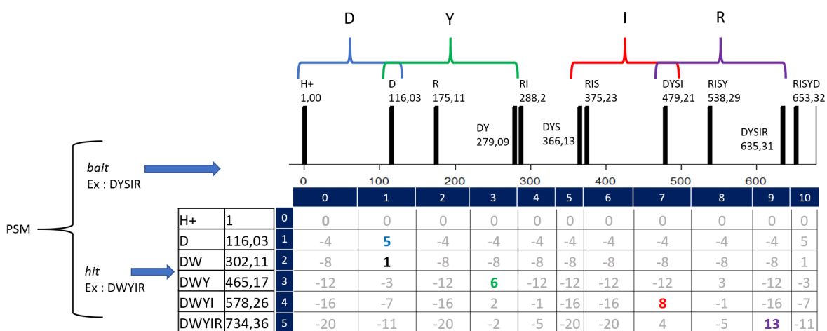
FIGURE 4.5 – Matrice D entièrement remplie. Le meilleur alignement a un score de 13 (en violet). Les masses indiquées sont en Da.
