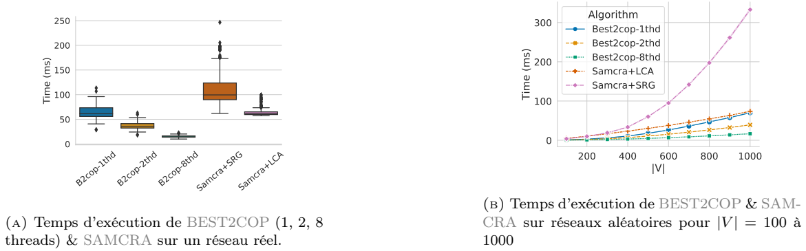
FIGURE 7.5: Temps d'exécution de BEST2COP and SAMCRA dans divers scénarios.
