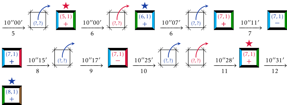
FIGURE F.8 – Résumé 3.1 : le cas de la bande \mathcal{B}_1 .
