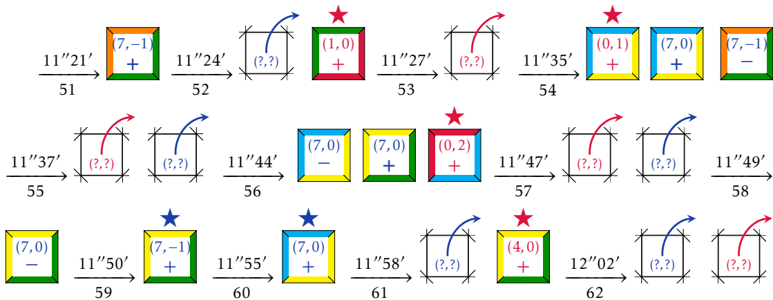
FIGURE H.6 – Résumé 2.2 : le cas du plan.
