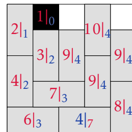
(d) Résumé correspondant à l'intervalle [0, 18[ dans la retranscription.
