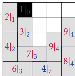
(c) Résumé correspondant à l'intervalle [0, 16[ dans la retranscription.
