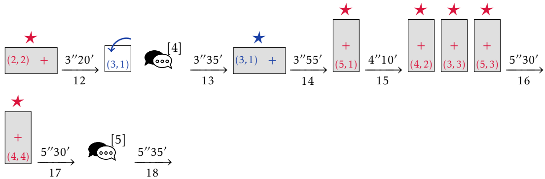
FIGURE V.6 – Fragment de retranscription correspondant à l'intervalle [0, 18[ de l'exemple V.7 (p. 66) avec le symbole « \star » permettant d'identifier les éléments qui apparaissent dans les résumés.
