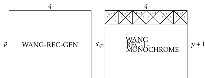
FIGURE VII.26 – \mathcal{NP} -dureté, réduction polynomiale pour un bord monochrome au nord : \text{WANG-REC-GEN} \leq_p \text{WANG-REC-1-MONOCHROME} .
