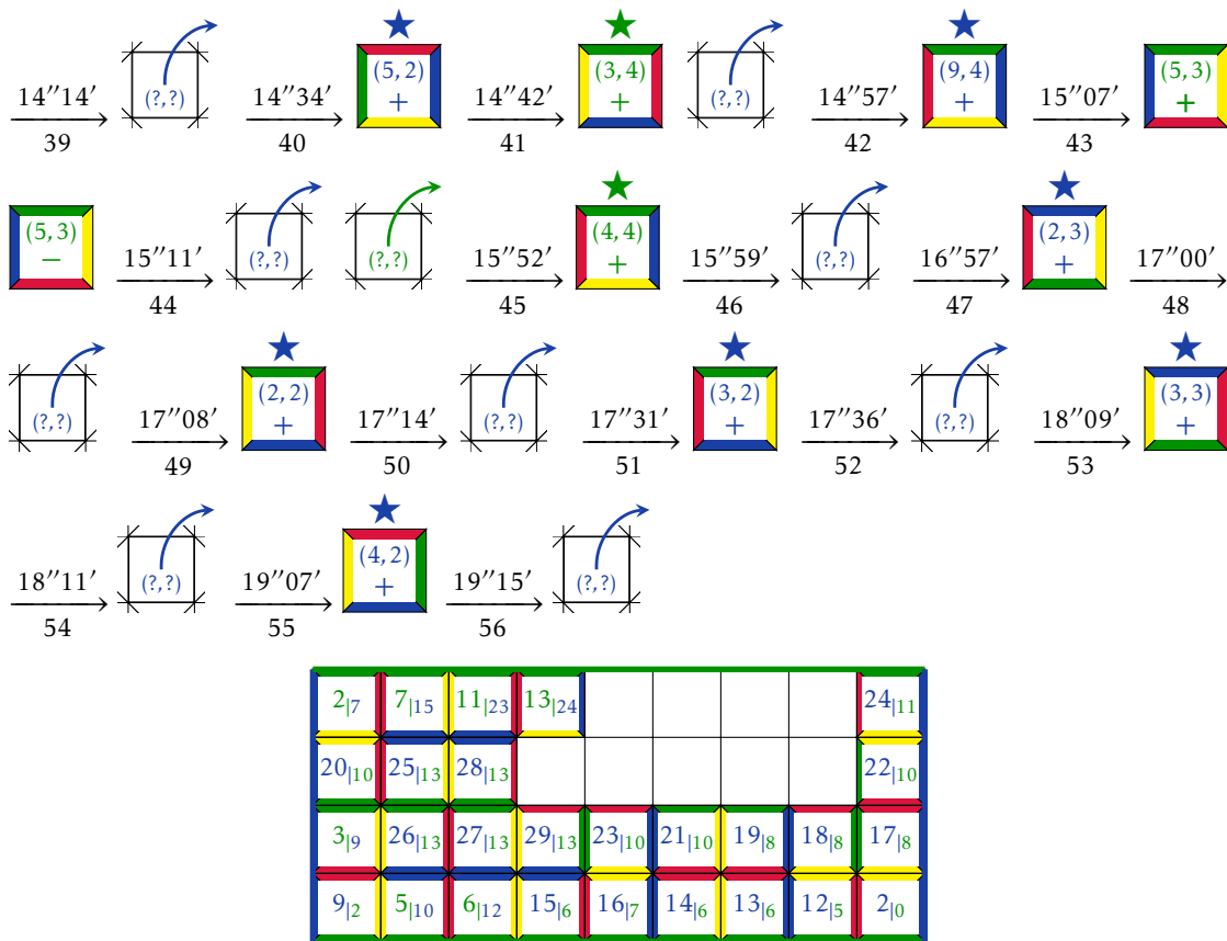
FIGURE E.4 – Résumé 1.3 : le cas du rectangle de type A.
