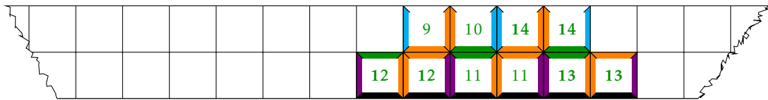
FIGURE G.3 – Résumé 1.2 : le cas de la bande \mathcal{B}_2 .
