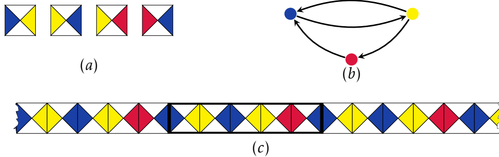
FIGURE VIII.47 – Ensemble de tuiles (a) pavant la bande \mathfrak{B}_1 avec toutes les tuiles (c) sans pour autant que son graphe associé (b) soit eulérien.
