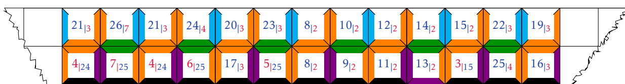
FIGURE G.9 – Résumé 2.4 : le cas de la bande \mathcal{B}_2 .
