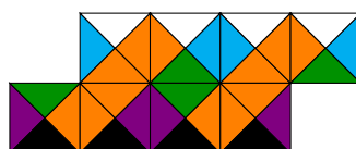
FIGURE XI.31 – Répétition du premier sous-mot permettant de générer deux motifs identiques.
