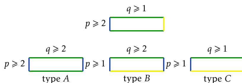
FIGURE VIII.3 – Les trois types de rectangle du problème WANG-RECTANGLE.
