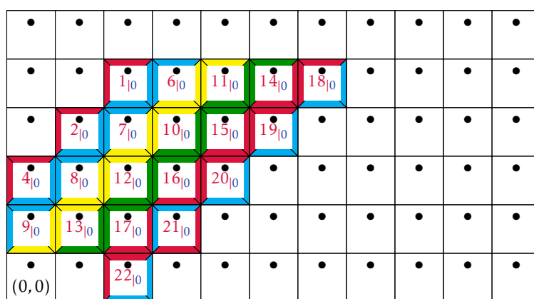
FIGURE H.12 – Résumé 3.1 : le cas du plan.
