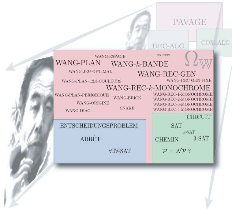
FIGURE VII.31 – Premier zoom sur l'espace-problème \Omega_W .
