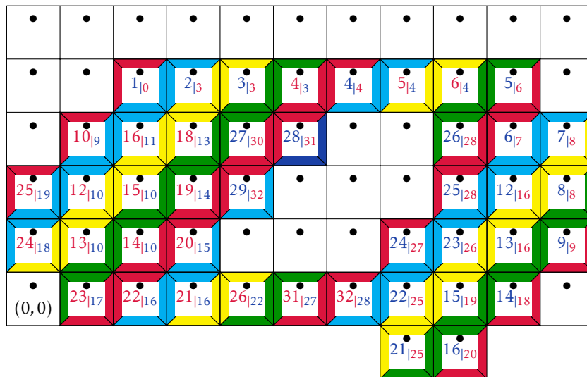
FIGURE H.7 – Résumé 2.3 : le cas du plan.
