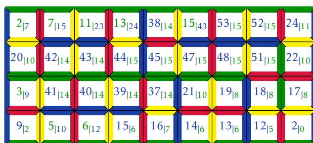
FIGURE XI.11 – Résumé 1.5 issu de la figure E.6, p. 339.
