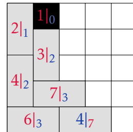
(b) Résumé correspondant à l'intervalle [0, 14[ dans la retranscription.
