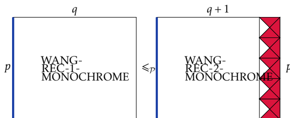
FIGURE VII.28 – \mathcal{NP} -dureté, réduction polynomiale pour deux bords monochromes opposés distincts : WANG-REC-1-MONOCHROME \leq_p WANG-REC-2-MONOCHROME.
