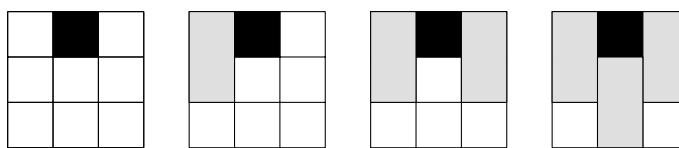
FIGURE V.2 – Preuve par forçage pour démontrer l'impossibilité de paver la grille 3 \times 3 avec le trou noir dans cette configuration.
