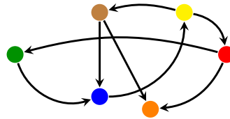
FIGURE VIII.45 – Exemple d'un ensemble de tuiles \mathcal{T} et son graphe G associé.
