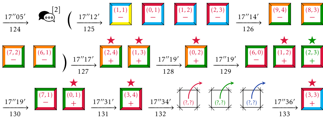
FIGURE H.9 – Résumé 2.5 : le cas du plan.
