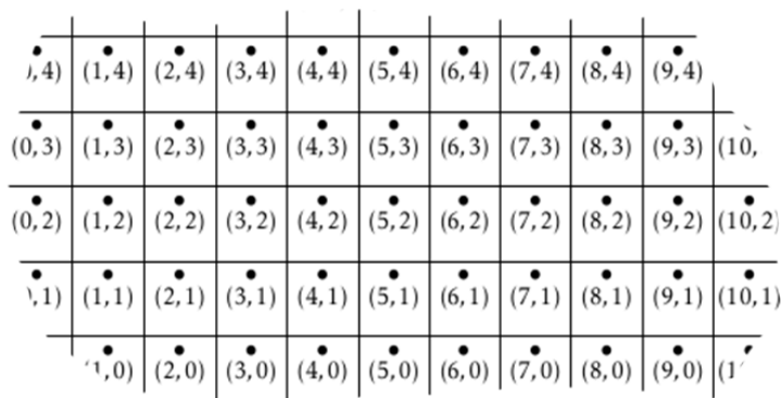
FIGURE H.1 – \mathcal{Z}_T concernant la situation du plan.
