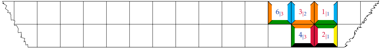
FIGURE G.10 – Résumé 3.1 : le cas de la bande \mathcal{B}_2 .
