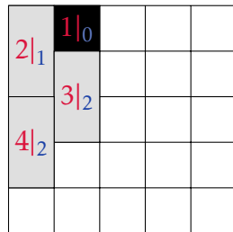
(a) Résumé correspondant à l'intervalle [0, 7[ dans la retranscription.
