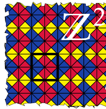
Pavage de plan \mathbb{Z}^2 avec quatre tuiles de \mathcal{T} .
