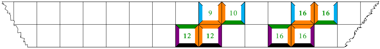
FIGURE G.5 – Résumé 1.4 : le cas de la bande \mathcal{B}_2 .
