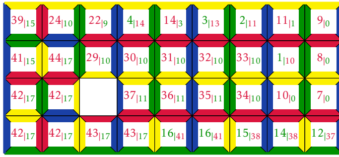
FIGURE E.11 – Résumé 2.5 : le cas du rectangle de type |B|.
