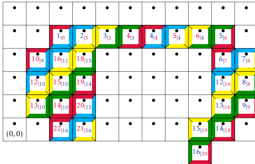
FIGURE H.6 – Résumé 2.2 : le cas du plan.
