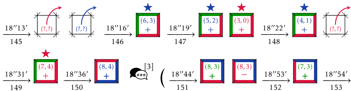
FIGURE H.10 – Résumé 2.6 : le cas du plan.
