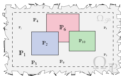
FIGURE IV.3 – Fragment de l'espace des problèmes \Omega_{\mathbb{P}} centré sur l'univers d'un problème \mathcal{P} autour de trois ensembles de problèmes \mathbb{P}_6 , \mathbb{P}_2 et \mathbb{P}_{10} dont les questions sont jugées proches de celle de \mathcal{P} .
