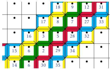
FIGURE XI.46 – Extrait du résumé 1.2 de la figure H.4, p. 370 montrant la répétition du motif 1 \times 4 pour paver le plan.
