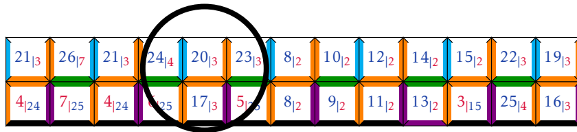
FIGURE XI.38 – Extrait du résumé 2.4 de la figure G.9 (p. 361) montrant que la stratégie FORÇAGE est mobilisée localement par s_4 .
