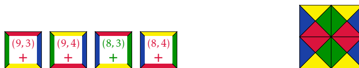
FIGURE XI.2 – Sous-mot périodique extrait de la retranscription générant un motif 2 \times 2 périodique.
