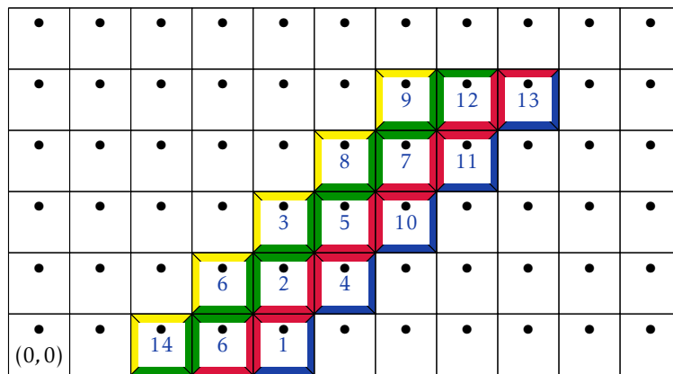
FIGURE H.3 – Résumé 1.1 : le cas du plan.
