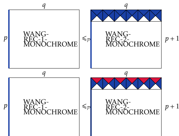
FIGURE VII.27 – \mathcal{NP} -dureté, réduction polynomiale pour deux bords monochromes adjacents distincts ou non : WANG-REC-1-MONOCHROME \leq_p WANG-REC-2-MONOCHROME.
