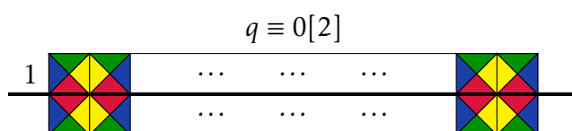
FIGURE VIII.9 – Existence d'un pavage pour le rectangle 2 \times q de type A avec q pair à partir de la réflexion d'un rectangle 1 \times q de type B .
