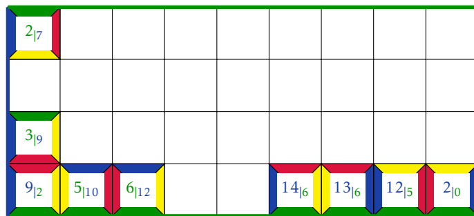
FIGURE E.2 – Résumé 1.1 : le cas du rectangle de type A.
