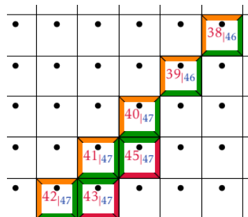
FIGURE XI.43 – Extrait du résumé 2.5 de la figure H.9 (p. 375) montrant la structuration « diagonale » d'une de ces \mathcal{T} -actions.
