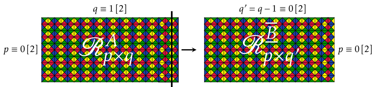
FIGURE VIII.27 – Construction de pavages valides pour les rectangles de types |B| et \overline{B} à partir d'un pavage de type A de taille p \times q avec p pair et q impair.
