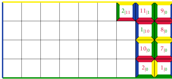
FIGURE E.7 – Résumé 2.1 : le cas du rectangle de type |B|.
