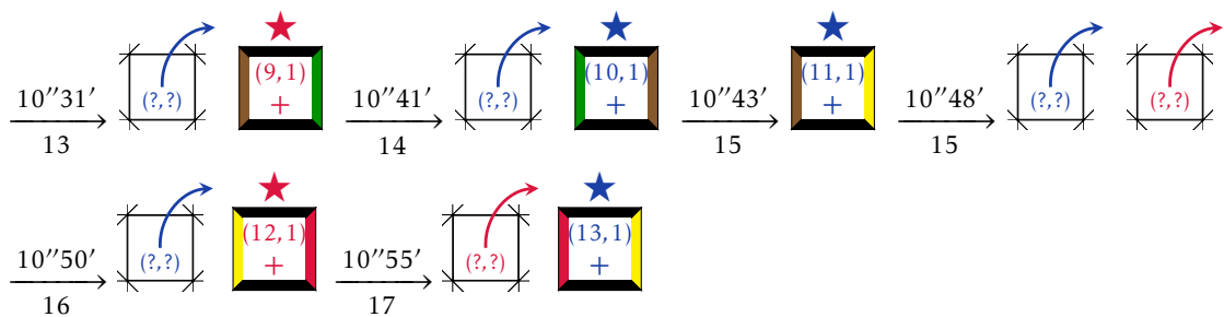
FIGURE F.9 – Résumé 3.2 : le cas de la bande \mathcal{B}_1 .
