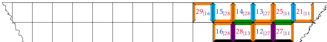
FIGURE G.12 – Résumé 3.3 : le cas de la bande \mathfrak{B}_2 .
