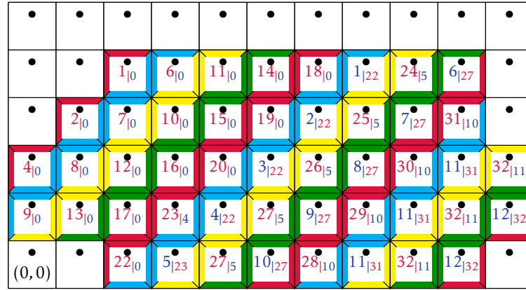
FIGURE H.13 – Résumé 3.2 : le cas du plan.
