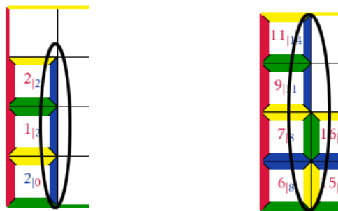
FIGURE XI.18 – Extrait des résumés 3.1 et 3.3 des figures E.13 et E.15 (p. 344 et 346).
