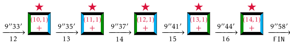
FIGURE F.3 – Résumé 1.2 : le cas de la bande \mathcal{B}_1 .
