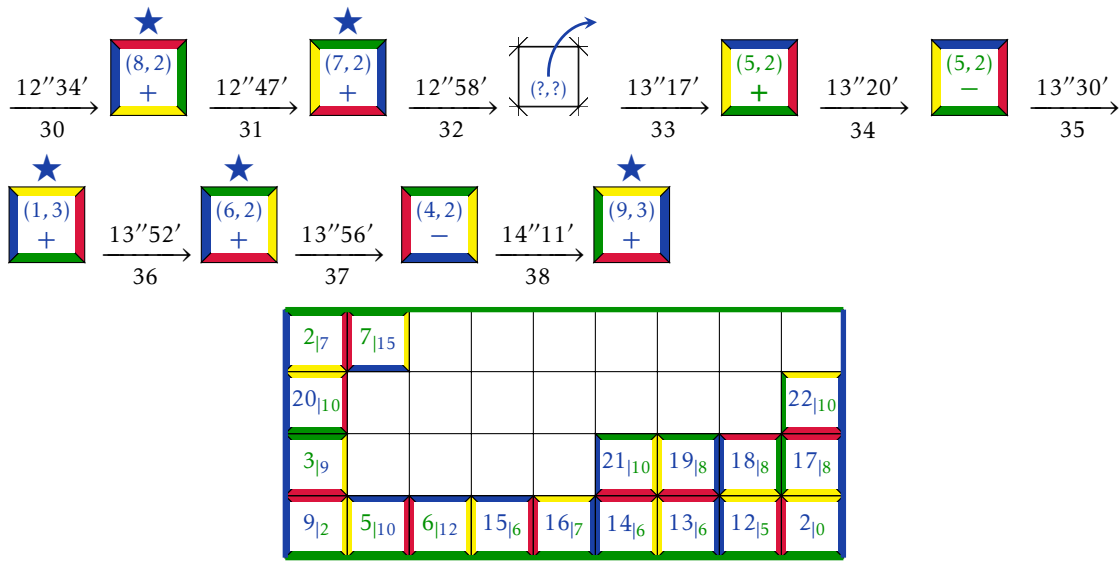
FIGURE E.3 – Résumé 1.2 : le cas du rectangle de type A.
