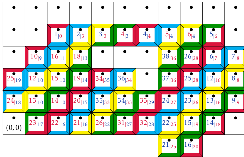
FIGURE H.8 – Résumé 2.4 : le cas du plan.
