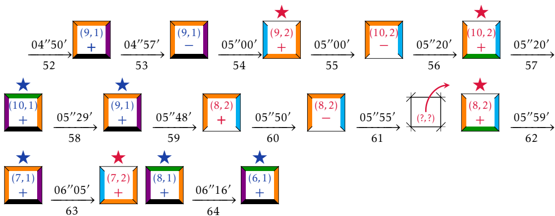
FIGURE G.12 – Résumé 3.3 : le cas de la bande \mathfrak{B}_2 .
