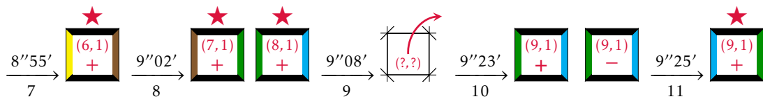
FIGURE F.2 – Résumé 1.1 : le cas de la bande \mathcal{B}_1 .
