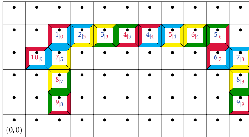
FIGURE H.5 – Résumé 2.1 : le cas du plan.
