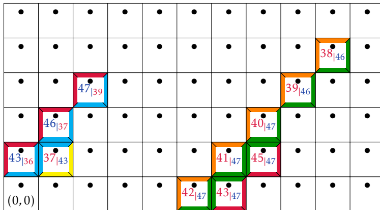
FIGURE H.9 – Résumé 2.5 : le cas du plan.
