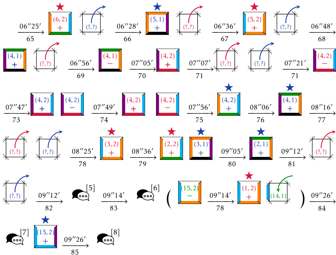
FIGURE G.13 – Résumé 3.4 : le cas de la bande \mathcal{B}_2 .
