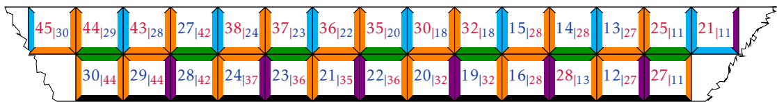
FIGURE G.14 – Résumé 3.5 : le cas de la bande \mathcal{B}_2 .
