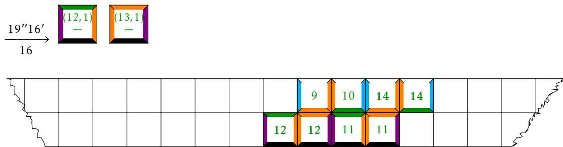
FIGURE G.4 – Résumé 1.3 : le cas de la bande \mathcal{B}_2 .
