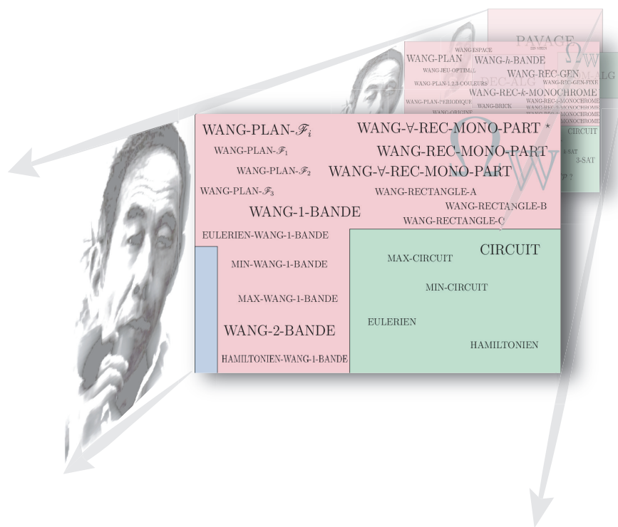
FIGURE VIII.61 – Deuxième zoom sur l'espace-problème \Omega_W .
