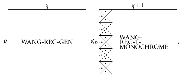
FIGURE VII.25 – \mathcal{NP} -dureté, réduction polynomiale pour un bord monochrome à l'ouest : \text{WANG-REC-GEN} \leq_p \text{WANG-REC-1-MONOCHROME} .
