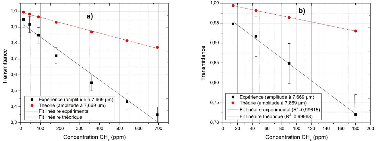
Figure V 2-17 : Courbe de calibration : transmission maximale due à l'absorption du CH 4 à 7,669 μm (expérience et théorie) (a) et zoom sur la partie linéaire (b).
