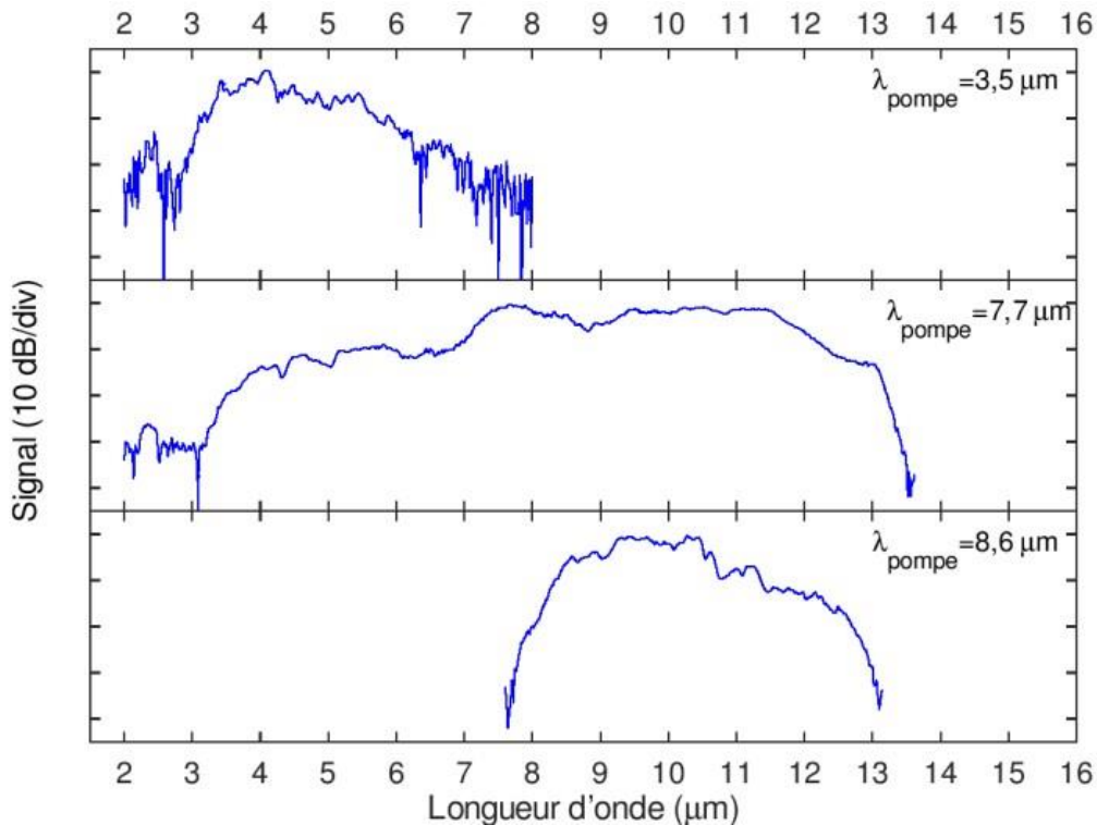
Figure IV 4-3 : Génération de supercontinuum dans une fibre à saut d'indice ( Ge_{20}Se_{60}Te_{20}/Ge_{20}Se_{70}Te_{10} ) de 4 cm et avec un cœur de 10 µm de diamètre [46].
