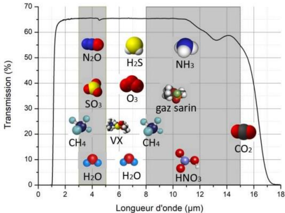
Figure IV 4-5 : Transmission d'un verre massif Ge_{20}Se_{60}Te_{20} d'épaisseur 5,88 mm et fenêtres de transparences atmosphériques (3-5 \mu\text{m} et 8-15 \mu\text{m} ). Représentation du domaine d'absorption de plusieurs molécules d'intérêts [22].
