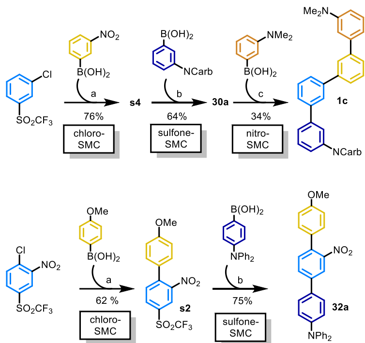
Schéma 1 : Couplage séquentiel pour la synthèse de ter- et quaterphényles
