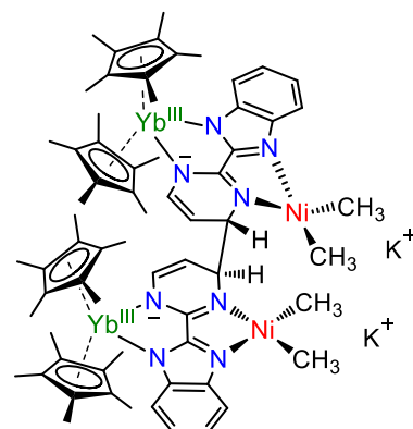
[Yb(bimpym)Ni] 2
