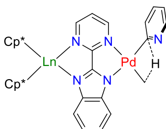
Ln-TS
