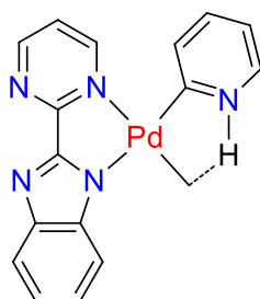
1.12-TS2
