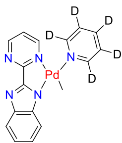
1.12-py-d 5
