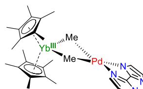
YbPd(impym)
