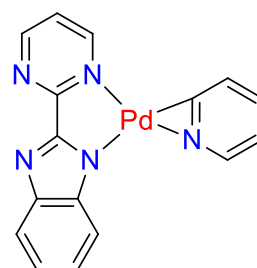
1.12-η 2
