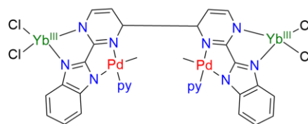
2.5Cl
