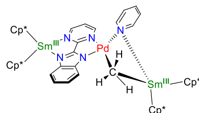
1.12-Sm 2
