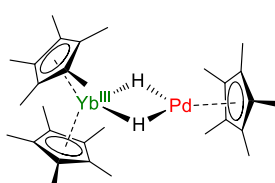
YbH 2 Pd
