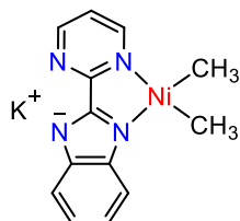
K(bimpym)NiMe 2
