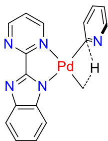
1.12-TS
