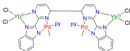
2.4Cl
