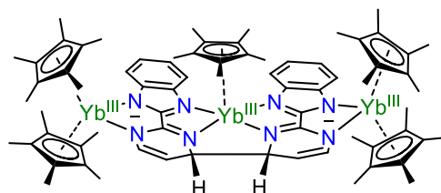
Yb 3 (bimpym) 2
