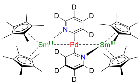
2.7-pyr-d 4
