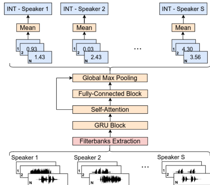
Figure 3 : Vue d'ensemble du système Word-RNN, utilisé pour prédire l'intelligibilité au niveau des mots. INT représente le score d'intelligibilité. N correspond au nombre de pseudo-mots utilisés pour le score.
