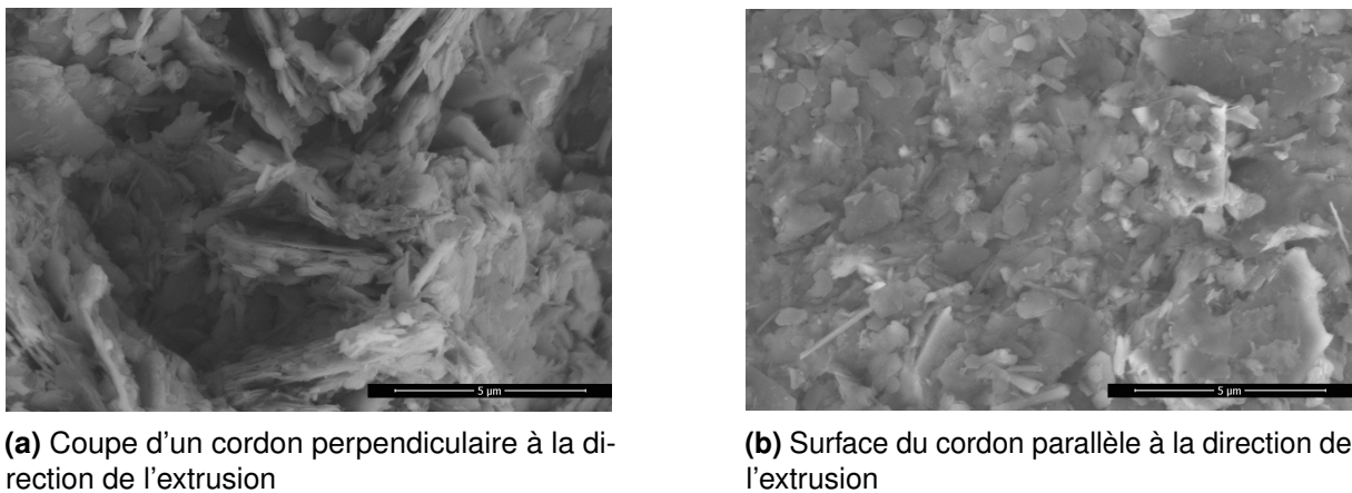
Figure 4.19: Images MEB d'un cordon de pâte de porcelaine EZPrint3D-E
