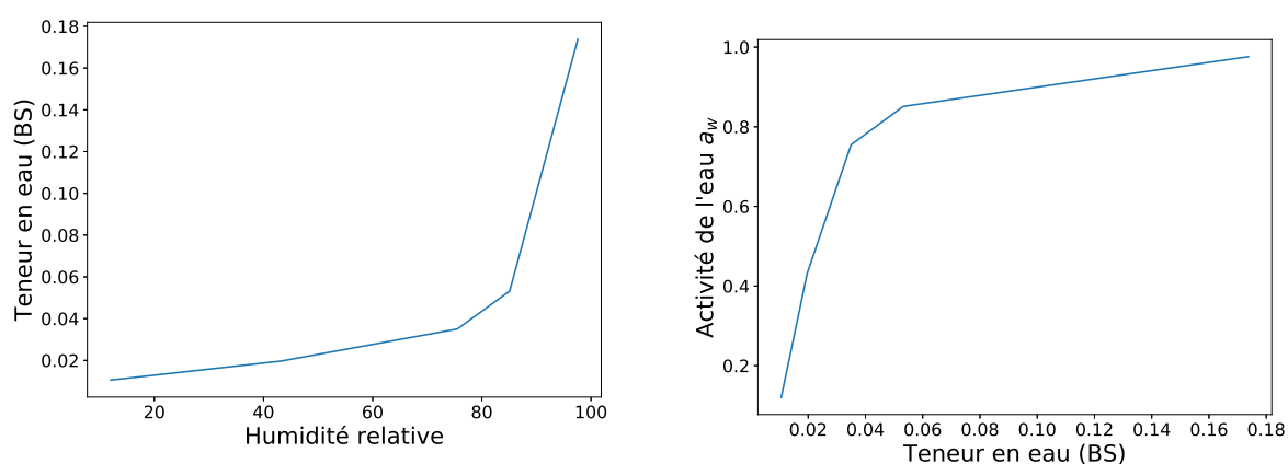
(a) Teneur en eau d'équilibre de l'échantillon en fonction de l'humidité relative de l'atmosphère de séchage. (b) Isotherme de désorption équivalent à la teneur en eau en fonction de l'activité de l'eau à 20°C.
