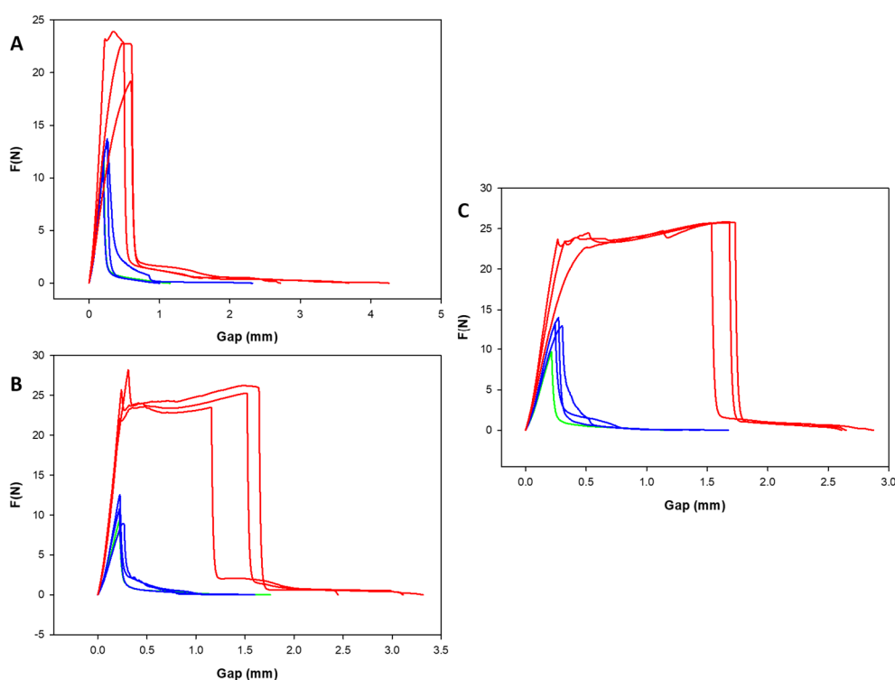
Figure III.8. Courbes de probe-tack (3h, 25°C, 100 \mu m/s ) des hydrogels 10% p/v gélatine + 10 mM catéchol avec NaIO_4 ( rouge ), 10% p/v gélatine + 10 mM pyrogallol avec NaIO_4 ( bleu ) et 10% p/v gélatine avec NaIO_4 ( vert ). Avec une concentration en NaIO_4 variable ; A ) 10 mM, B ) 20 mM et C ) 30 mM.
