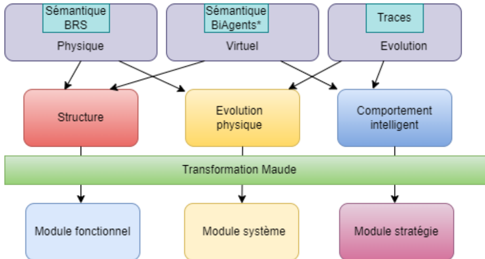
FIGURE 6.3 – Principe de transformation des spécification BiAgents* dans Maude strategy
